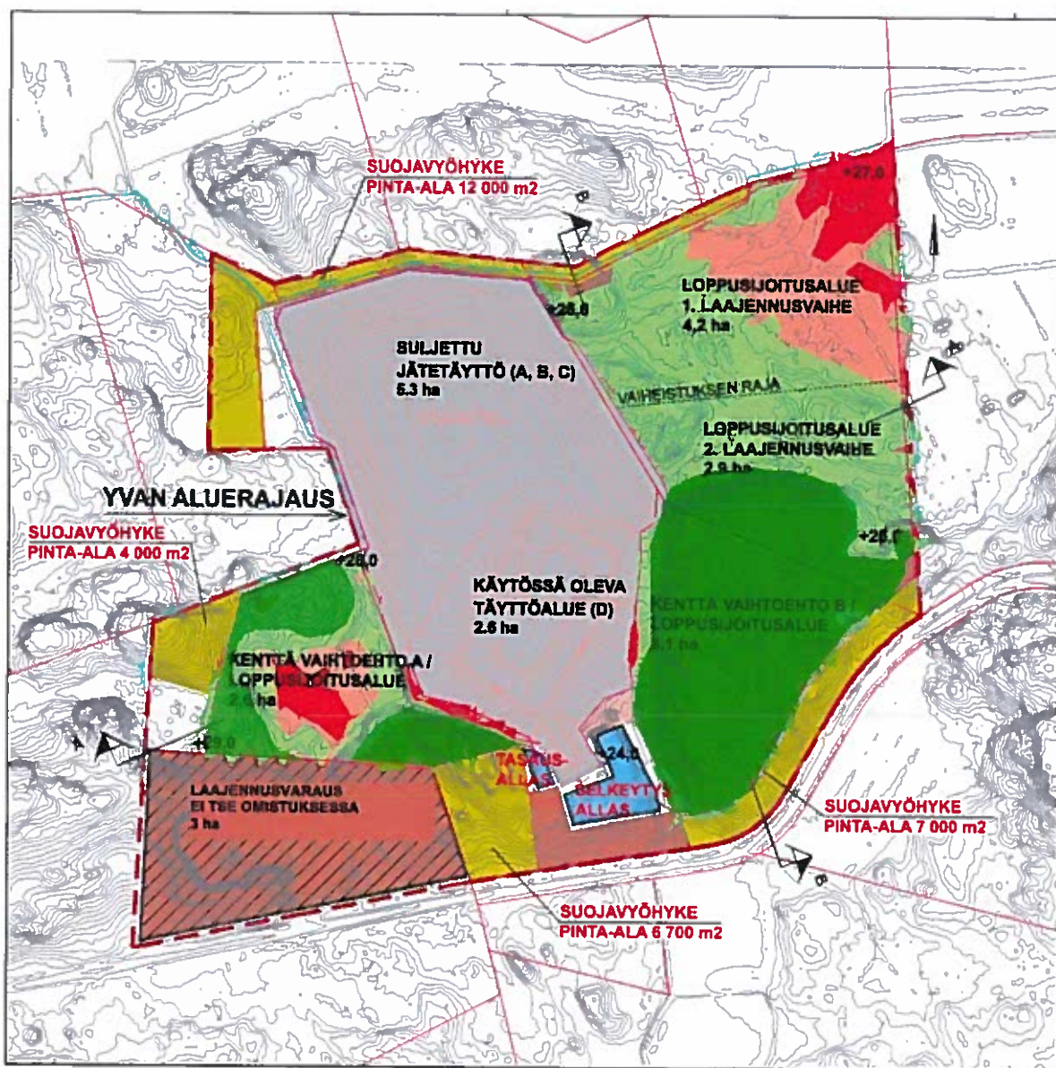
Kuva 3-8 Kuvassa on alustavasti esitetty vaihtoehdossa VE1b vihreällä kaivettavat/louhittavat ja punaisella värillä täytettävät alueet. Arvioidut louhittavat alueet on esitetty tumman vihreällä värityksellä. Louhittavien alueiden lopullinen määrä riippuu rakennussuunnitteluvaiheen tasauksesta.
