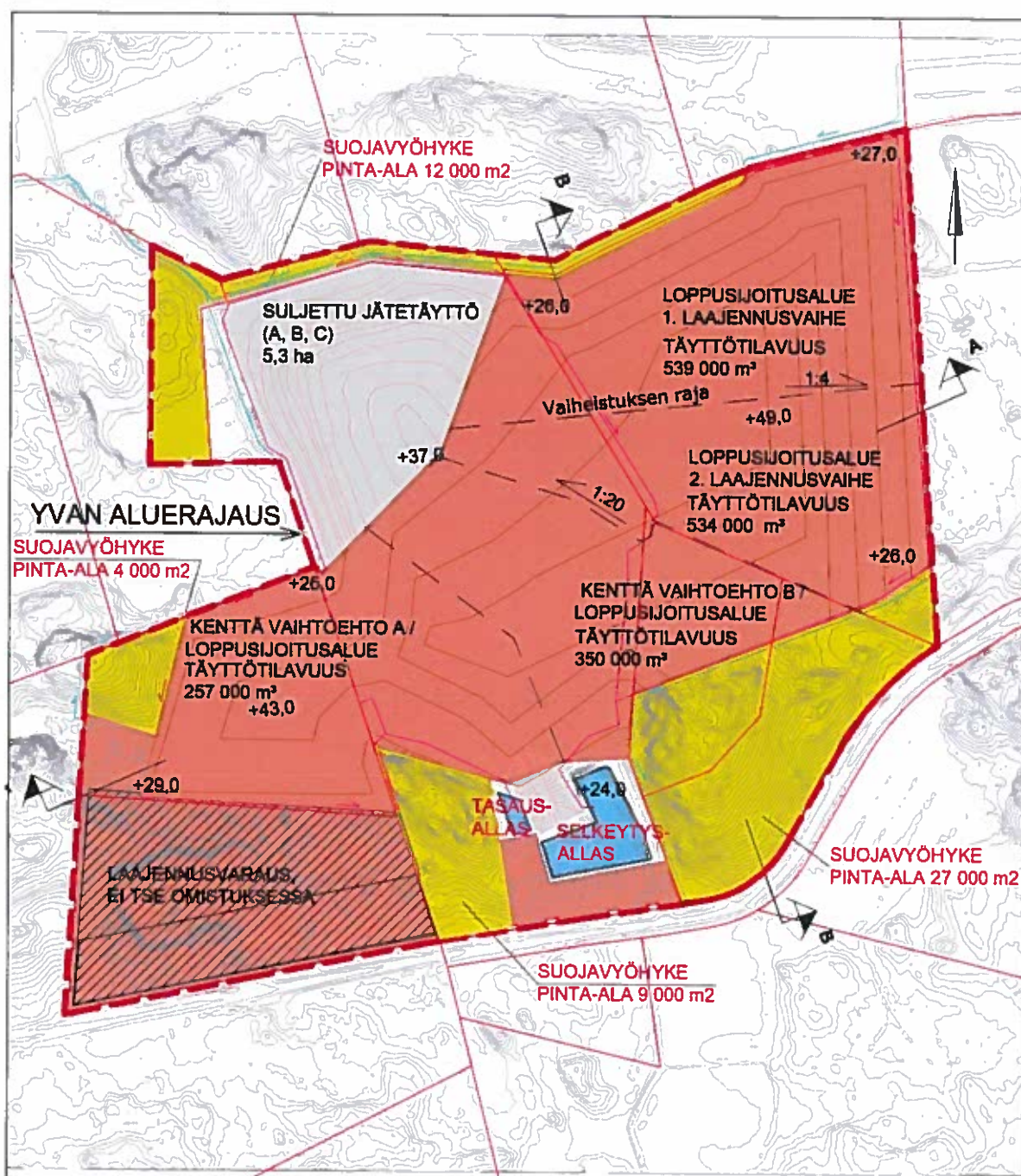
Kuva 3-5 Käsittelyalueen loppusijoitusalueet VE1a viimeisen vaiheen mukaisessa tilanteessa. Loppusijoitusalueiden laajennusvaiheet nojaavat vanhaan jätetäyttöön.
