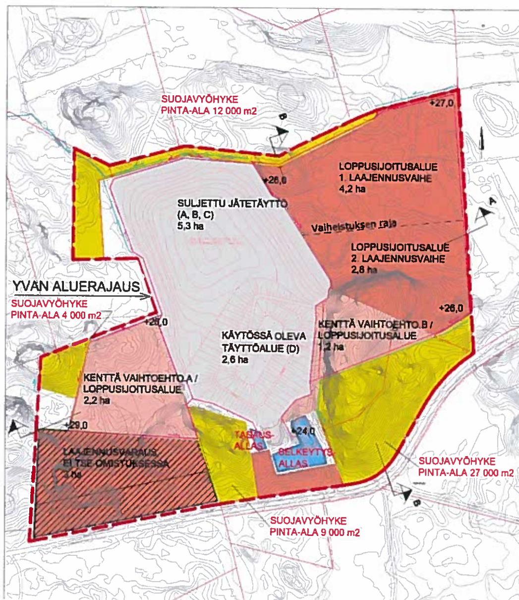
Kuva 3-4. Käsittelyalueen vaihtoehtoon VE1a mukainen alue. Laajennusalueiden pinta-alassa ei ole mukana vanhaan jätetäyttöön nojaavaa osuutta.
