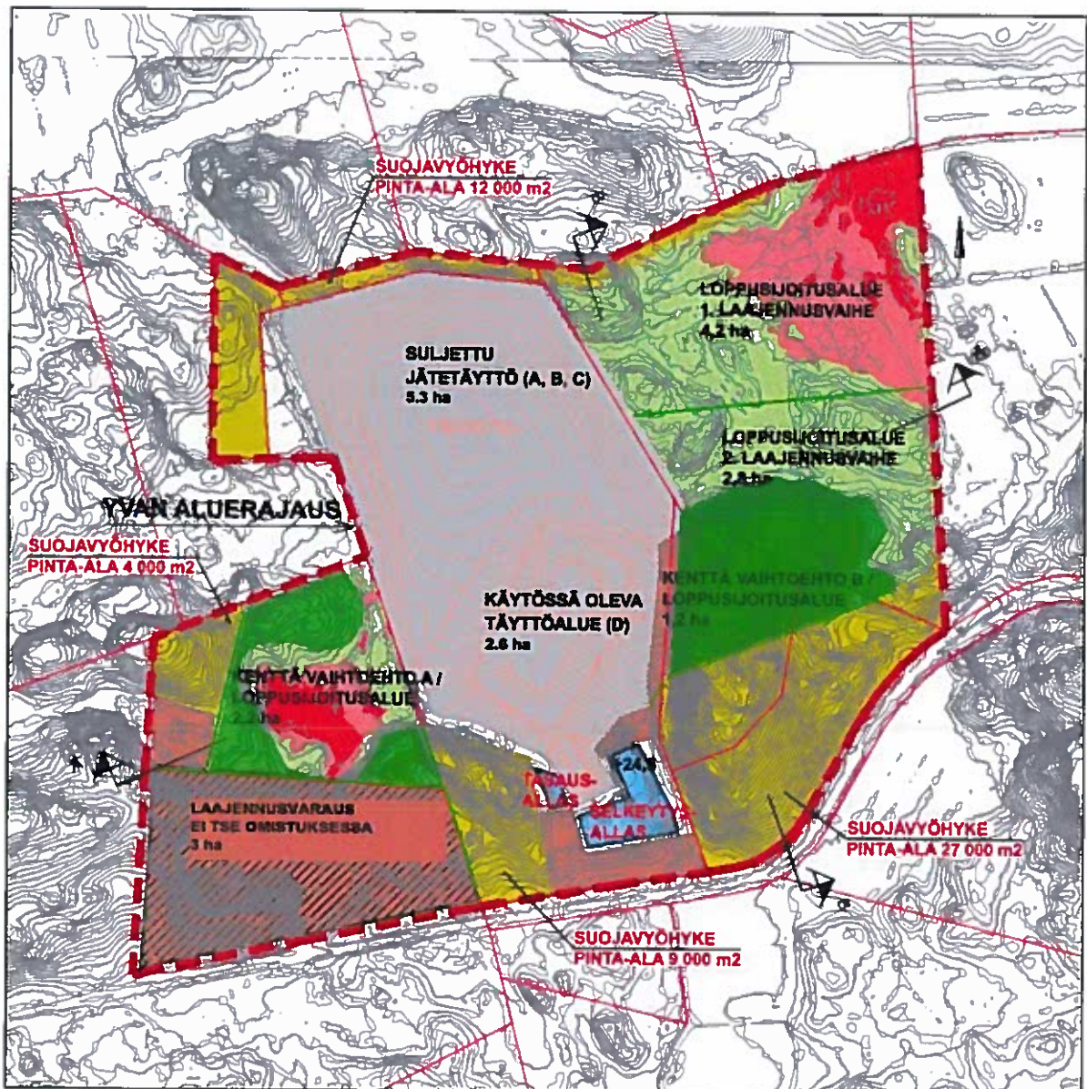
Kuva 3-7 Kuvassa on alustavasti esitetty vaihtoehdossa VE1a vihreällä kaivettavat/louhittavat ja punaisella värillä täytettävät alueet. Arvioidut louhittavat alueet on esitetty tumman vihreällä värityksellä. Louhittavien alueiden lopullinen määrä riippuu rakennussuunnitteluvaiheen tasauksesta.
