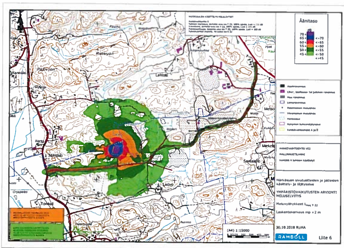
Kuva 11-6 Vaihtoehdon 1b melutasot hankealueen ympäristössä kentällä A tehtävän tuhkien murskauksen aikana.
