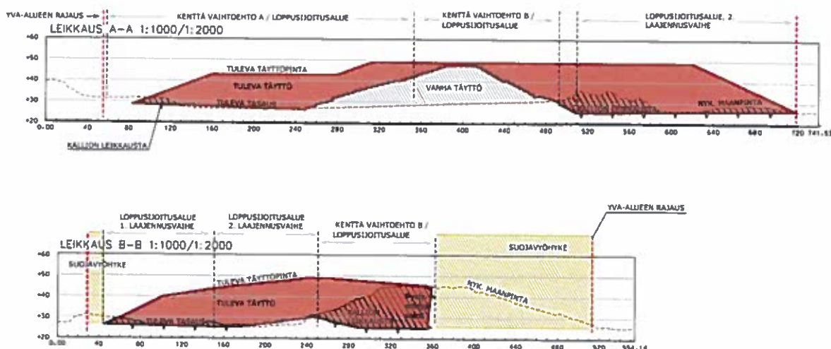
Kuva 3-6 Poikkileikkauksen viimeisen vaiheen mukaisesta tilanteesta.
