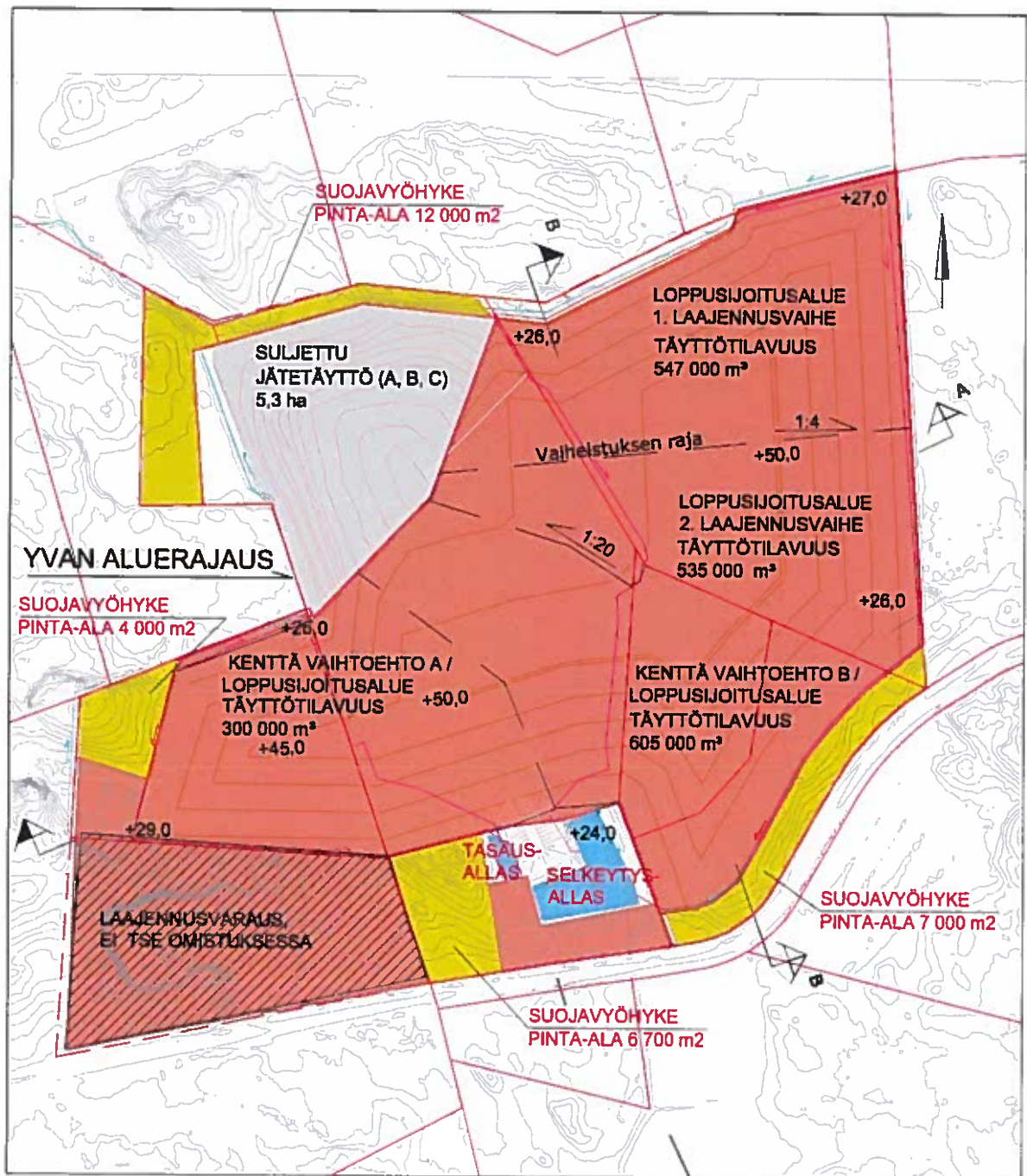
Kuva 3-8 Käsittelyalueen loppusijoitusalueet VE1b viimeisen vaiheen mukaisessa tilanteessa. Loppusijoitusalueiden laajennusvaiheet nojaavat vanhaan jätetäyttöön.
