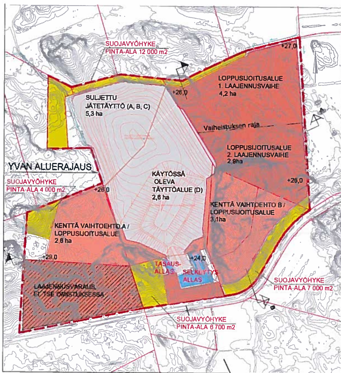
Kuva 3-7 Käsittealueen vaihtoehdot VE1b mukainen alue.
