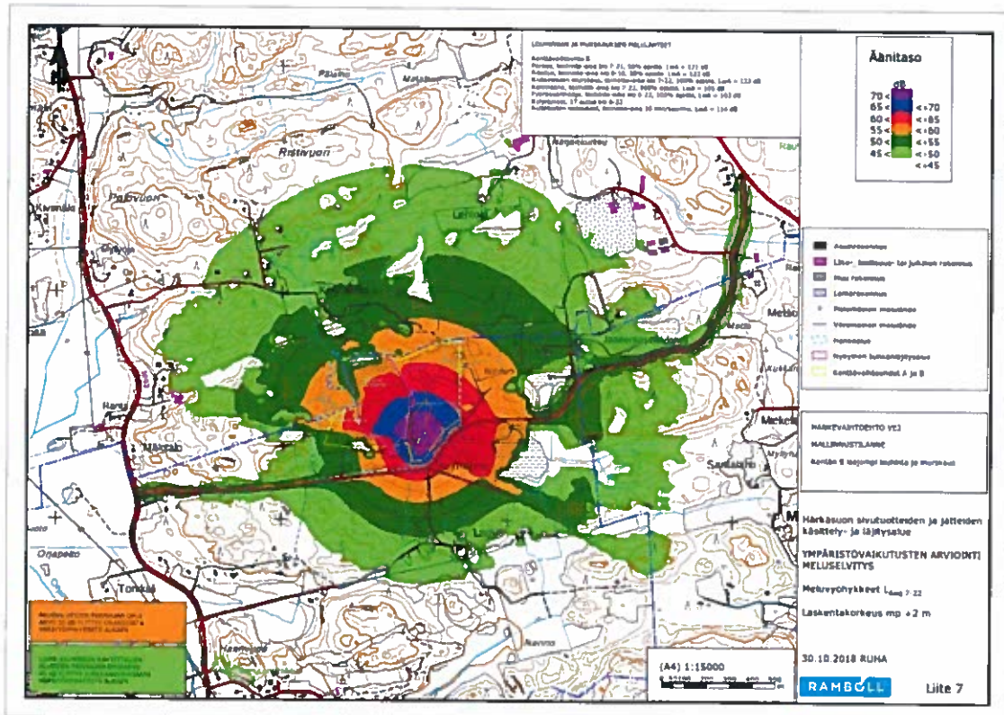
Kuva 11-7 Vaihtoehdon 1b melutasot hankealueen ympäristössä kenttävaihtoehto B louhinnan aikana.
