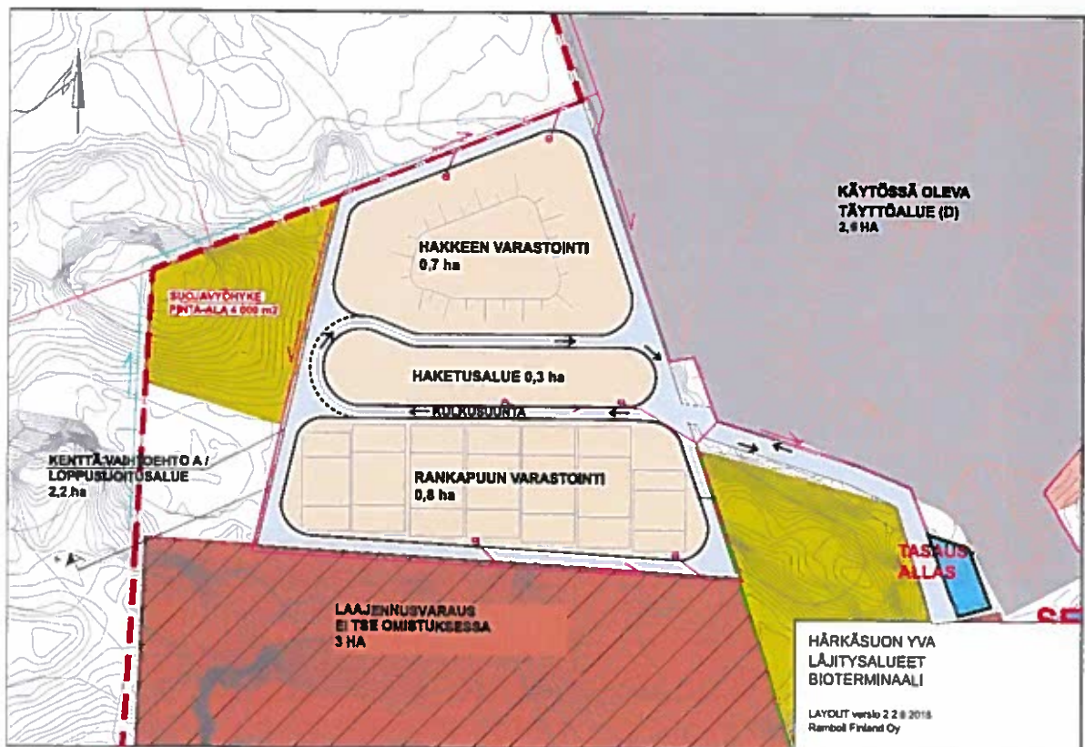
Kuva 3-10 Biotermiinalin sijoittuminen hankealueella
