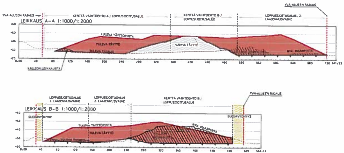
Kuva 3-9 Poikkileikkauksen viimeisen vaiheen mukaisesta tilanteesta vaihtoehdossa VE1b.
