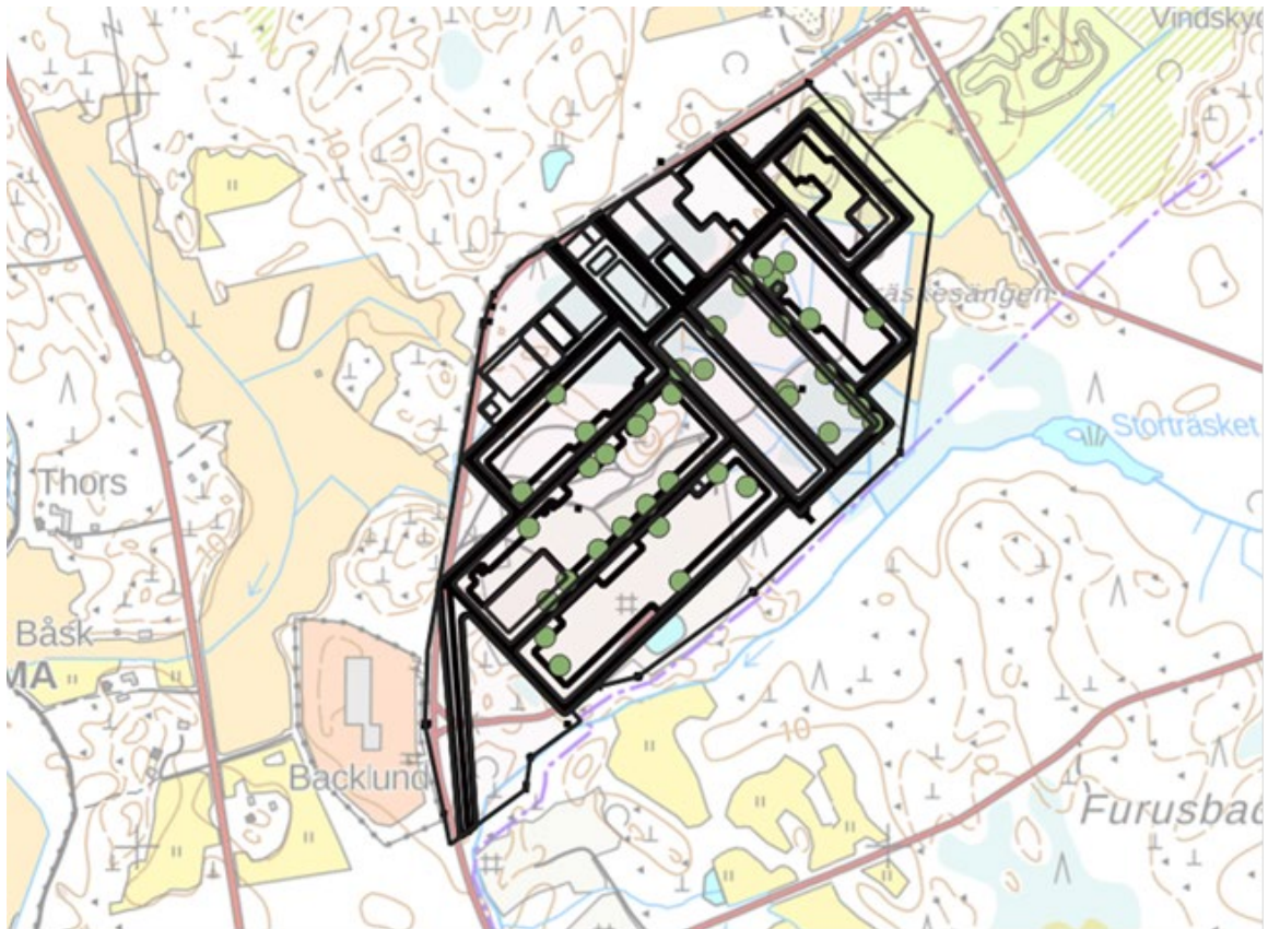
Kuva 3-7. Laitoksen päästöasteiden (savupiiput) sijainnit vaihtoehdossa VE1b.
