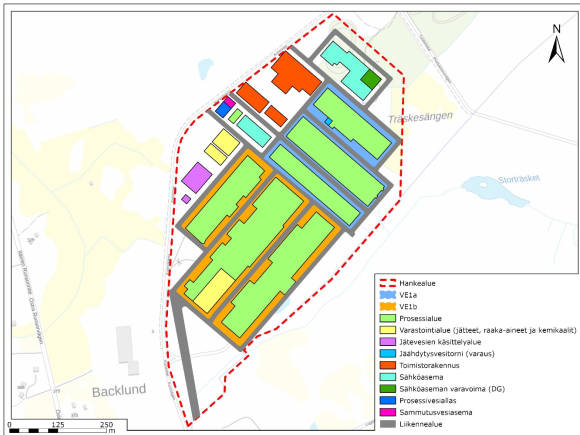
Kuva 3-3. Toimintojen sijoittuminen hankealueelle. Vaihtoehdossa VE1b kaikki rakennukset ovat valmiina.
