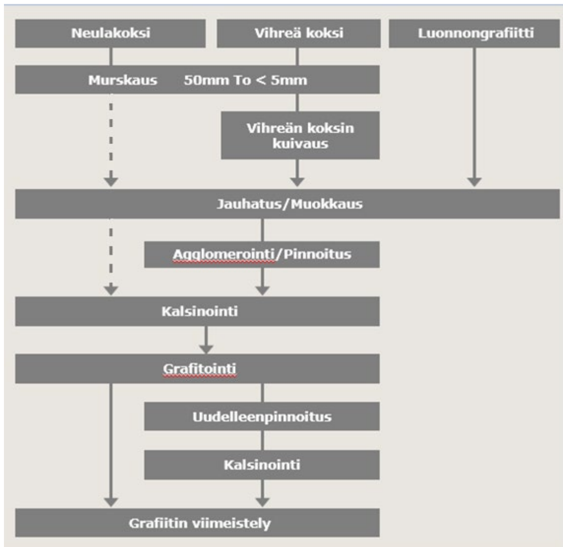
Kuva 3-4. Grafiittipohjaisen anodimateriaalin tuotantoprosessin kuvaus. Katkoviivalla merkityt reitit ovat vaihtoehtoisia eivätkä kaikki lopputuotteet käy kaikkia prosessivaiheita läpi.
