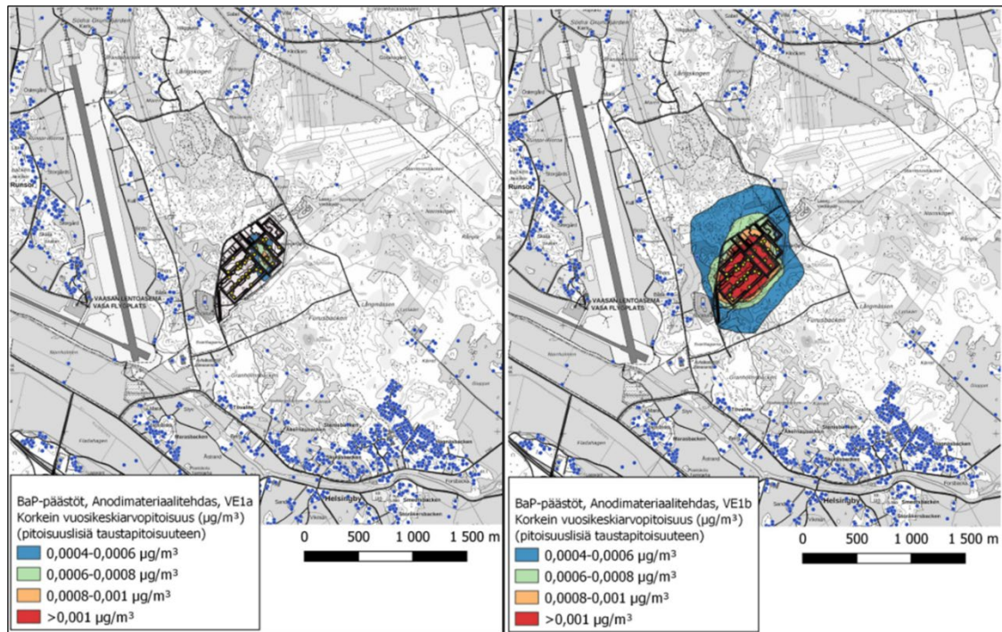
Kuva 9-5. Bentso[a]pyreenin (BaP) mallinnetut vuosikeskiarvopitoisuudet ( \mu\text{g}/\text{m}^3 ) vaihtoehdoissa VE1a ja VE1b. Suurin pitoisuus on VE1a:ssa 0,97 ng/m 3 eli 0,00097 \mu\text{g}/\text{m}^3 ja VE1b:ssä 2,9 ng/m 3 eli 0,0029 \mu\text{g}/\text{m}^3 . Esitetyt pitoisuudet ovat pitoisuuslisiä taustapitoisuuksiin.
