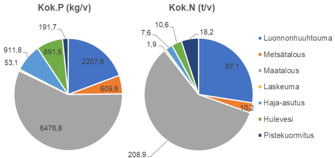
Kuva 17-4 Laihianjoen vesistöalueen (41) keskimääräinen ravinnekuormitus vuosina 2013–2020 (Suomen ympäristökeskus 2023f).
