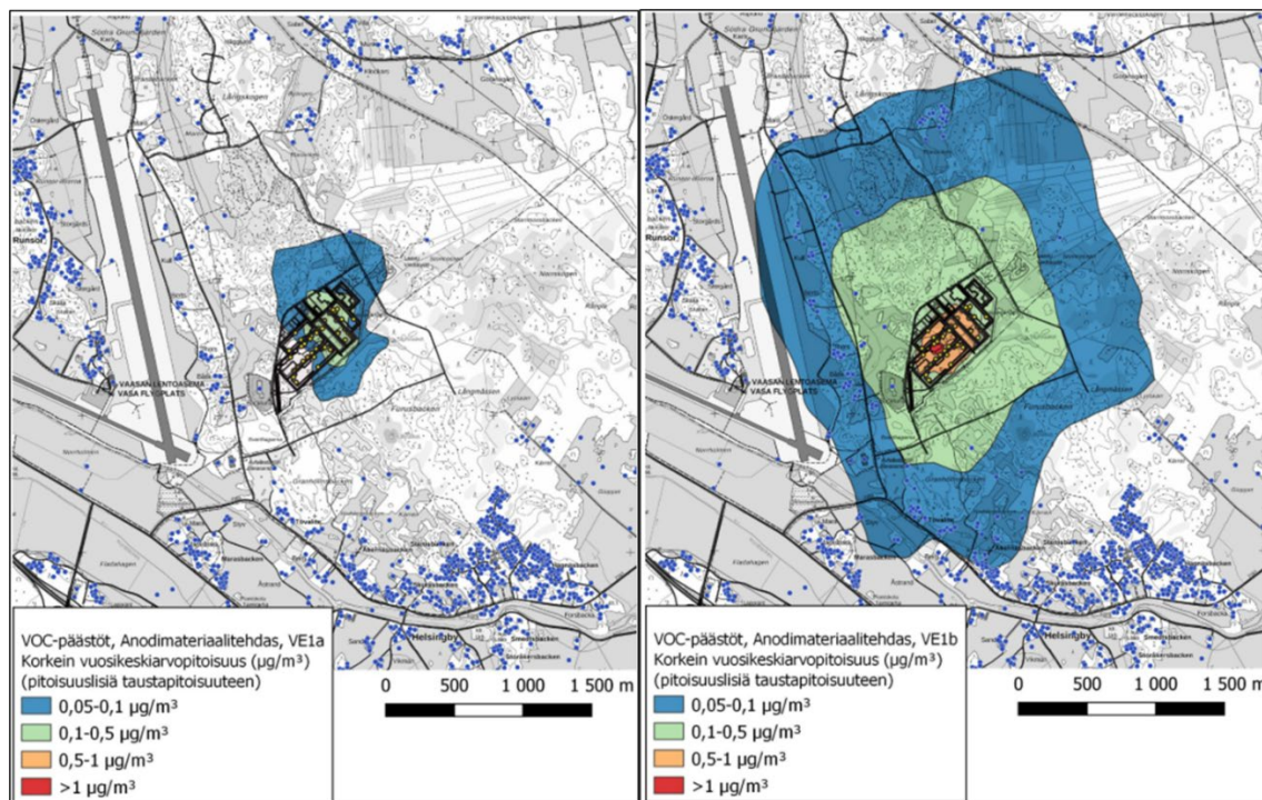
Kuva 9-6. Korkeimmat mallinnetut VOC-pitoisuudet vuosikeskiarvoina ( \mu\text{g}/\text{m}^3 ) vaihtoehtoisissa VE1a ja VE1b. Suurin pitoisuus on VE1a:ssa 0,4 \mu\text{g}/\text{m}^3 ja VE1b:ssä 1,2 \mu\text{g}/\text{m}^3 . Esitetyt pitoisuudet ovat pitoisuusliisiä taustapitoisuuksiin.
