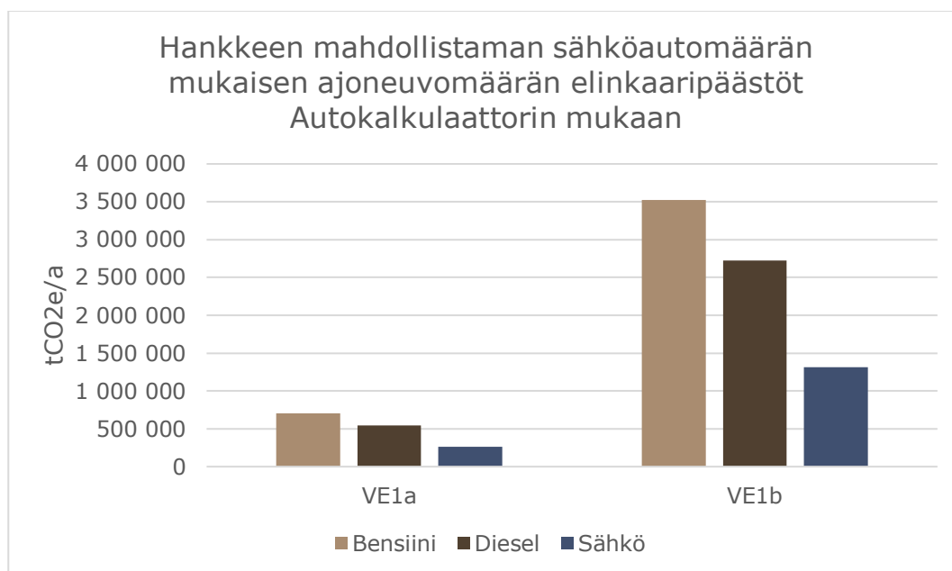
Kuva 10-9. Bensiini, diesel ja sähköauton elinkaaripäästöjen vertailu Suomen ilmastopaneelin Autokalkulaattorin mukaan kesikokoiselle autoille, kun ajokilometrejä on keskimäärin 14 000 km vuodessa ja auton keskimääräinen käyttöaika on 9 vuotta.
