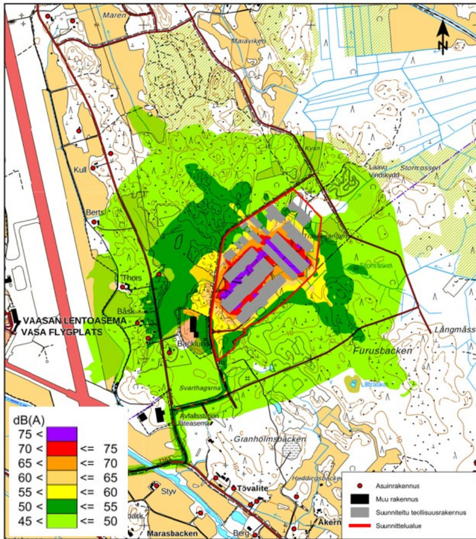
Kuva 11-3. Hankevaihtoehdon VE1b meluvyöhykkeet normaalin käyttötilanteen aikana vuorokauden keskiäänitasona (klo 00–24).
