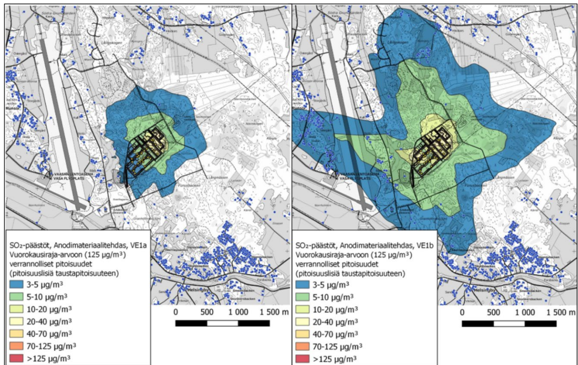
Kuva 9-3. Vuosiraja-arvoon (125 µg/m 3 ) verratut SO 2 -pitoisuudet (µg/m 3 ) vaihtoehtoisissa VE1a ja VE1b. Suurin pitoisuus on VE1a:ssa 12 µg/m 3 ja VE1b:ssä 38 µg/m 3 . Esitetyt pitoisuudet ovat pitoisuuslisä taustapitoisuuksiin.
