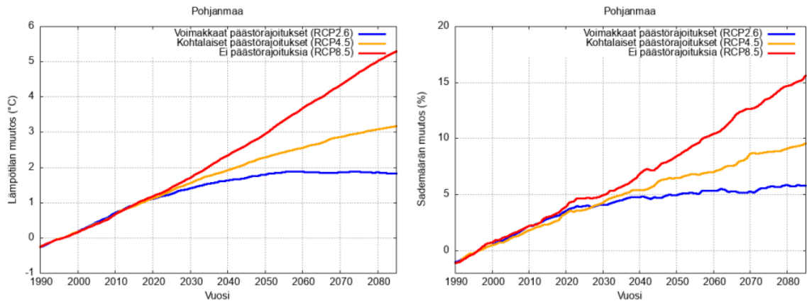
Kuva 10-4. Vuotuisen keskimääräisen lämpötilan ja sademäärän arvioidut muutokset Pohjanmaalla erilaisten kasvihuonekaasupäästöjen kehityskulkujen mukaan vuoteen 2100 asti. Muutokset ovat verrattuna jakson 1981–2010 ilmastoon (Gregow, H. et al. 2021).
