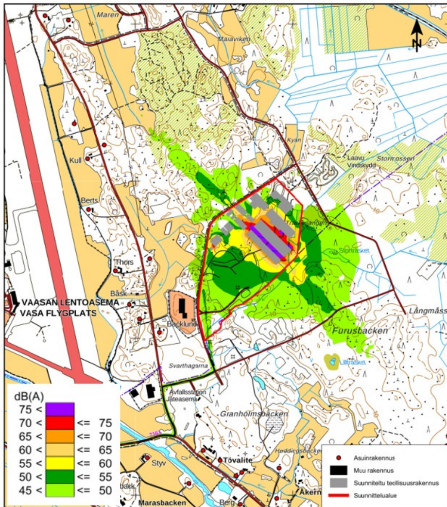
Kuva 11-2. Hankevaihtoehdon VE1a meluvyöhykkeet normaalin käyttötilanteen aikana vuorokauden keskiäänitasona (klo 00–24).
