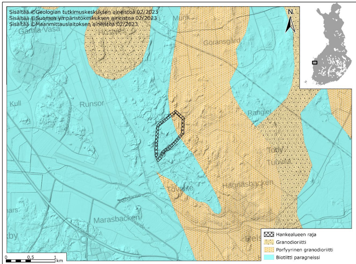
Kuva 16-1. Hankealueen lähiympäristön kallioperä. Hankealue on esitetty mustalla rajauksella. Lähde: Geologian tutkimuskeskus 2024a.
