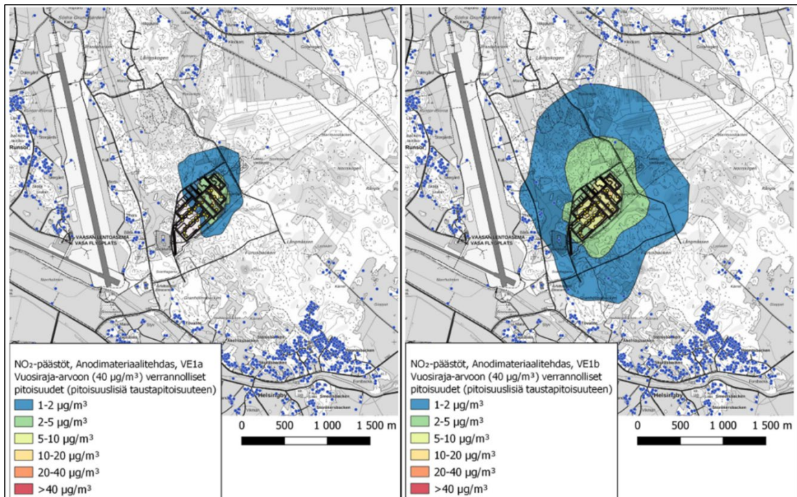
Kuva 9-4. Vuosisiraja-arvoon (40 µg/m 3 ) verratut NO 2 -pitoisuudet (µg/m 3 ) vaihtoehtoissa VE1a ja VE1b. Suurin pitoisuus on VE1a:ssa 9 µg/m 3 ja VE1b:ssä 11 µg/m 3 . Esitetyt pitoisuudet ovat pitoisuuslisä taustapitoisuuksiin.
