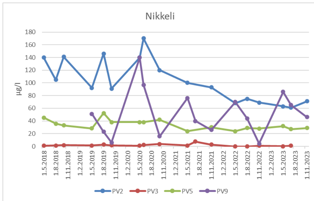
Kuva 16-10. Pohjaveden nikkelpitoisuuksia tuhkanlajitusalueen tarkkailupisteissä 2018–2023.
