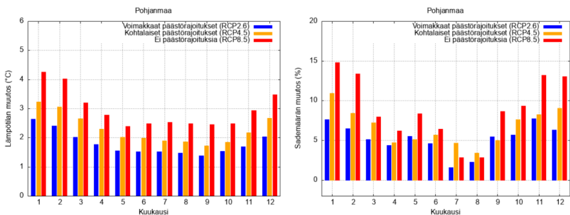
Kuva 10-5. Arvioidut lämpötilan ja sademäärän muutokset Pohjanmaalla kuukausittain v. 2050 mennessä. Muutokset ovat verrattuna jakson 1981–2010 ilmastoon. (Gregow, H. et al. 2021)
