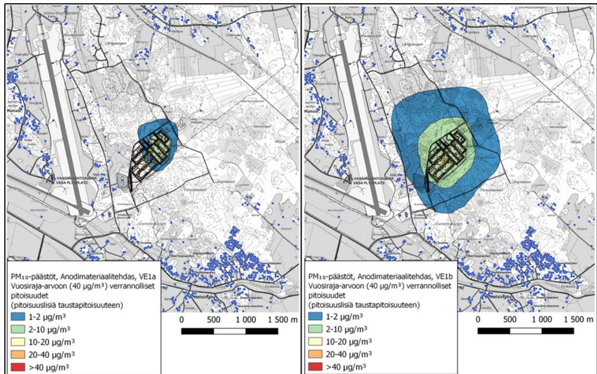
Kuva 9-2. Vuosisrāja-arvoon (40 µg/m³) verratut PM 10 -pitoisuudet (µg/m³) vaihtoehtoisissa VE1a ja VE1b. Suurin pitoisuus on VE1a:ssa 5 µg/m³ ja VE1b:ssä 11 µg/m³. Esitetyt pitoisuudet ovat pitoisuuslisiä taustapitoisuuksiin.
