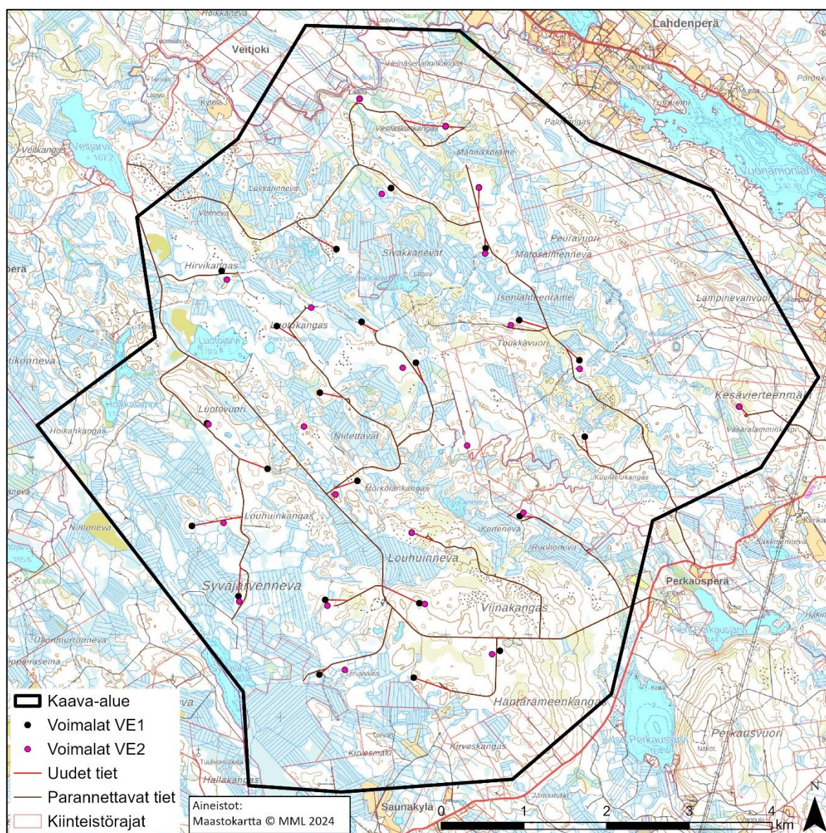
Kuva 3.1. Alustavat voimalasijoittelut VE 1 ja VE 2 sekä huoltotiestö vaihtoehdossa VE1. Voimaloiden väliset maakaapelit rakennetaan lähtökohtaisesti huoltotiestön yhteyteen.
