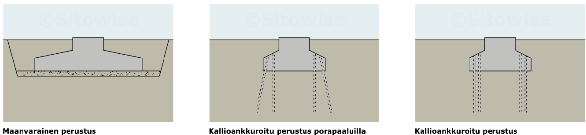
Kuva 4.2. Periaatekuvat tuulivoimalan vaihtoehtoisista perustamistavoista
