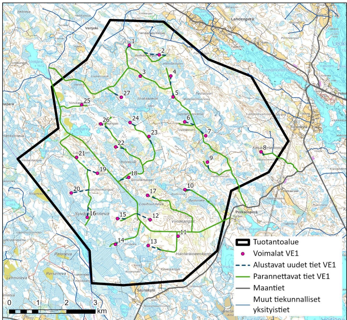
Kuva 4.3. Alustava suunnitelma VE1 parannettavista ja uusista teistä tuotantoalueella.
