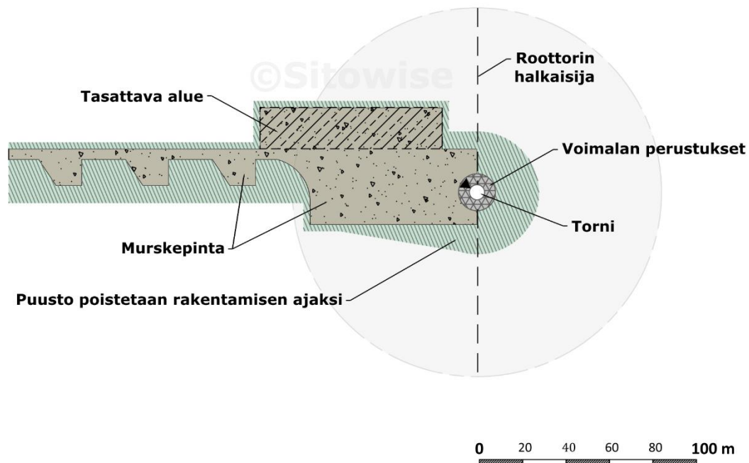
Kuva 4.6. Tuulivoimalan tyypillinen kokoamis- ja pystytysalue
