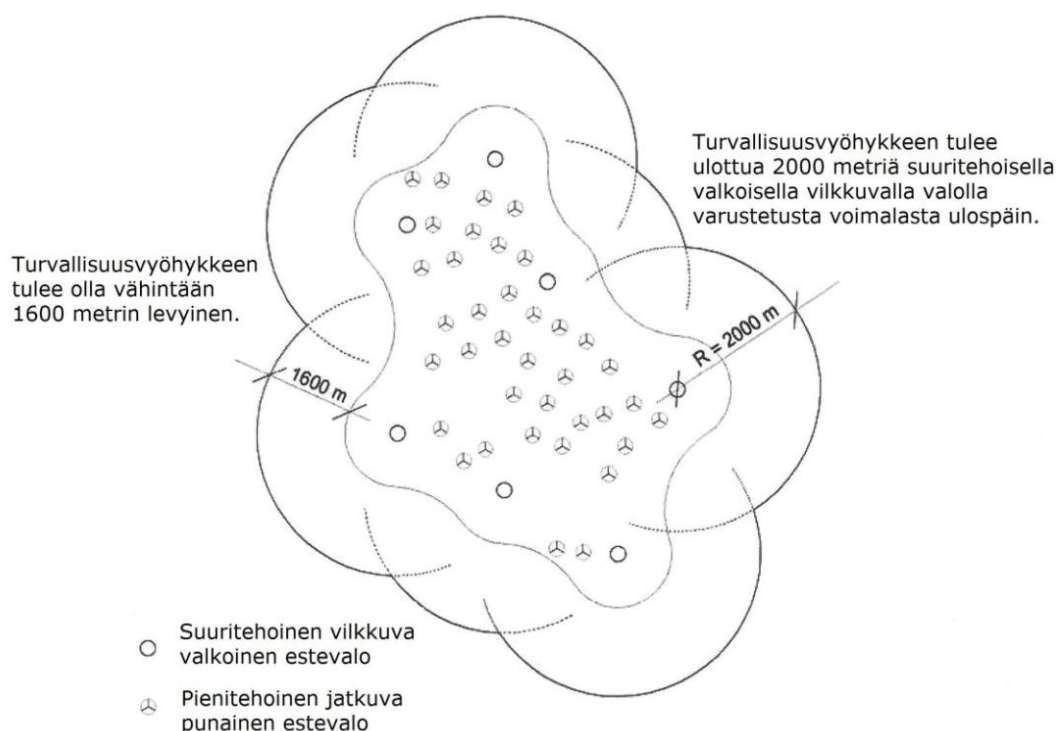
Kuva 4.7. Suuri- ja pienitehoisten lentoestevalojen sijoitteluesimerkki tuulivoimahankkeessa, jossa voimaloiden lapojen ylin pyyhkäisykorkeus on yli 150 metriä maanpinnasta (Liikenne- ja viestintävirasto Traficom 2020).
