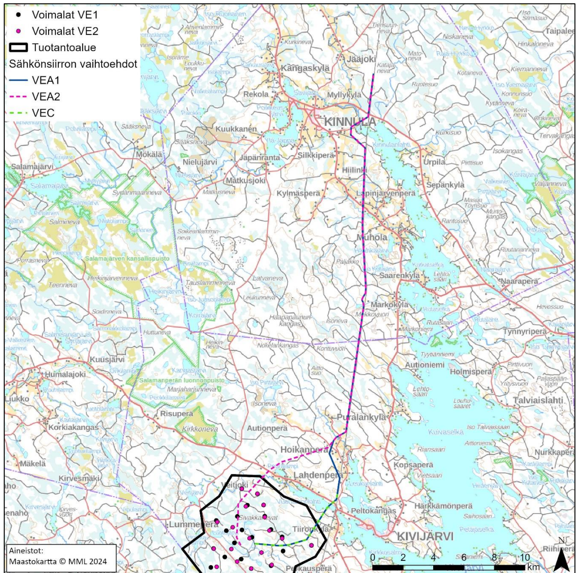
Kuva 1.2. Sähkönsiirtoyhteysvaihtoehdot VEA1 ja VEA2 pohjoiseen: 400 kV voimajohto tuotanto-alueelta olemassa olevan Metsälinjan tuntumaan linjan länsipuolelle sekä Metsälinjan tuntumaan kiertäen kauempaa asutuksen pohjoiseen päin seuraten Kinnulaan rakennettavalle sähköasemalle. Pituudet 36,3–36,6 km. Lisäksi sähkönsiirtoyhteys VEC: 110 kV voimajohto tuotantoalueelta suoraan Elenian Kivijärven sähköasemalle. Pituus 7,4 km.
