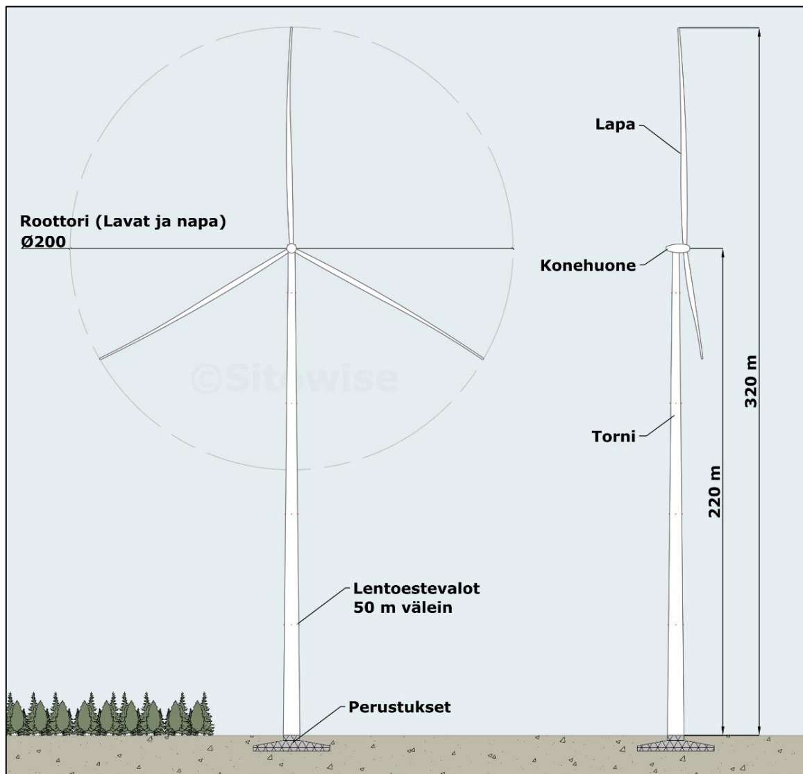
Kuva 4.1. Periaatekuva tuulivoimalan rakenteesta ja koosta.
