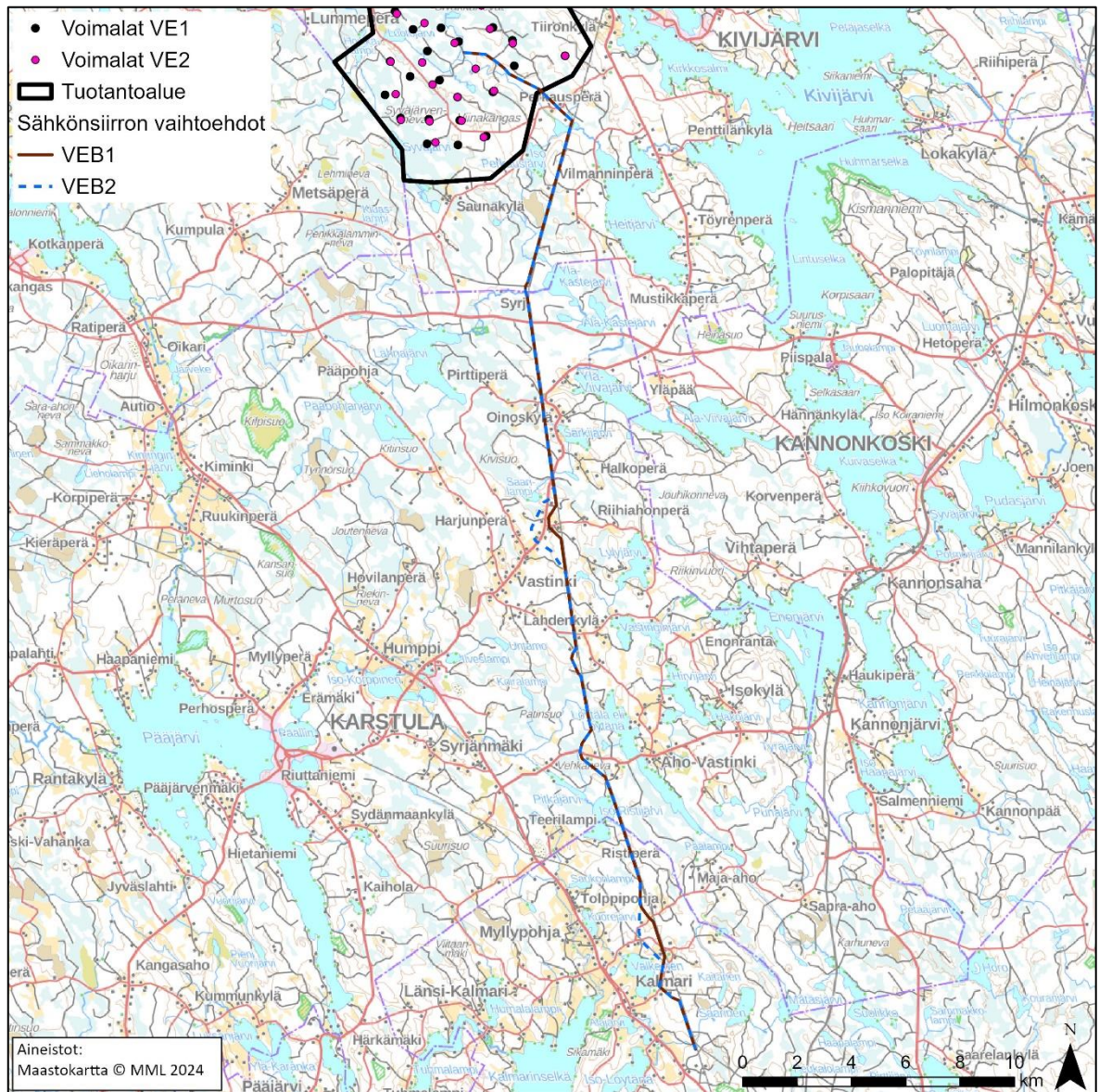
Kuva 1.3. Sähkönsiirtoyhteysvaihtoehdo VEB1 etelään: 110 kV voimajohto tuotantoalueelta olemassa olevan Metsälinjan tuntumaan linjan länsipuolelle sekä Metsälinjaa etelään päin seuraten Saarijärvelle rakennettavalle sähköasemalle. Pituus 41,3 km. Sähkönsiirtoyhteysvaihtoehdo VEB2 etelään: 400 kV voimajohto tuotantoalueelta olemassa olevan Metsälinjan tuntumaan linjan länsipuolelle ja Metsälinjaa etelään päin seuraten Saarijärvelle rakennettavalle sähköasemalle. Pituus 42 km.
