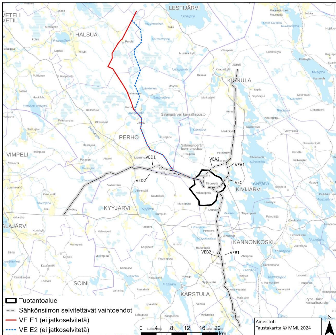
Kuva 4.8. YVassa tutkittavat sähkönsiirtoreitit (VEA1, VEA2, VEB1, VEB2, VEC, VED1 ja VED2) ovat esitetty kartassa mustalla katkoviivalla. Halsuan sähköasemalle tuotantoalueesta luoteeseen alustavasti harkitut sähkönsiirtoreitit, joita ei huomioida jatkoselvittelyissä, on esitetty punaisella viivalla ja sinisellä katkoviivalla.
