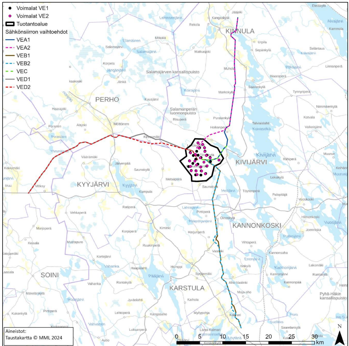
Kuva 3.2. Sähkönsiirron alustavat reittivaihtoehdot (VEA1, VEA2, VEB1, VEB2, VEC, VED1, VED2) tuotantoalueelta.
