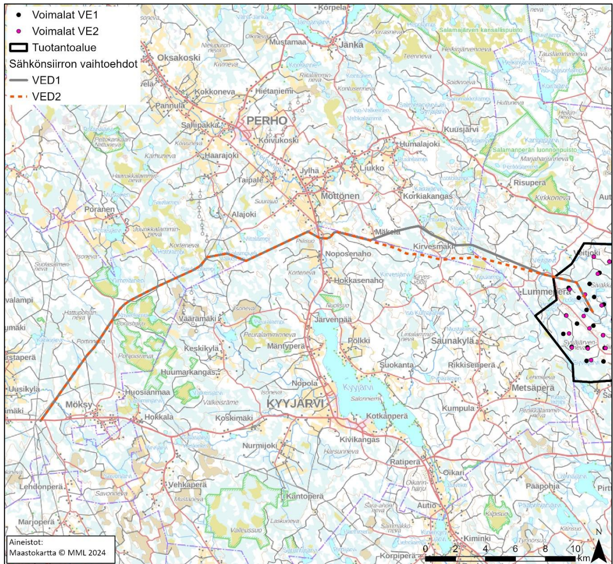
Kuva 1.4. Sähkönsiirtoyhteysvaihtoehto VED1: 400/110 kV voimajohto tuotantoalueelta länteen kohti Alajärvi - Perho A 110 kV voimajohtoa, jonka vierellä linjaa seuraten Alajärven sähköasemalle. Kiertää Kirvesvuoren tuulivoima-alueen. Pituus 44,7 km. Sähkönsiirtoyhteysvaihtoehto VED2: 400/110 kV voimajohto tuotantoalueelta länteen kohti Alajärvi - Perho A 110 kV voimajohtoa, jonka vierellä linjaa seuraten Alajärven sähköasemalle. Linja suunniteltu Kirvesvuoren tuulivoima-alueen läpi. Pituus 44,3 km.
