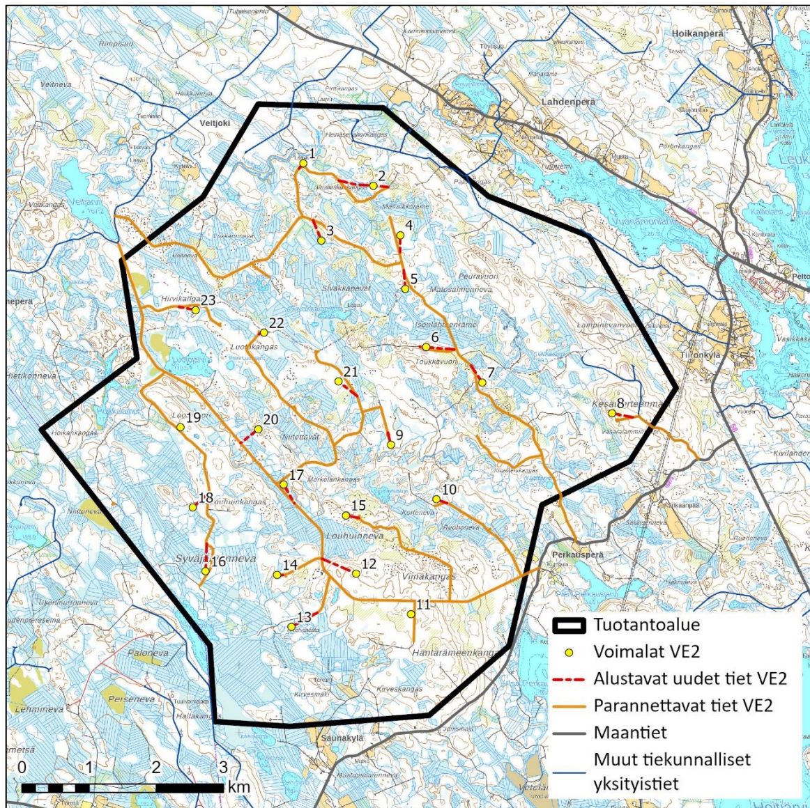
Kuva 4.4. Alustava suunnitelma VE2 parannettavista ja uusista teistä tuotantoalueella.
