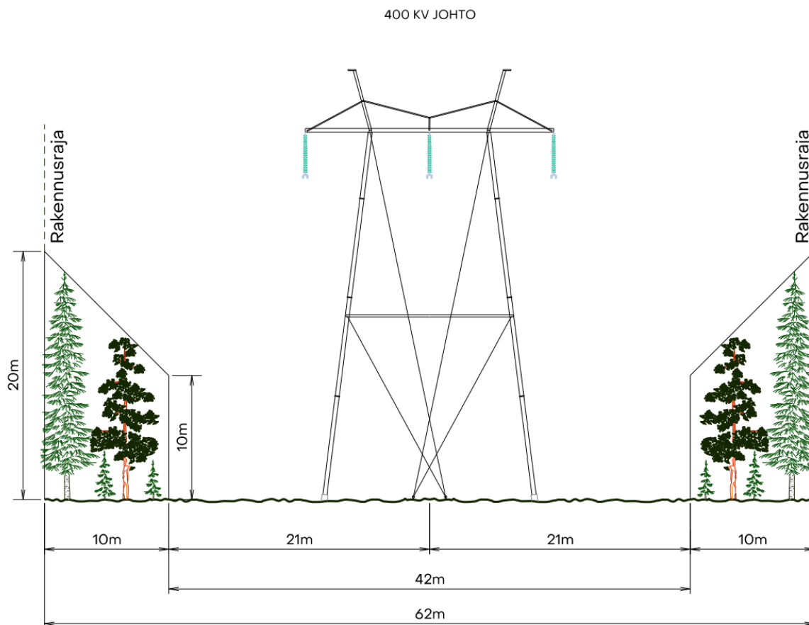
Kuva 4.10. Uuden rakennettavan 400 kV voimajohdon voimajohtoalueen periaatekuva. Johtoaukean leveys on yleensä noin 42 m. Lisäksi johtoaukean molemmin puolin on 10 metrin reunavyöhykkeet, joilla puuston ei anneta kasvaa liian korkeaksi.
