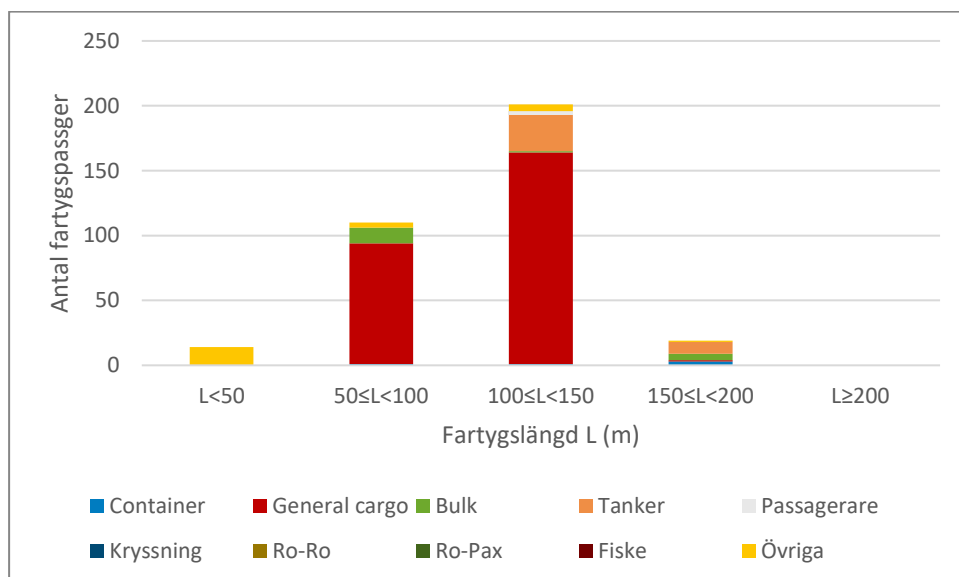
Figur 5 Antal fartygspassager över linje 2 fördelat på fartygstyp och längdintervall.
