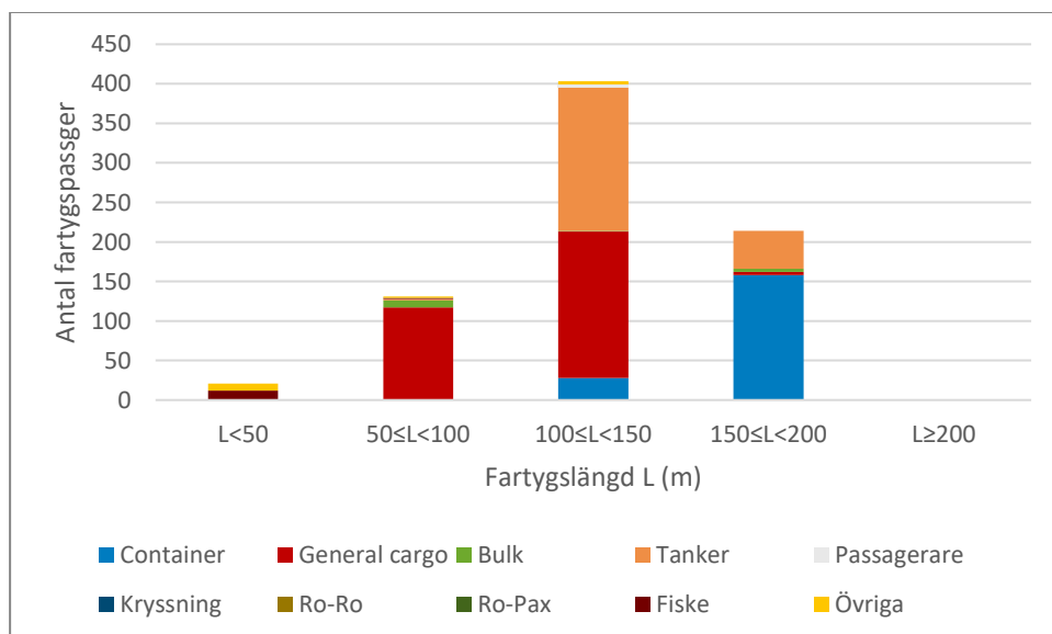
Figur 12 Antal fartygspassager över linje 7 fördelat på fartygstyp och längdintervall.
