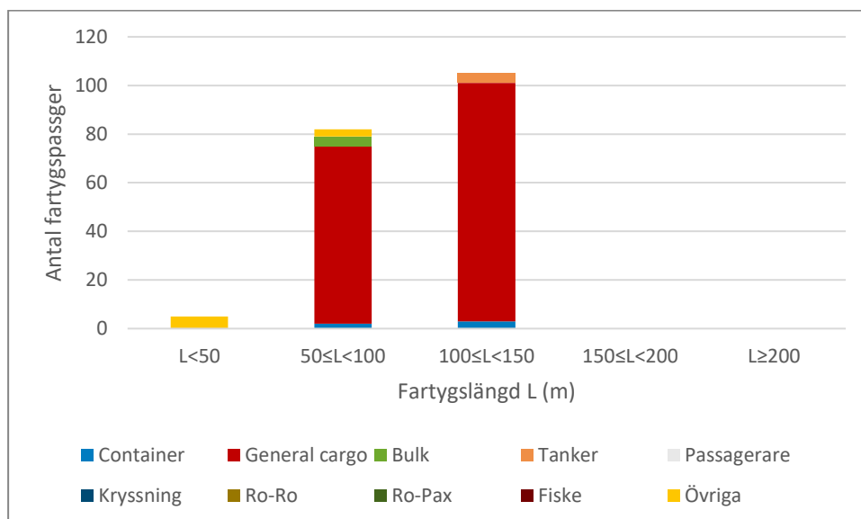
Figur 9 Antal fartygspassager över linje 5 fördelat på fartygstyp och längdintervall.
