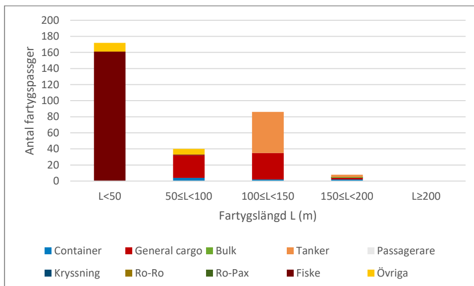
Figur 7 Antal fartygspassager över linje 3 fördelat på fartygstyp och längdintervall.
