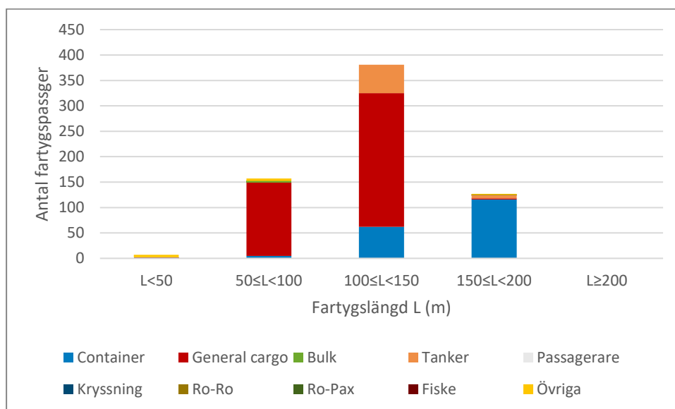
Figur 10 Antal fartygspassager över linje 6 fördelat på fartygstyp och längdintervall.
