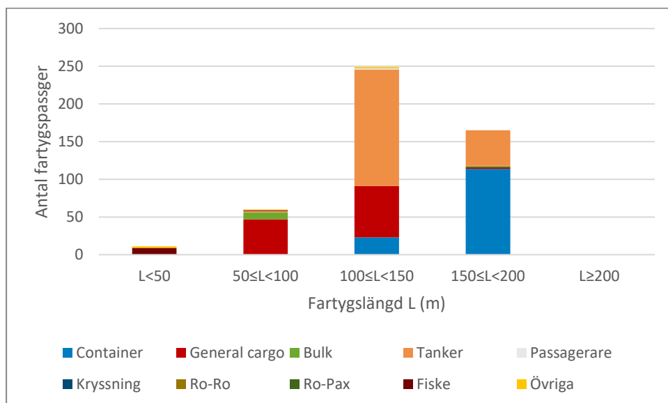
Figur 14 Antal fartygspassager över linje 7 som trafikerat Gävle fördelat på fartygstyp och längdintervall
