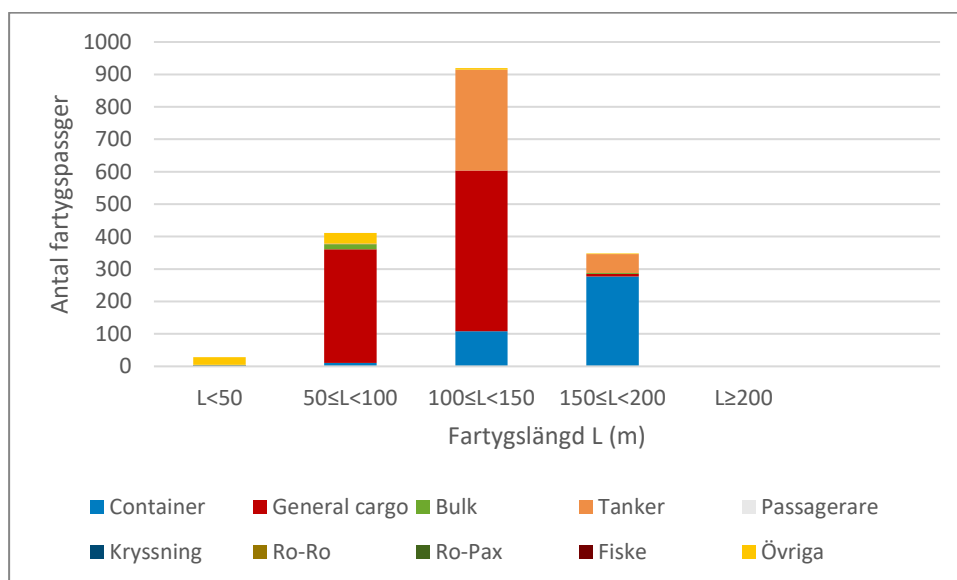
Figur 8 Antal fartygspassager över linje 4 fördelat på fartygstyp och längdintervall.
