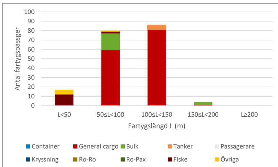
Figur 3 Antal fartygspassager över linje 1 fördelat på fartygstyp och längdintervall.
