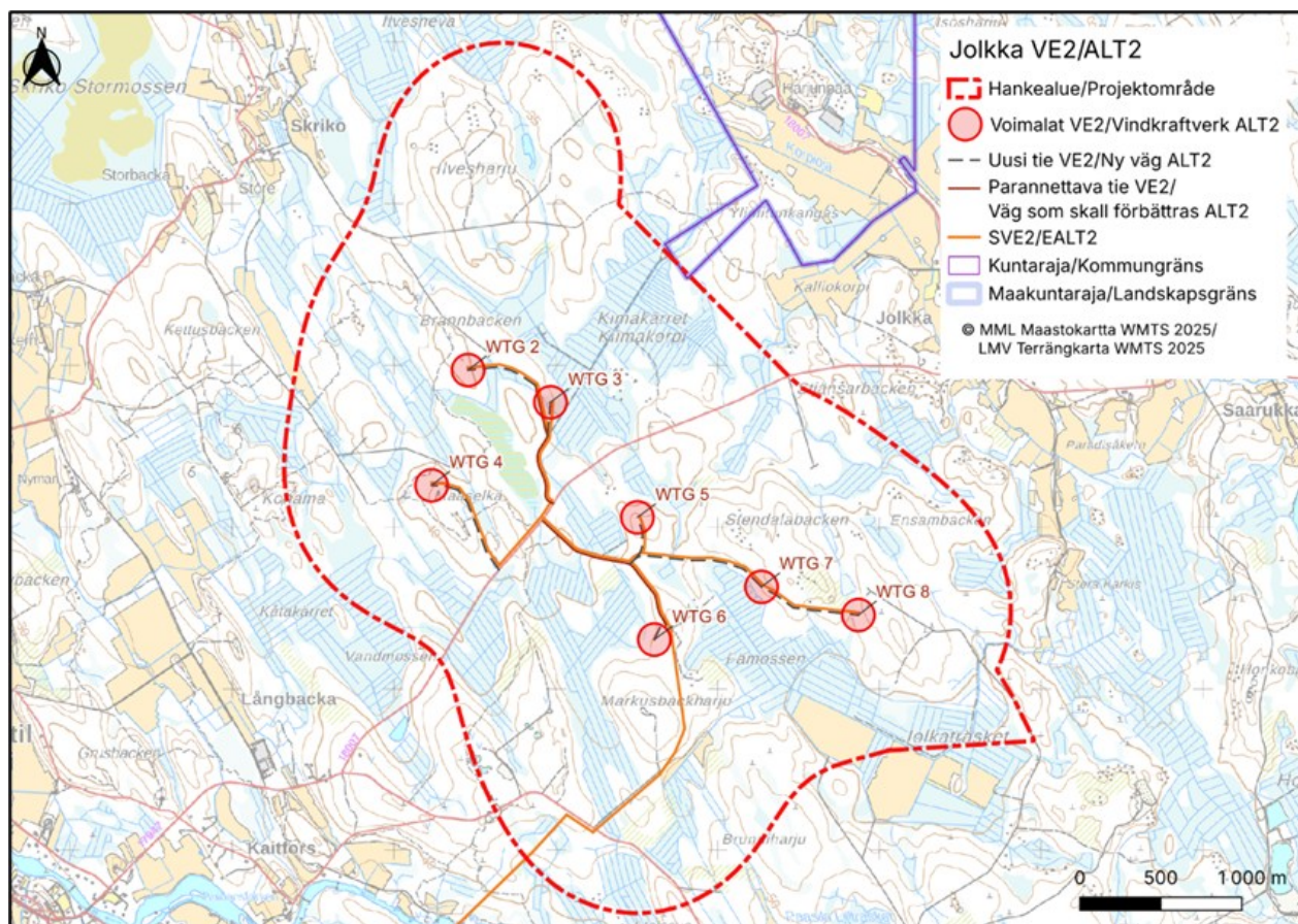
Bild 3 Layout för kraftverken i Jolikka vindkraftspark i projektalternativ ALT2.
