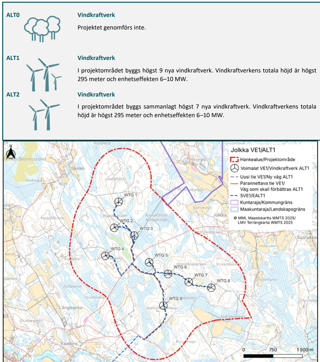
Bild 2 Layout för kraftverken i Jolkka vindkraftspark i projektalternativ ALT1.
