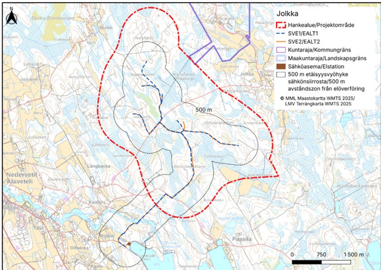
Bild 4 Projektets planerade jordkabelrutter och elstation.
