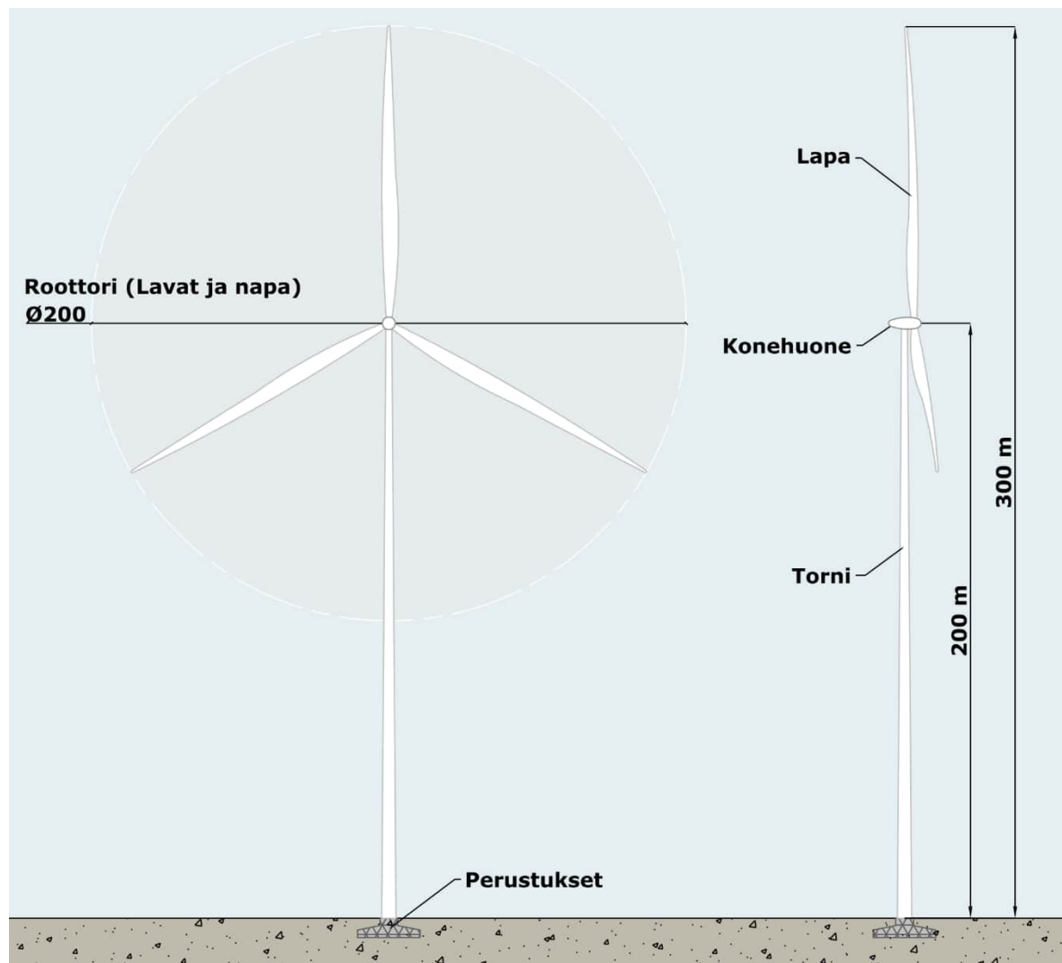
Kuva 3.1. Tuulivoimalan rakenne ja koko.
