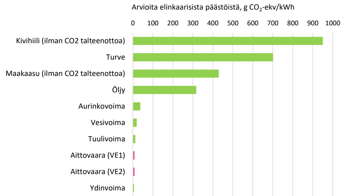
Kuva 26.1. Arvioita muiden sähköntuotantomenetelmien elinkaarisista päästöistä.
