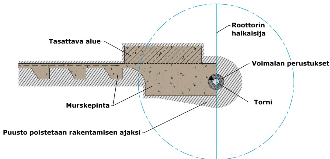
Kuva 3.3. Periaatekuva voimalan nostoalueesta.
