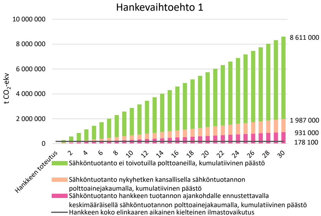
Kuva 26.2. Sähköntuotannon kumulatiiviset päästöt sekä hankkeen koko elinkaaren aikainen kielteinen ilmastovaikutus hankevaihtoehdossa 1.
