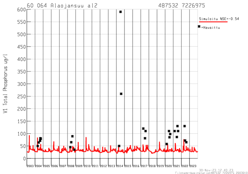
Kuva 23.2. Alaoja-Heteojan Alaojansuu al2 -näytepisteeseen mitattu (piste) ja simuloitu (viiva) kokonaisfosforipitoisuus vuosina 2003–2023 (SYKE 2023).
