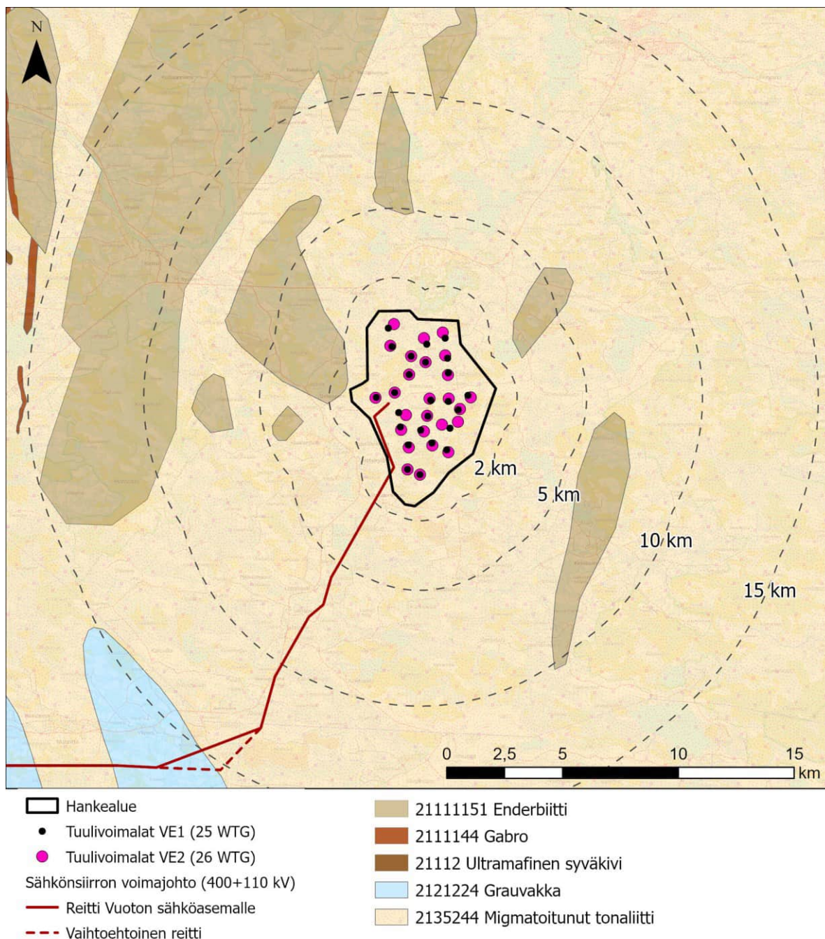
Kuva 22.2. Hankealueen kallioperä (GTK Kallioperä 1:170 000).
