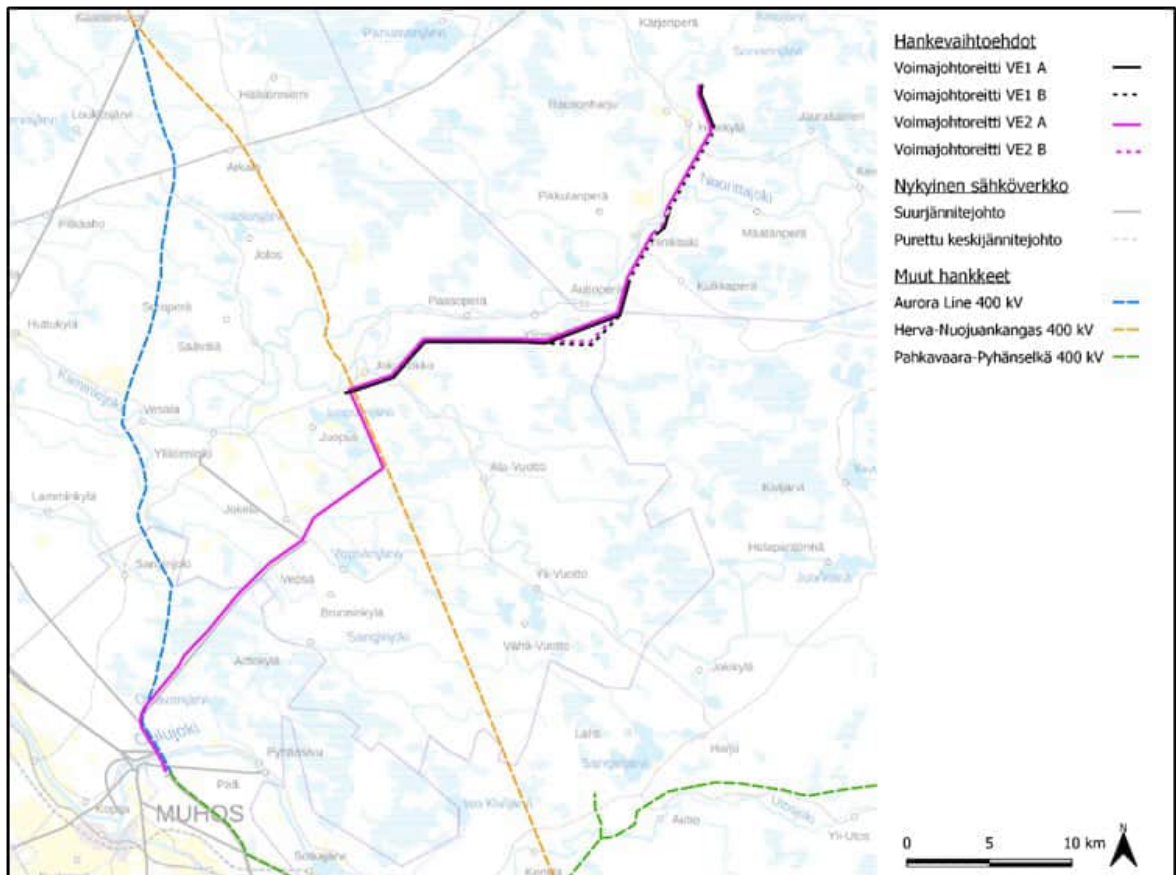
Kuva 32.2. Nykyisten, rakenteilla olevien ja suunnitteilla olevien voimajohtojen sijoittuminen suhteessa Aittovaara-Pyhänselkä 400+110 kV voimajohtoon, joka osa Aittovaaran tuulivoimahankkeen sähkönsiirtoa. (Kuvan lähde: Aittovaara-Pyhänselkä 400+110 kV voimajohtohankkeen YVA-selostuksen luonnosmateriaali 19.6.2024, Sitema Oy)
