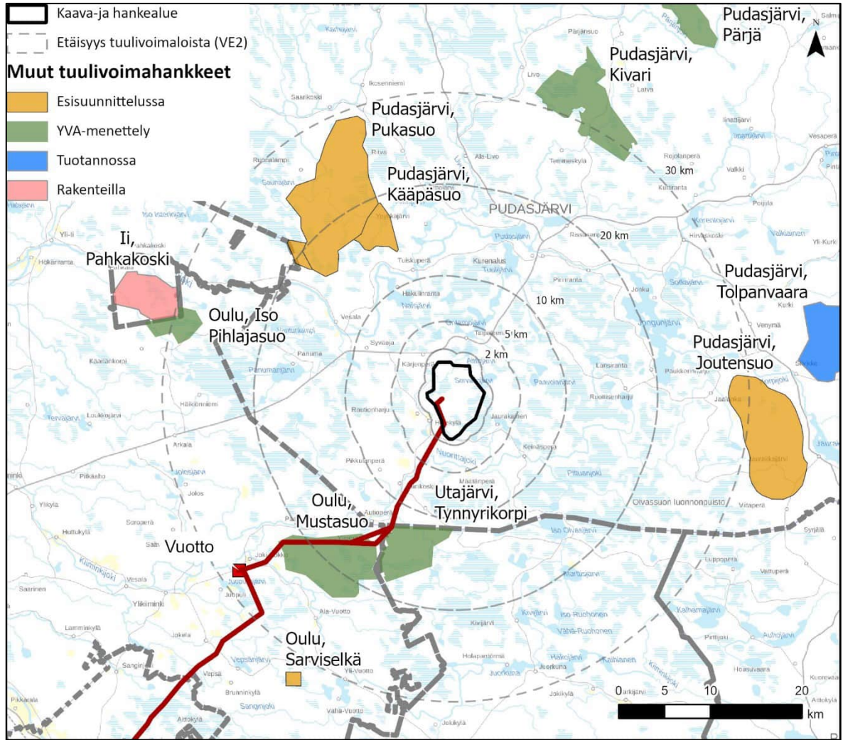
Kuva 32.1. Hankealueen läheiset tiedossa olevat tuulivoimahankkeet (tilanne 19.6.2024) ja Aittovaara-Pyhänselkä 400+110 kV voimajohdon reitti tumman punaisella viivalla sekä Vuoton tulevan sähköaseman paikka.
