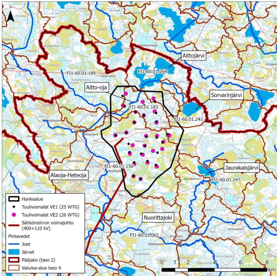
Kuva 23.1. Hankealueen sijoittuminen tason 4 valuma-alueille (Syke) sekä pintavedet hankealueen läheisyydessä.
