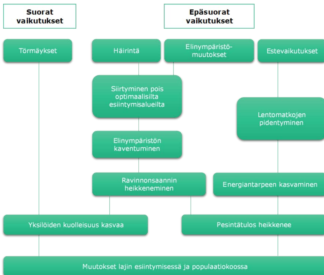
Kuva 20.5. Yleistetty kaavio tuulivoimatuotantoalueiden linnustovaikutuksista.
