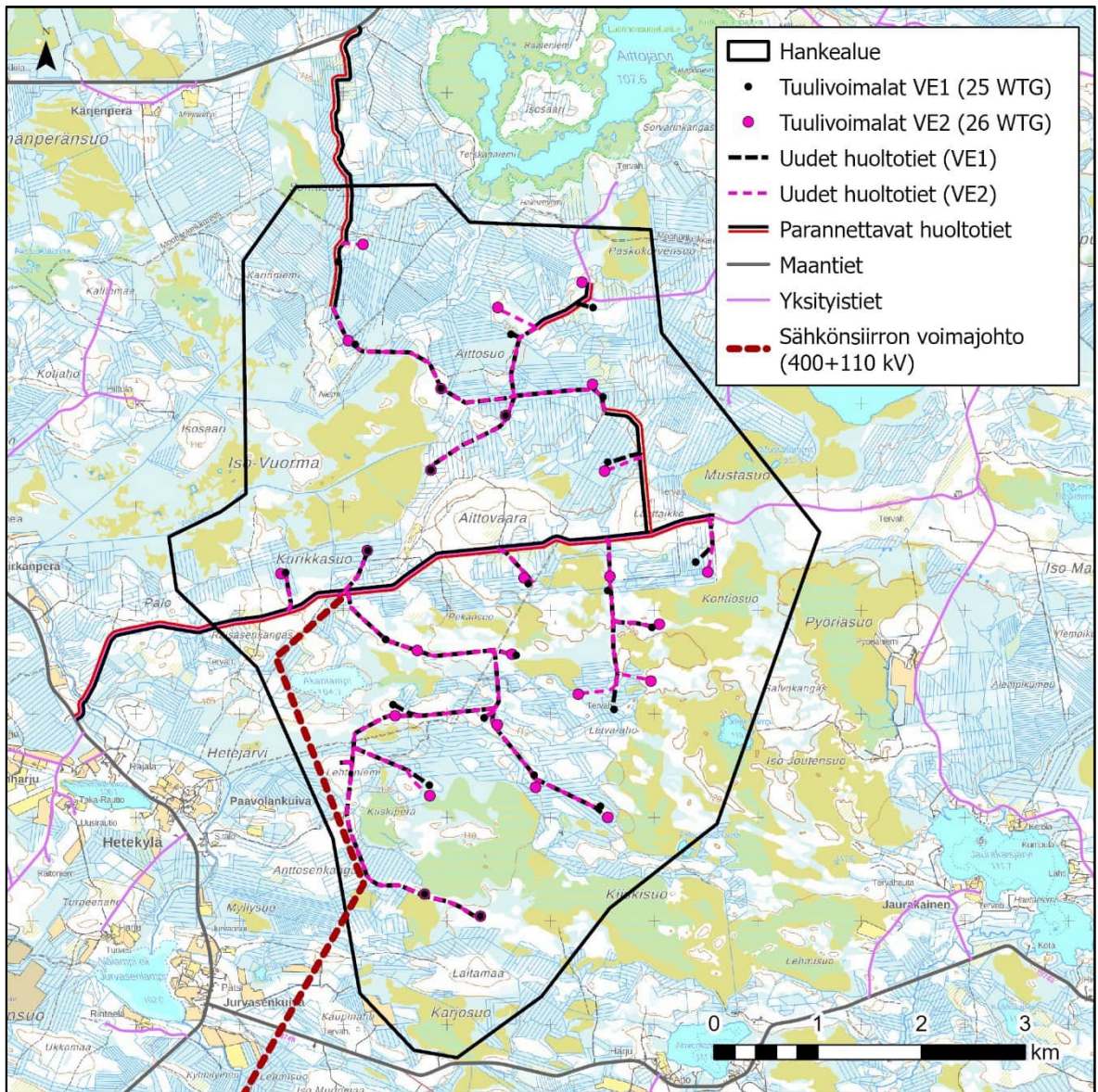
Kuva 27.2. Hankealueen suunnitellut sisääntulotiet sekä olemassa olevat parannettavat tieyhteydet ja uudet huoltotiet voimaloiden välillä.
