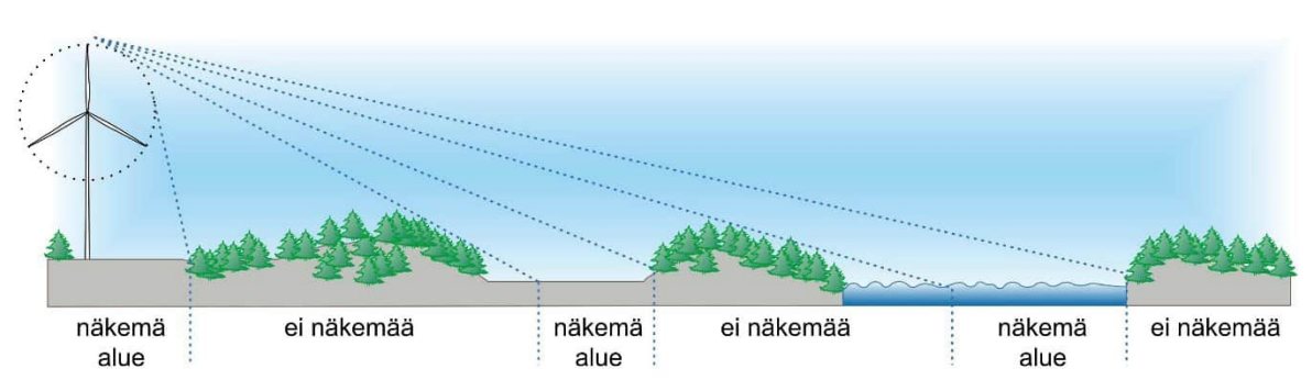
Kuva 16.4. Periaatekuva, miten puuston ja maastonmuotojen aiheuttama katvevaikutus vaikuttaa tuulivoimaloiden näkyvyyteen.
