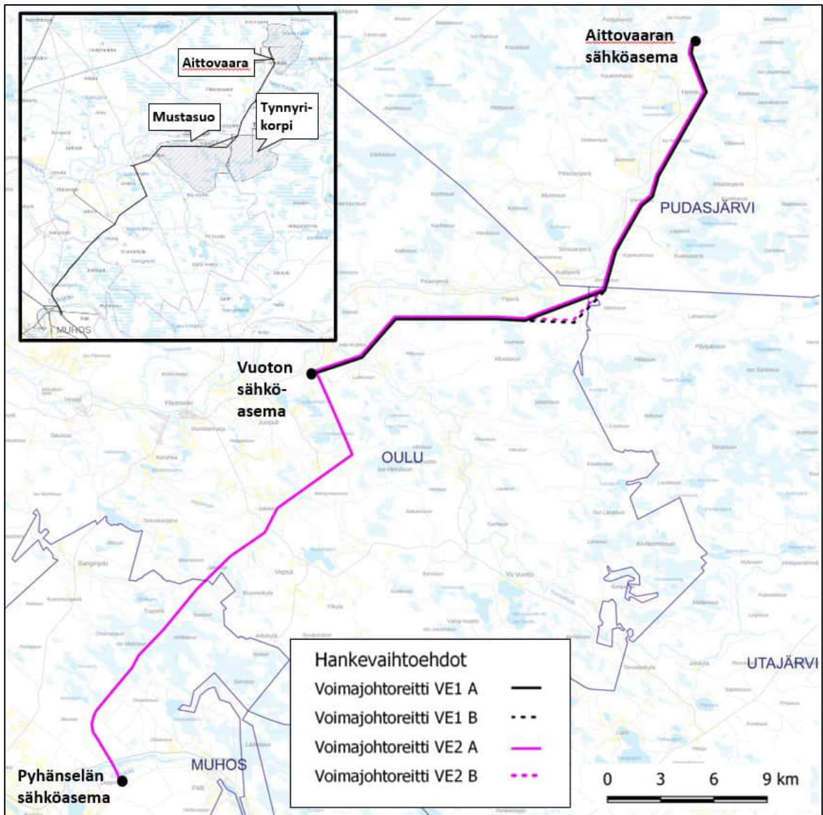
Kuva 4.3. Aittovaara-Pyhänselkä 400+110 kV voimajohtohankkeen erillisessä YVA-menettelyssä tarkastellut vaihtoehdot VE1(A/B) Vuoton sähköasemalle tai VE2(A/B) Pyhänselän sähköasemalle. Alavaihtoehtojen A ja B reitti eroaa Mustasuon-Tynnyrikorven hankealueiden välisellä alueella sinne sijoitettavasta sähköaseman paikasta riippuen. Voimajohtohanke toteuttaa Aittovaaran tuulivoimahankkeen sekä Mustasuo-Tynnyrikorven tuulivoimahankkeen sähkönsiirtoa hankealueilta kantaverkkoon. (Kuvan lähde: Sitema Oy, Aittovaara-Pyhänselkä 400+110 kV voimajohtohankkeen YVA-selostuksen luonnosmateriaali 19.6.2024)
