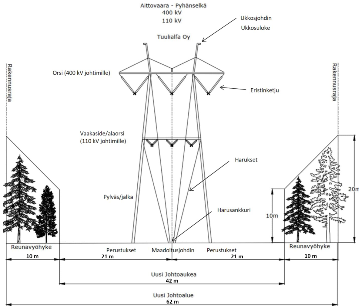
Kuva 3.6. Periaatekuva Aittovaara-Pyhänselkä 400+100 kV:n ilmajohdon rakenteista ja mitoista sekä ja voimajohtoon liittyvistä erityiskäsitteistä (Kuvan lähde: Sitema Oy 2023).
