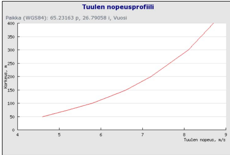
Kuva 3.8. Hankealueen tuulennopeus korkeuden suhteen (Tuuliatlas 2022).
