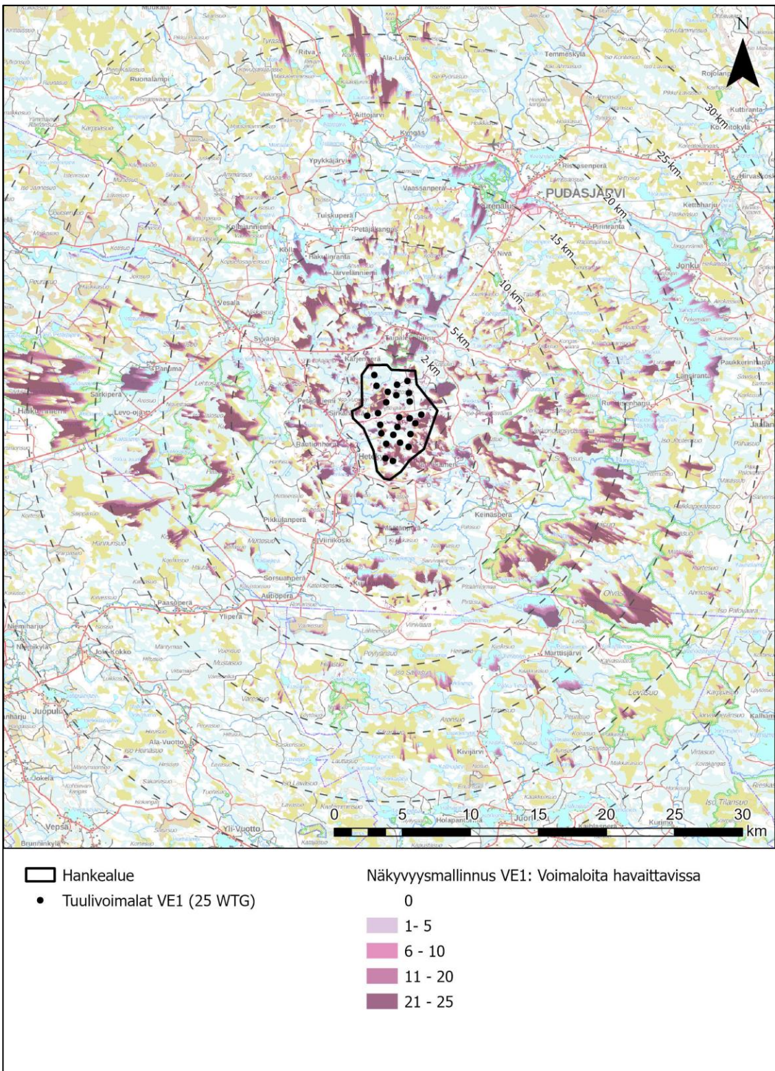
Kuva 1.2. Näkemäalueanalyysi hankevaihtoehdon VE1 tuulivoimaloista (AFRY Finland Oy). Tarkastelualue 25 km voimaloista.
