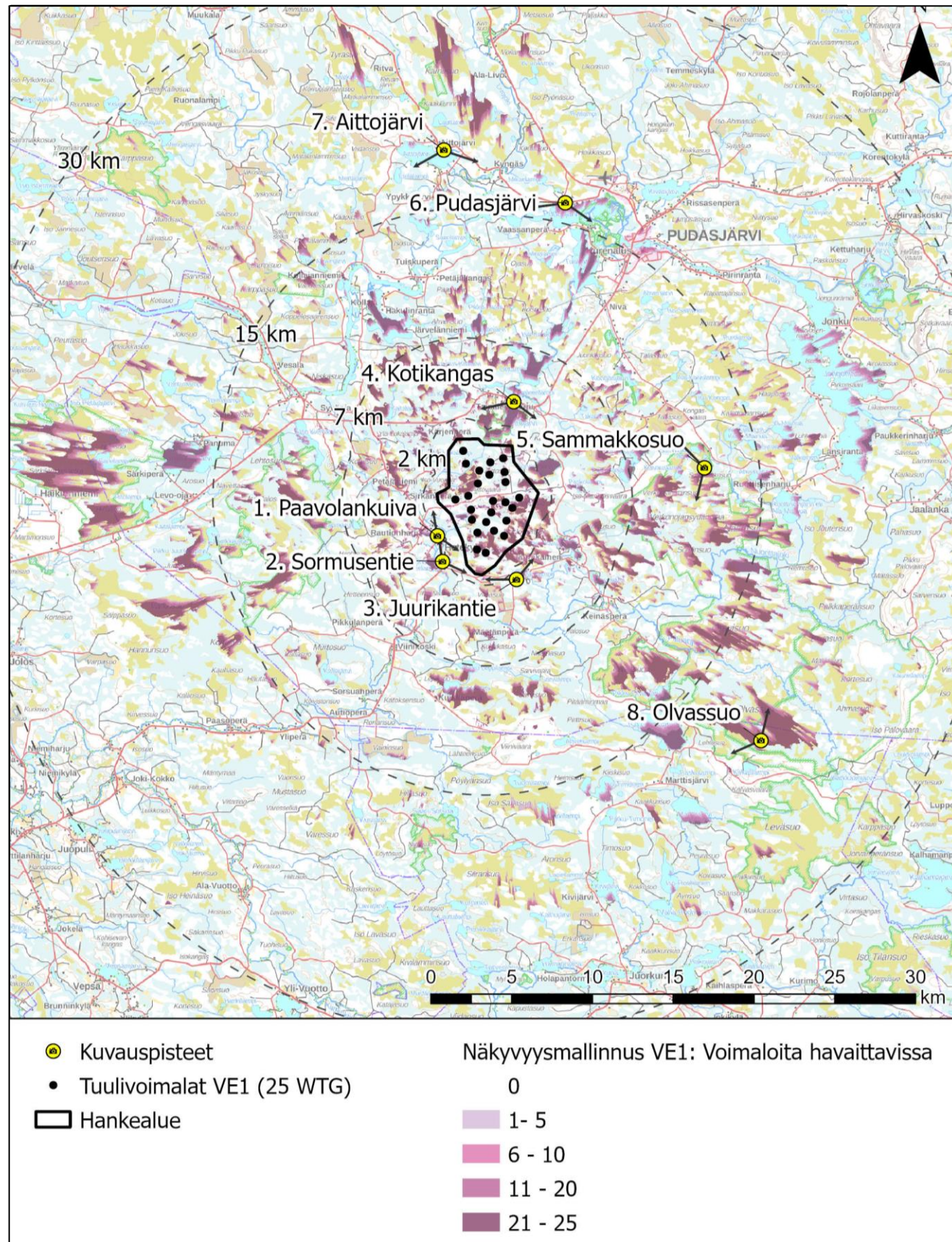
Kuva 1.6. Näkyyvysaluemallinnus hankevaihtoehdon VE1 tuulivoimaloista (AFRY Finland Oy). Karttaan merkitty havainnekuvien kuvanottoapaikat (kuvauspisteet).
