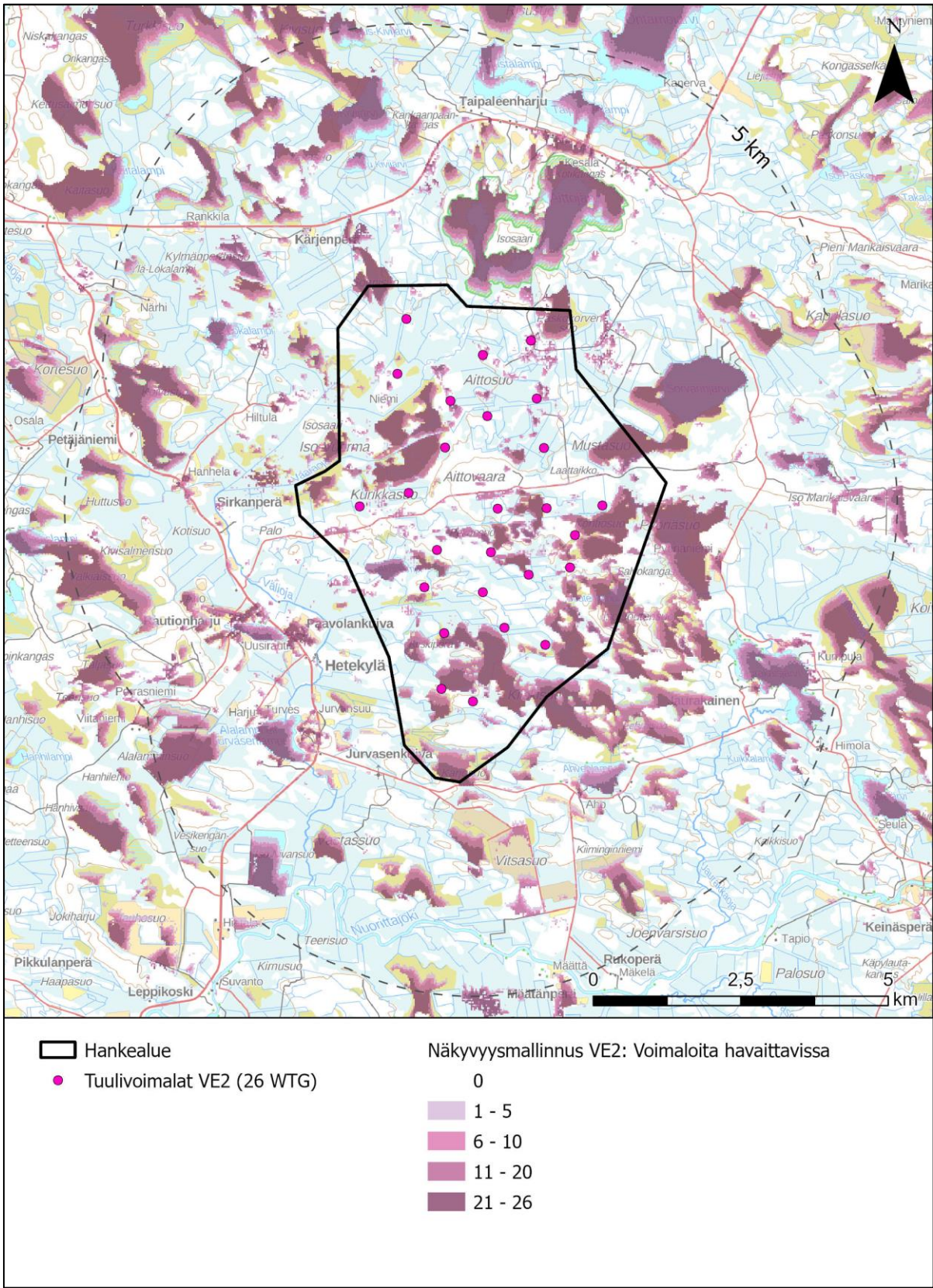
Kuva 1.3. Näkemäalueanalyysi hankevaihtoehdon VE2 tuulivoimaloista (AFRY Finland Oy). Lähialue 5 km voimaloista.
