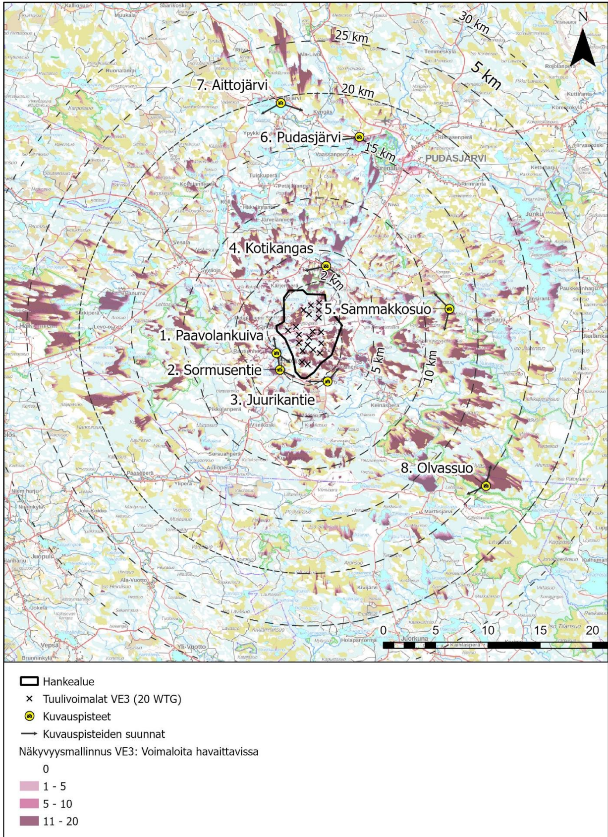
Kuva 1.9. Näkyvyysaluemallinnus hankevaihtoehdon VE3 tuulivoimaloista (AFRY Finland Oy). Karttaan merkitty havainnekuvien kuvanottoapaikat (kuvauspisteet).
