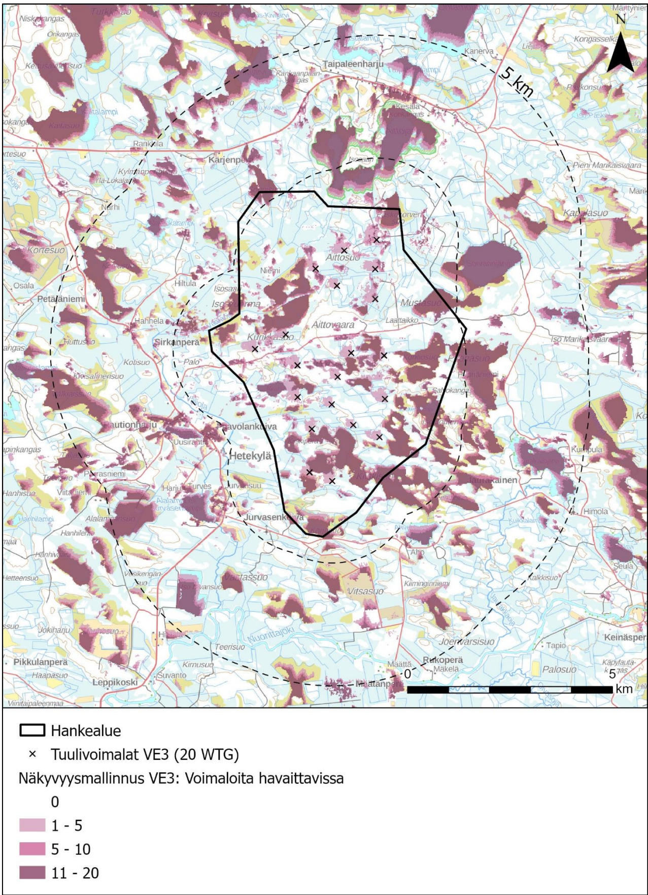
Kuva 1.4. Näkemäalueanalyysi hankevaihtoehdon VE3 tuulivoimaloista (AFRY Finland Oy). Lähialue 5 km voimaloista.
