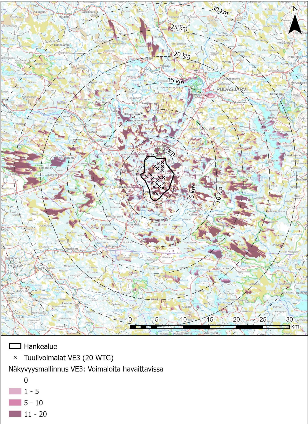
Kuva 1.5. Näkemäalueanalyysi hankevaihtoehdon VE3 tuulivoimaloista (AFRY Finland Oy). Tarkastelualue 25 km voimaloista.
