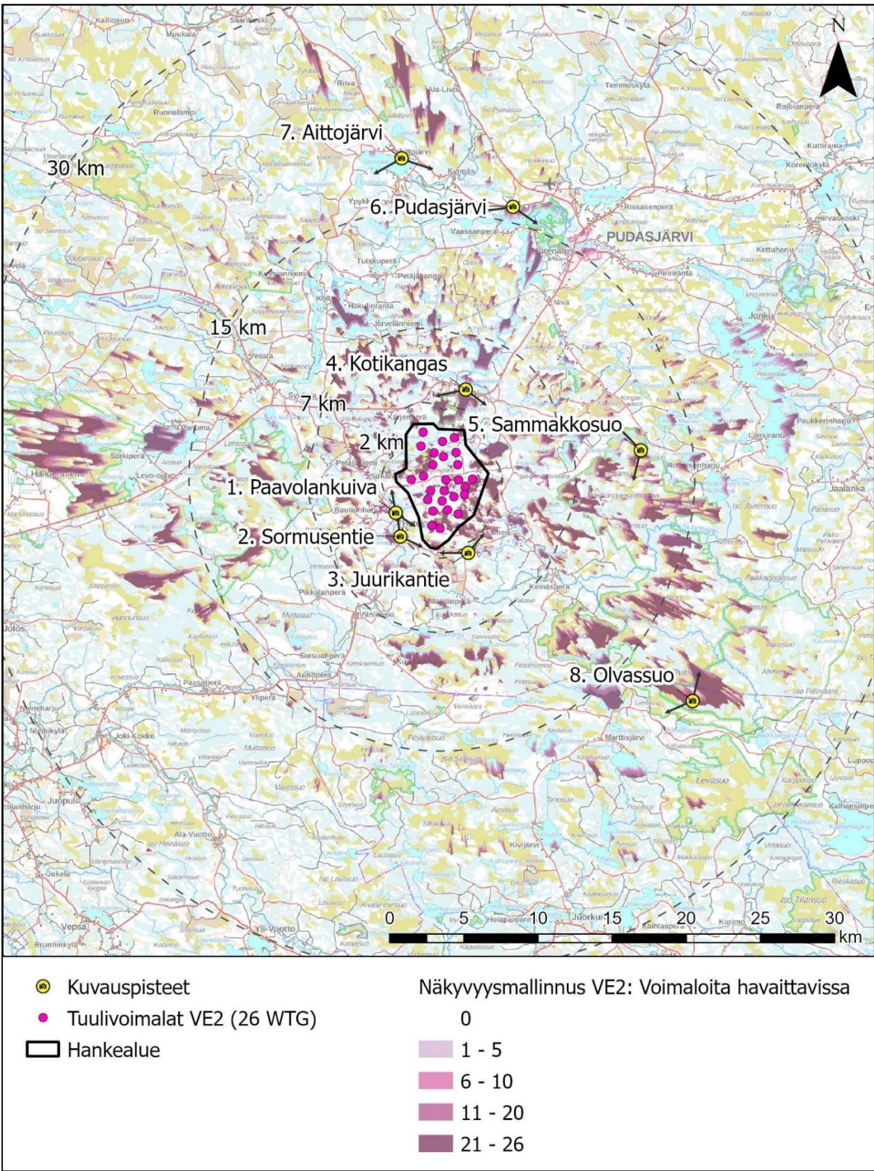
Kuva 1.8. Näkyvyysaluemallinnus hankevaihtoehdon VE2 tuulivoimaloista (AFRY Finland Oy). Karttaan merkitty havainnekuvien kuvanottoapaikat (kuvauspisteet).
