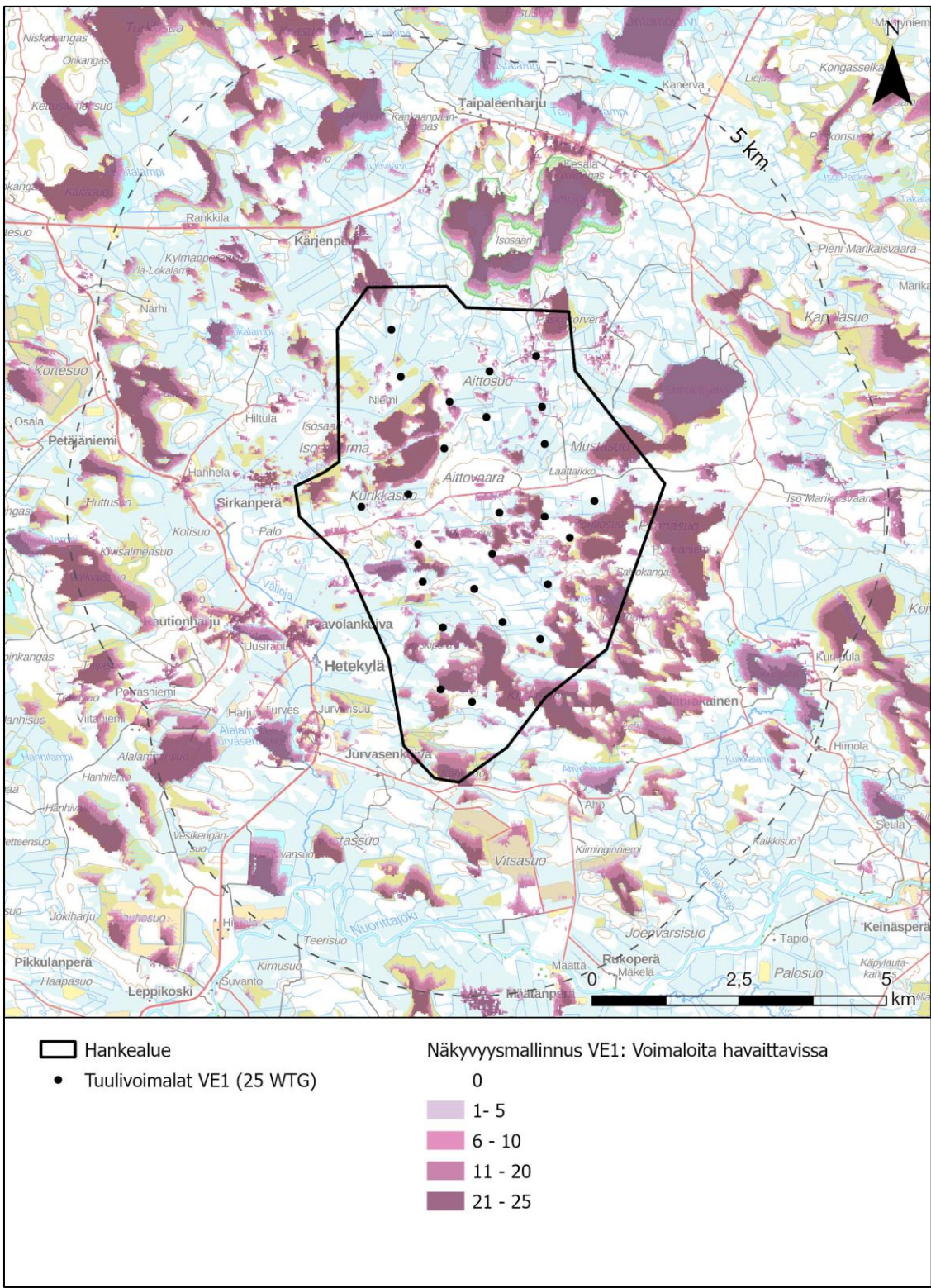
Kuva 1.1. Näkemäalueanalyysi hankevaihtoehdon VE1 tuulivoimaloista (AFRY Finland Oy). Lähialue 5 km voimaloista.
