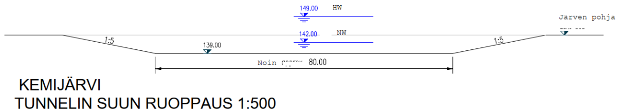
Kuva 2-3. Kuusilahteen ruopattavan kanaalin alustava poikkileikkauskuva (Afryst Austria GmbH 2023).
