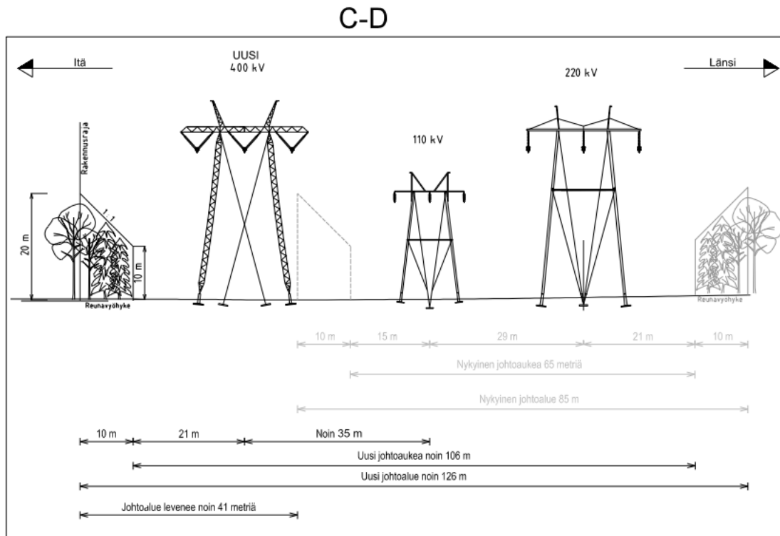
Kuva 2-10. Poikkileikkaus sillä osuudella, jossa johtoalueella on 110 kV, 220 kV ja 400 kV voimajohto samassa johtokäytävässä, eli välillä C-D (Kuva 2-7).
