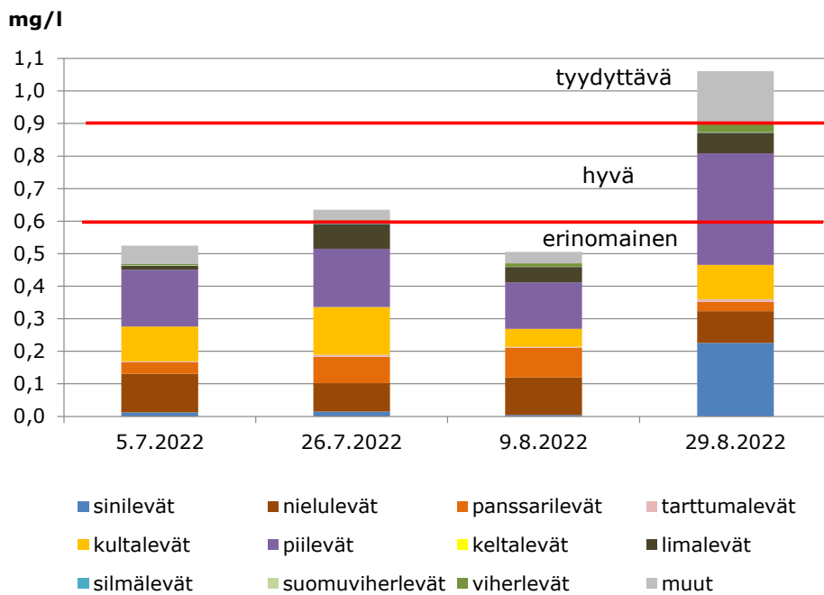
Kuva 5-2. Kemijärven Jumiskonselän (Ju106) tarkkailupisteen kasviplanktonnäytteiden biomassa ja lajistokoostumus vuonna 2022 (SYKE 2024g). Kesäkuun 2022 näytteen säilöntä oli epäonnistunut, joten ko. näytteen tuloksia ei esitetä tässä yhteydessä. Kuvaajassa on esitetty myös vertailun vuoksi Aroviidan ym. (2019) ekologisen tilan luokkarajat Sh-pintavesityypille.
