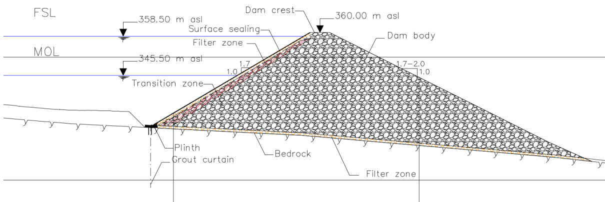
Kuva 2-5. Ylävaraston padon poikkileikkauskuva (Afray Austria GMBH 2023).
