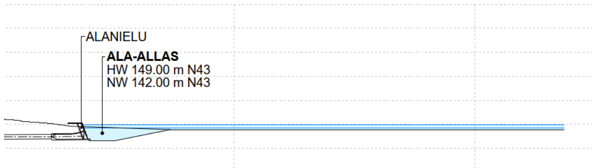
Kuva 2-2. Kuusilahteen kaivettavan syvänteen alustava pituusleikkauskuva (Afryst Austria GmbH 2023).
