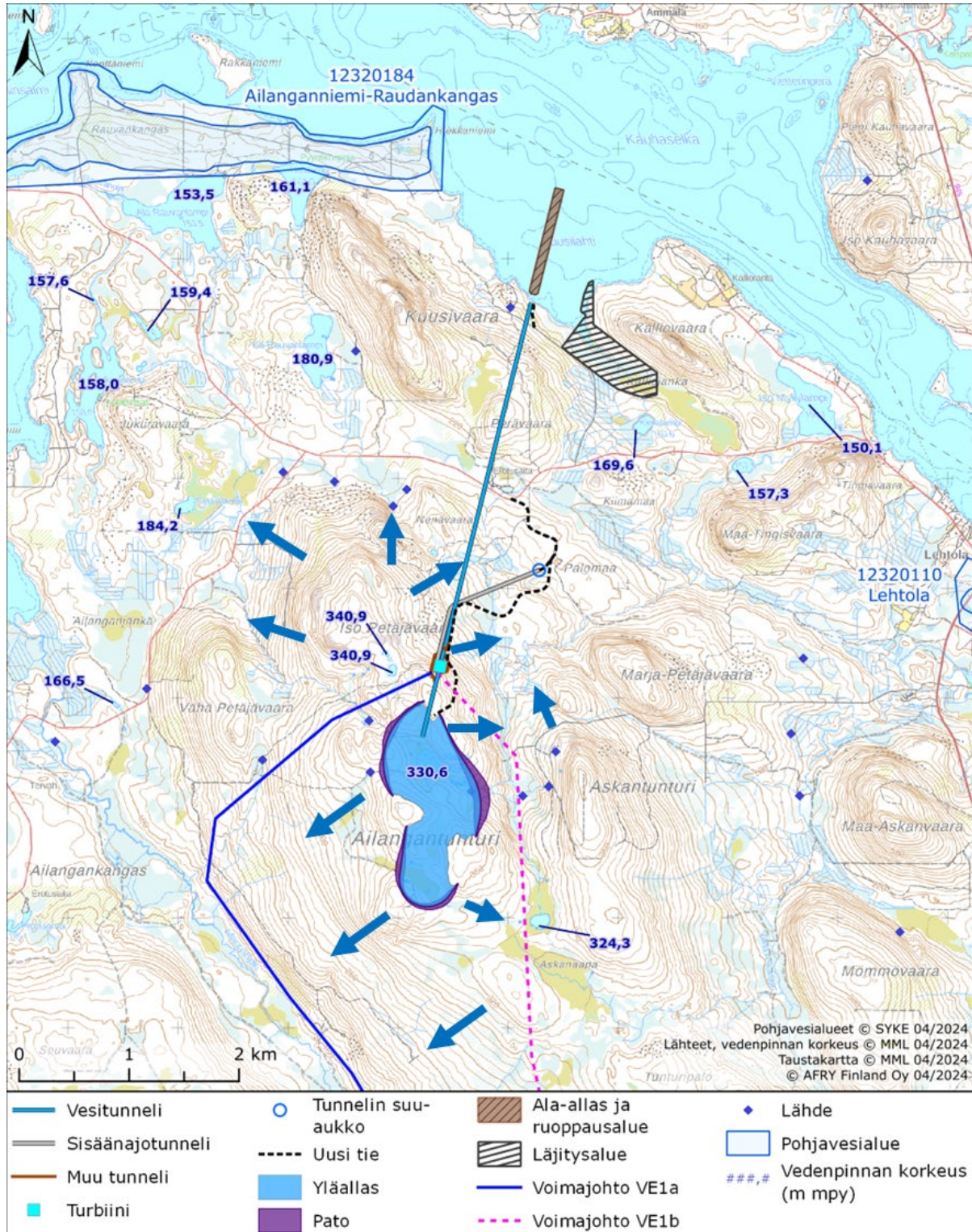
Kuva 6-9. Pumppuvoimalaitoksen hankealueen lähimmät pohjavesialueet, vedenpinnan korkeudet ja lähteet sekä vesipintojen gradientteihin perustuvat pohjaveden virtaussuunnat sinisillä nuolilla.
