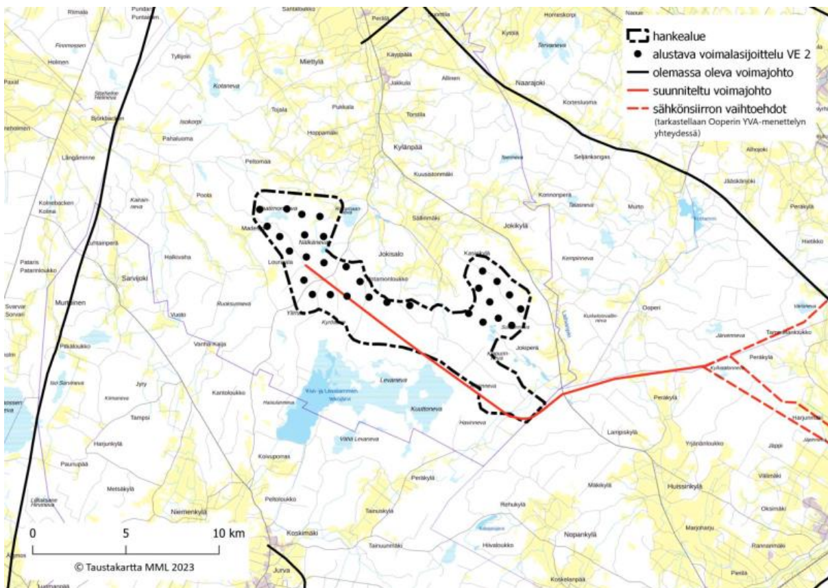
Alustava voimalasijoittelu VE2 (30 voimalan hanke)
