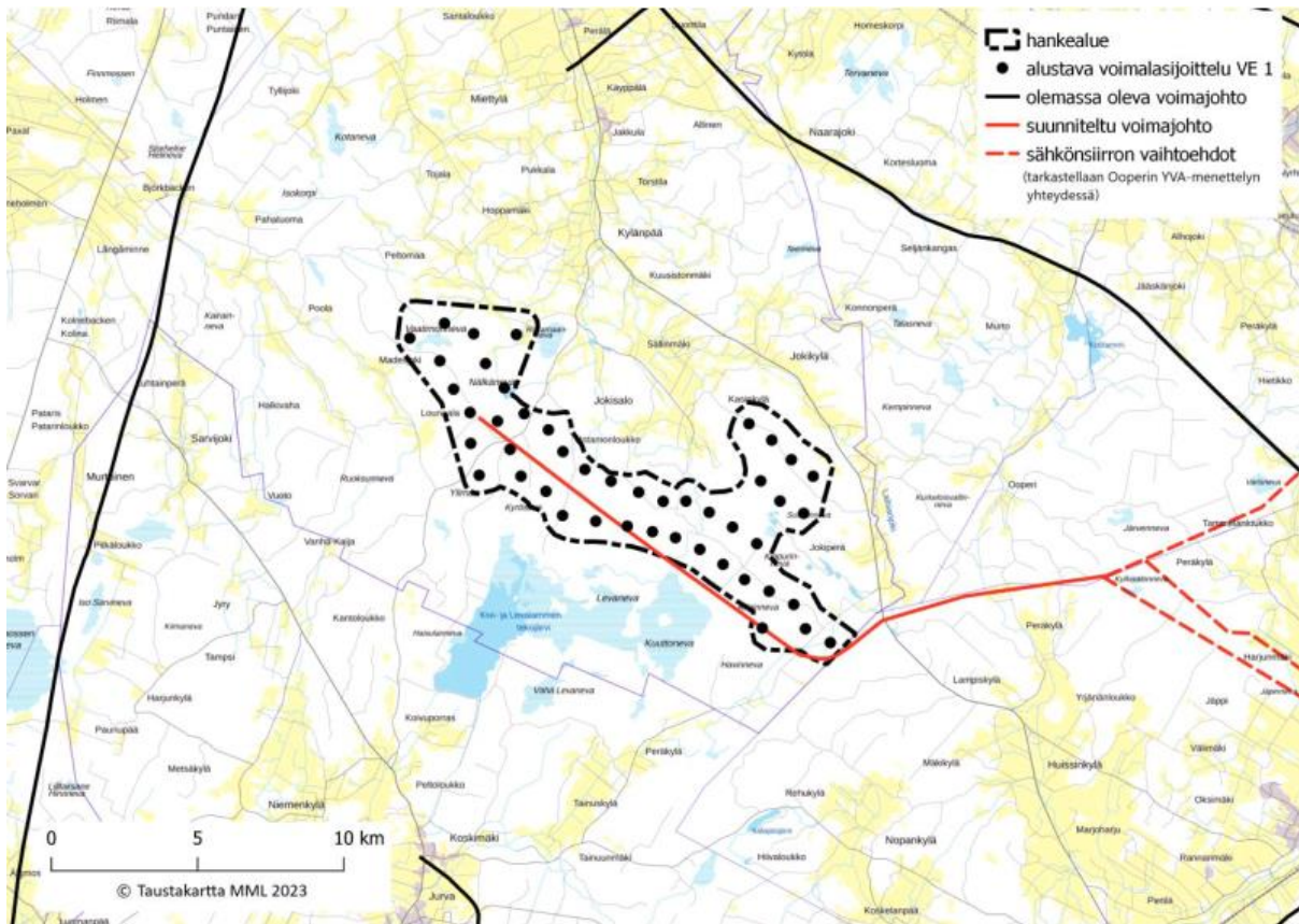
Alustava voimalasijoittelu VE1 (46 voimalan hanke)
