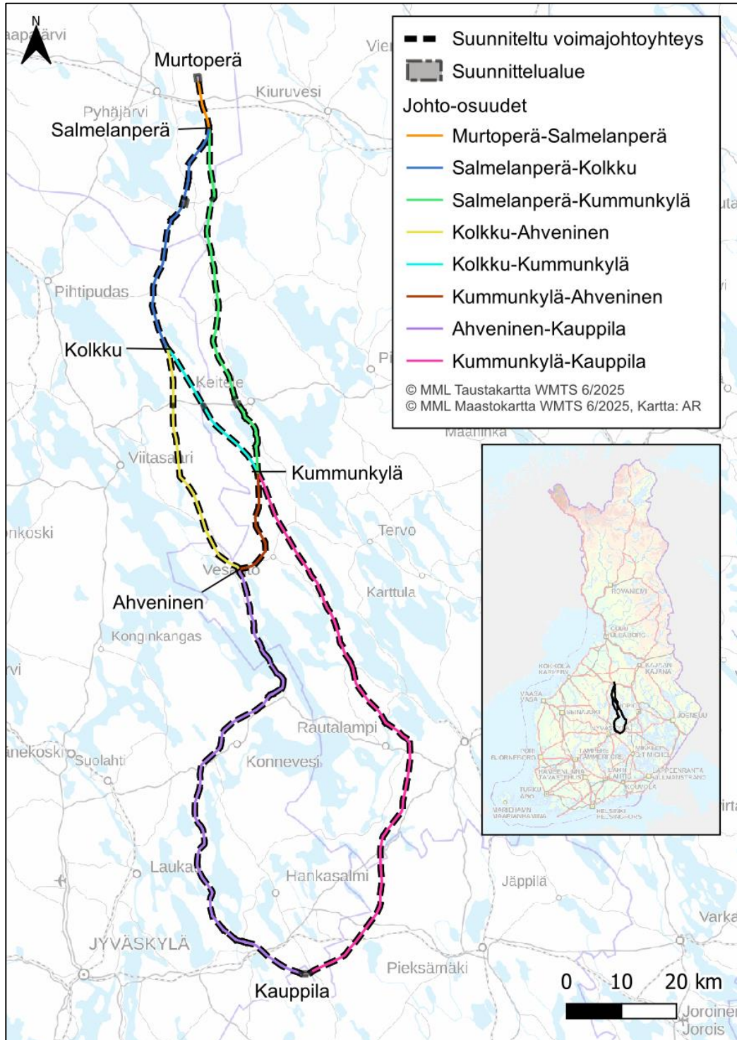
Kuva 4.1. Suunniteltu voimajohtoyhteys ja vaihtoehtoiset reitit Pyhäjärven Murtoperän ja Kangasniemen Kauppilan välillä.
