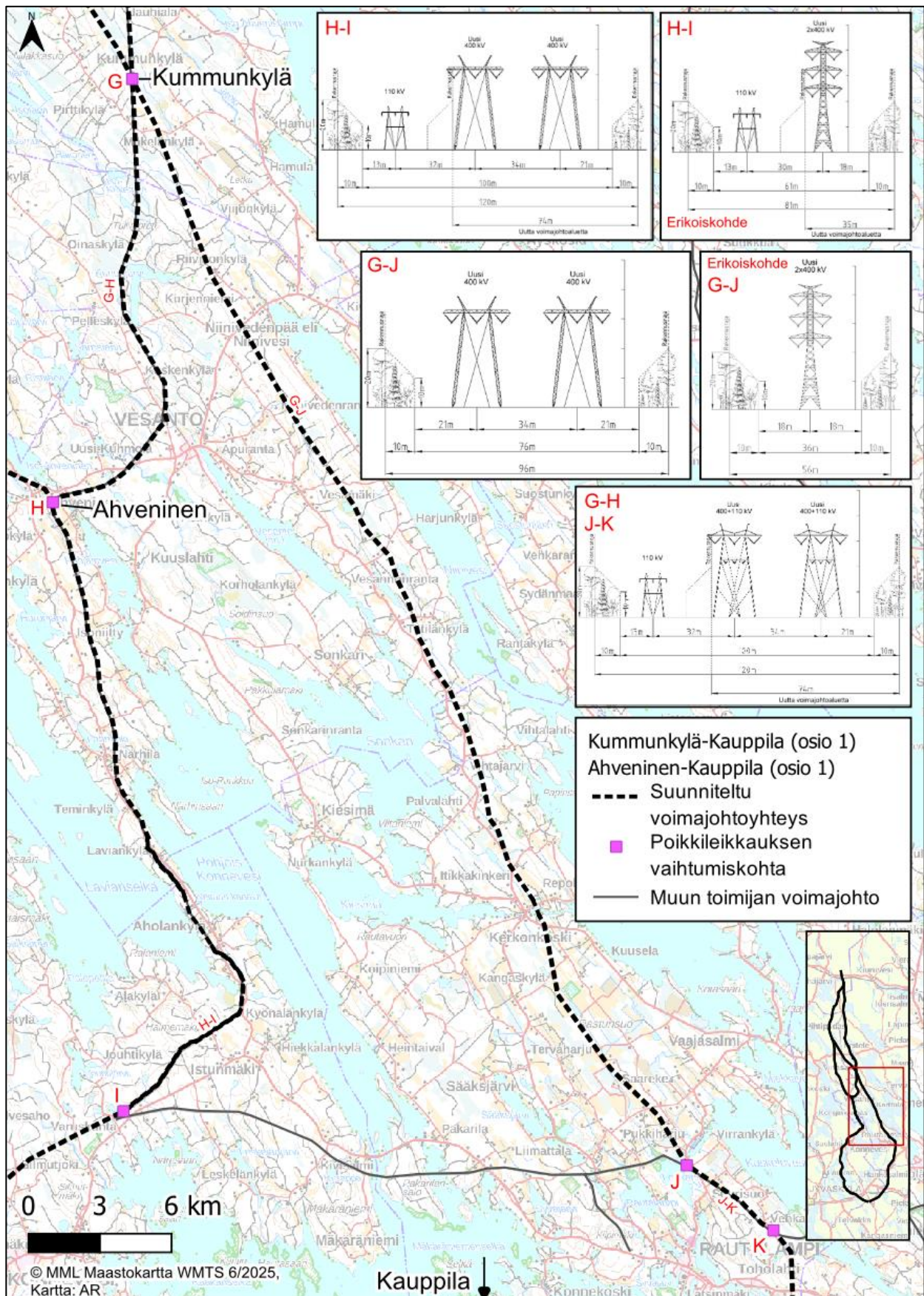
Kuva 4.7. YVA-menettelyssä tarkasteltavien voimajohtoreittien sijoittuminen Ahvenisen ja Kauppilan sekä Kummunkylän ja Ahvenisen (osioiden 1) välillä.
