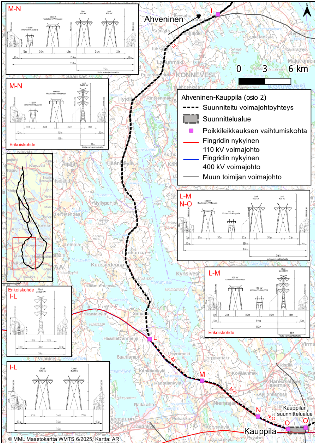
Kuva 4.8. YVA-menettelyssä tarkasteltavien voimajohtoreittien sijoittuminen Ahvenisen ja Kauppilan (osion 2) välillä.
