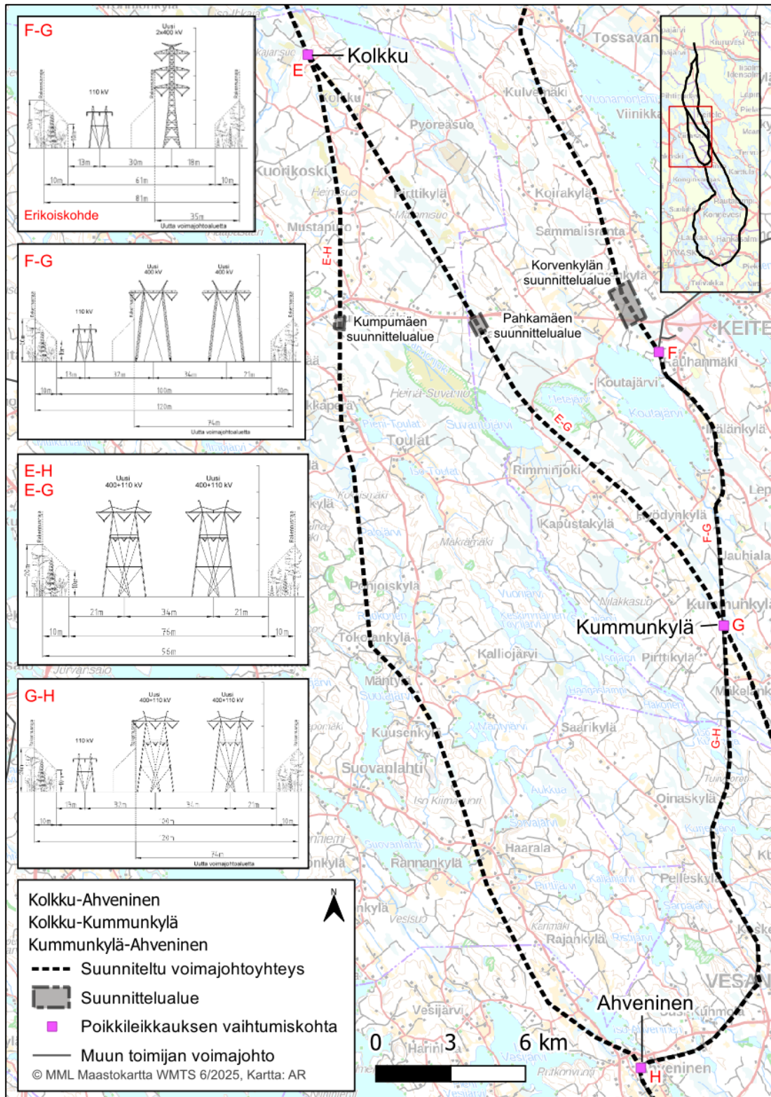
Kuva 4.6. YVA-menettelyssä tarkasteltavien voimajohtoreittien sijoittuminen Kolkun ja Ahvenisen, Kolkun ja Kummunkylän sekä Kummunkylän ja Ahvenisen välillä.
