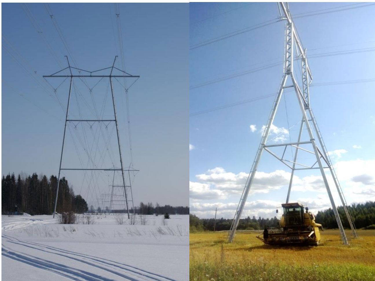
Kuva 4.10. Esimerkkikuvat eri pylvästyypeistä. Vasemmalla perusratkaisun mukainen 400+110 kilovoltin haruksin tuettu portaalipylväs ja oikealla vapaasti seisova harukseton peltopylväs.
