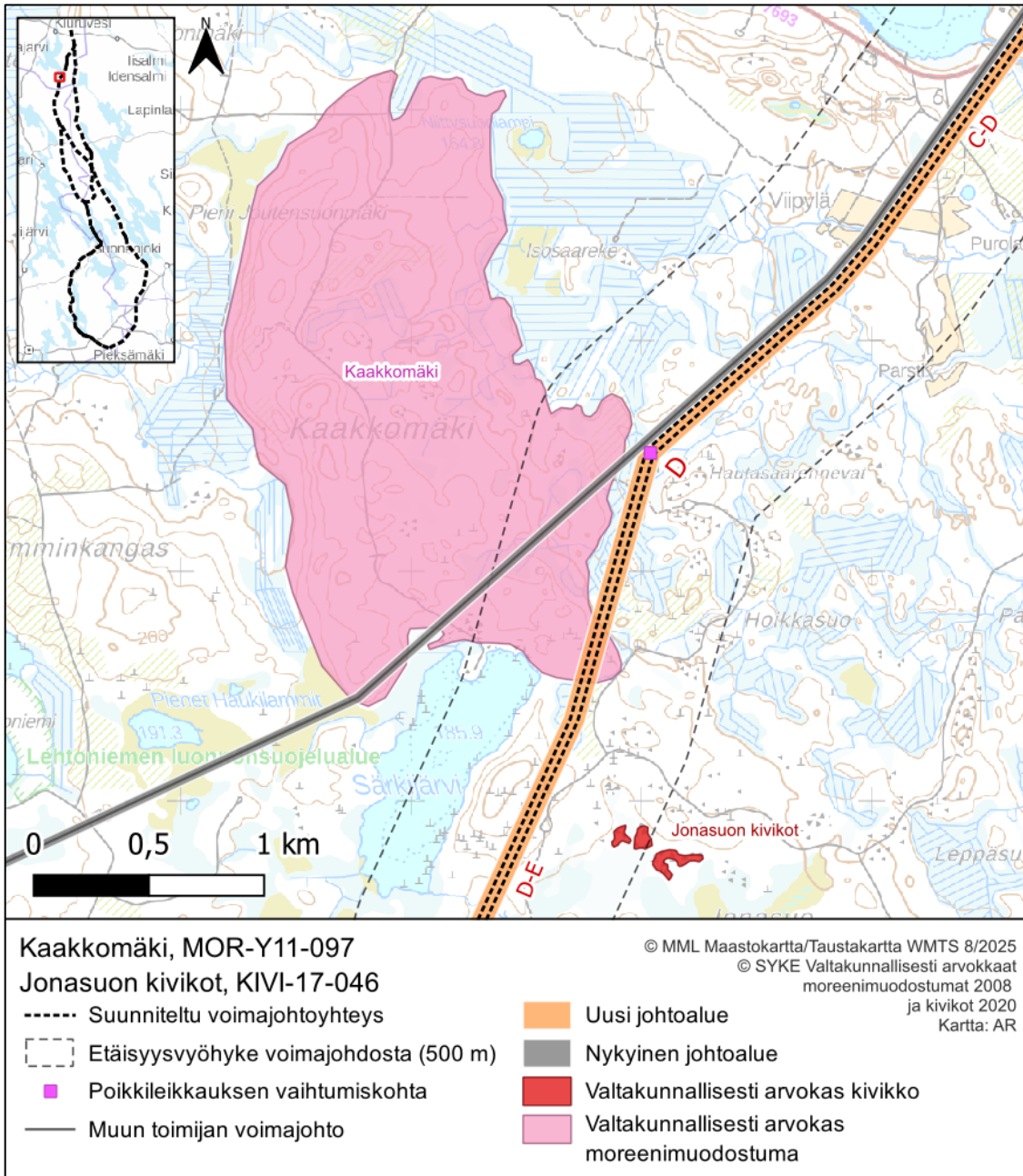
Kuva 5.58. Kaakkomäen arvokas moreenimuodostuma (MOR-Y11-097) sekä arvokas Jonasuon kivikot (KIVI-17-046) voimajohtoyhteyden johto-osuudella Salmelanperä-Kolkku.
