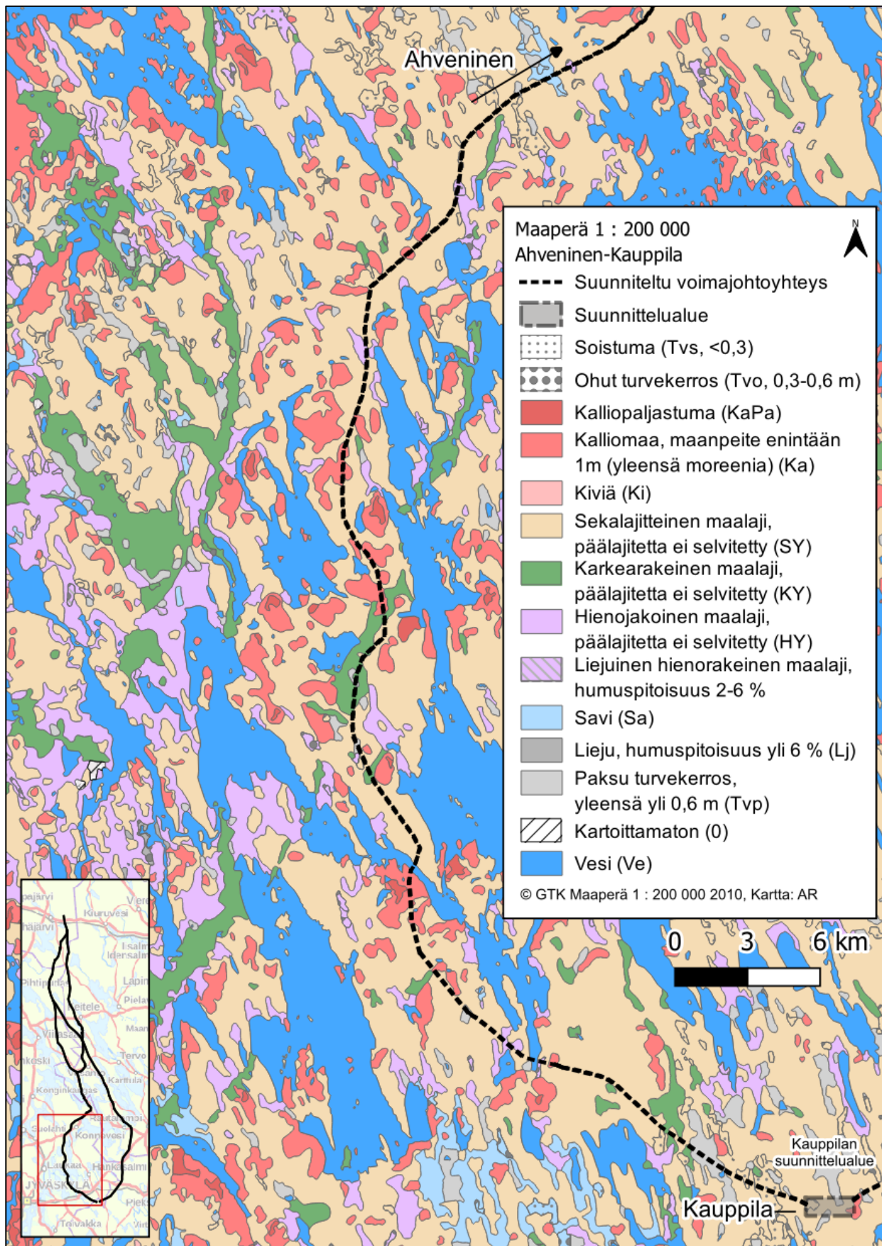
Kuva 5.54. Maaperä suunnitellun voimajohtoyhteyden johto-osuudella Ahveninen-Kauppila.
