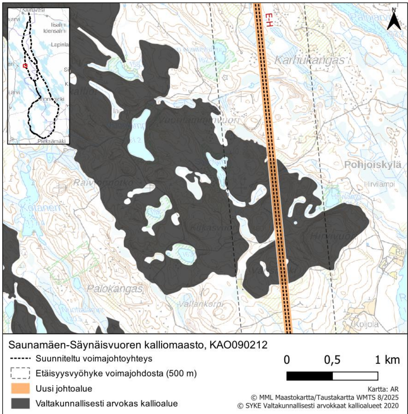
Kuva 5.59 Saunamäen-Säynäisvuoren arvokas kalliomaasto (KAO090212) voimajohtoyhteyden johto-osuudella Kolku-Ahveninen.
