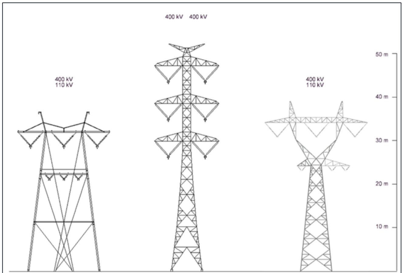
Kuva 3.4. Yhteispylvästyyppejä. Vasemmalla 400+110 kilovoltin harustettu portaalipylvä, keskellä kahden 400 kilovoltin voimajohdon vapaasti seisova T-pylvä ja oikealla 400+110 kilovoltin vapaasti seisova Y-pylvä.
