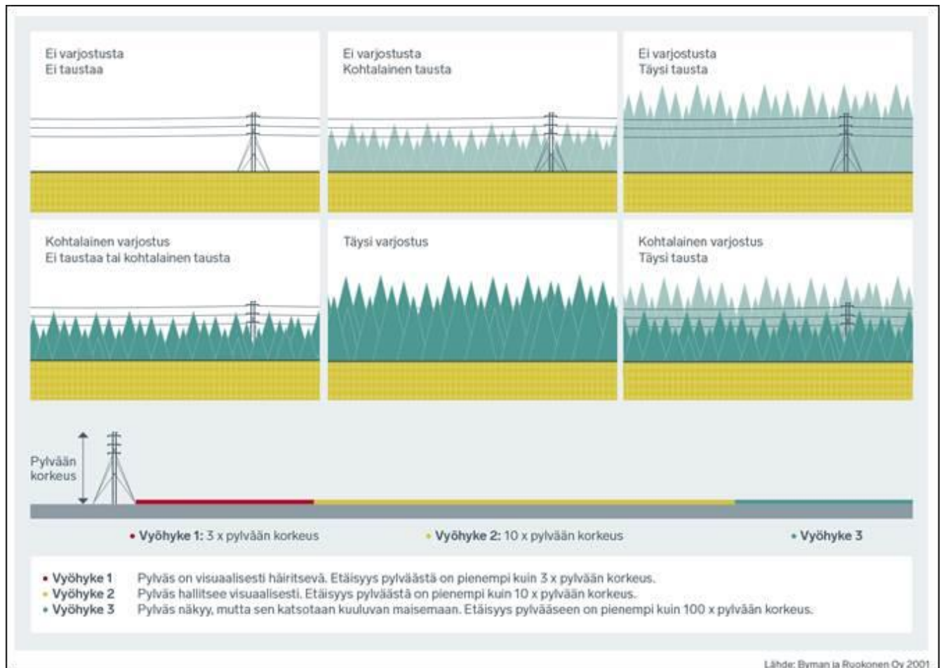
Kuva 5.46 Voimajohdon näkyvyyteen vaikuttavia tekijöitä (Maisema-arkkitehdit Byman ja Ruokonen Oy 2001).
