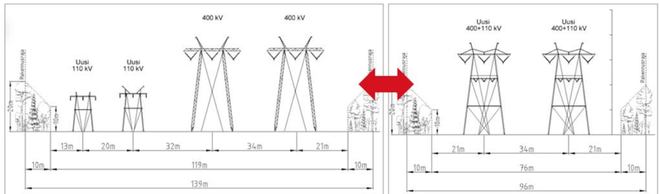
Kuva 3.3. Harjulinjan hankkeessa käytettävä 400+110 kilovoltin yhteispylväsratkaisu mahdollistaa voimajohtojen toteutusta samaan maastokäytävään sijoittamalla 110 kilovoltin voimajohdot yhteispylväiden ala-orteen.
