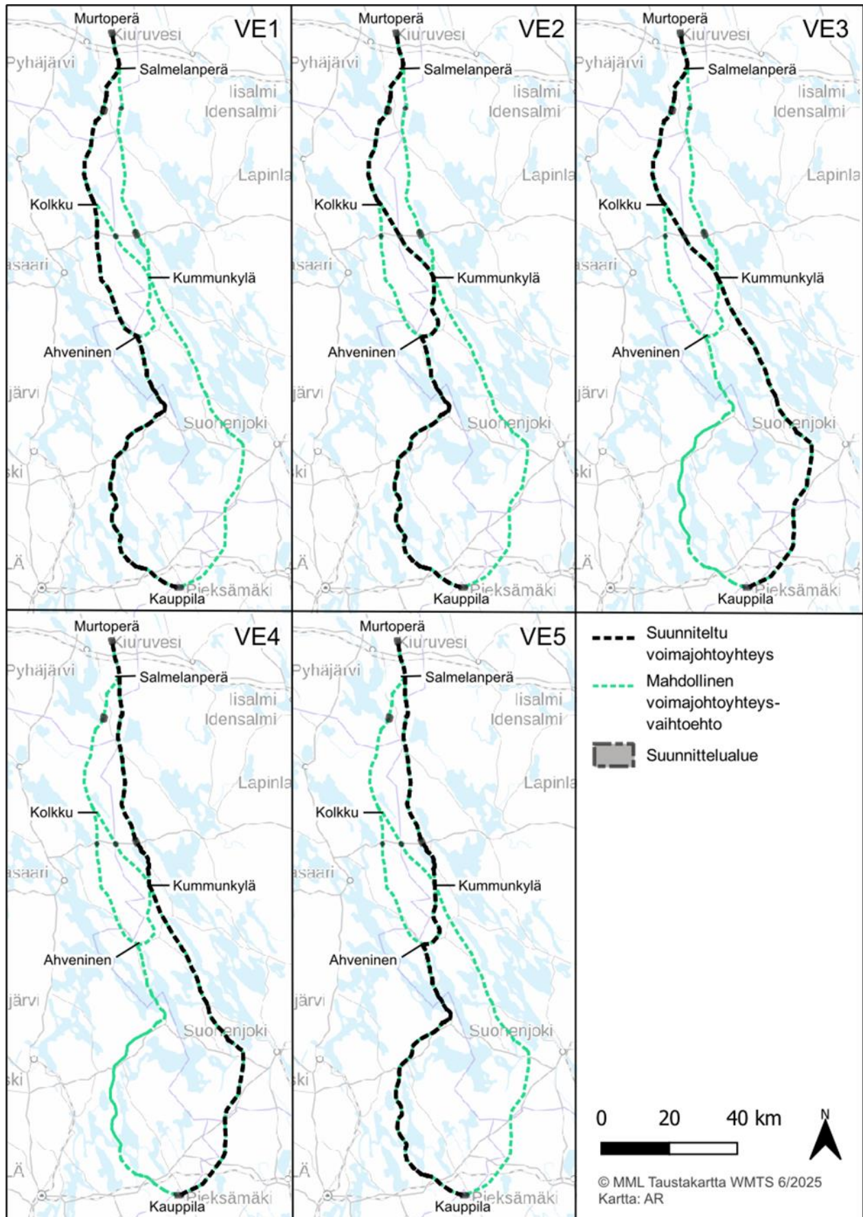
Kuva 1.2. Suunnitellut voimajohtoyhteysvaihtoehdot Murtoperän ja Kauppilan välillä.
