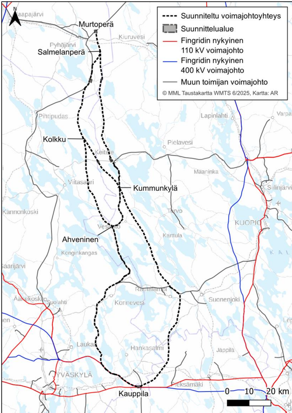
Kuva 1.1. YVA-menettelyssä tarkasteltavat voimajohtoreitit.
