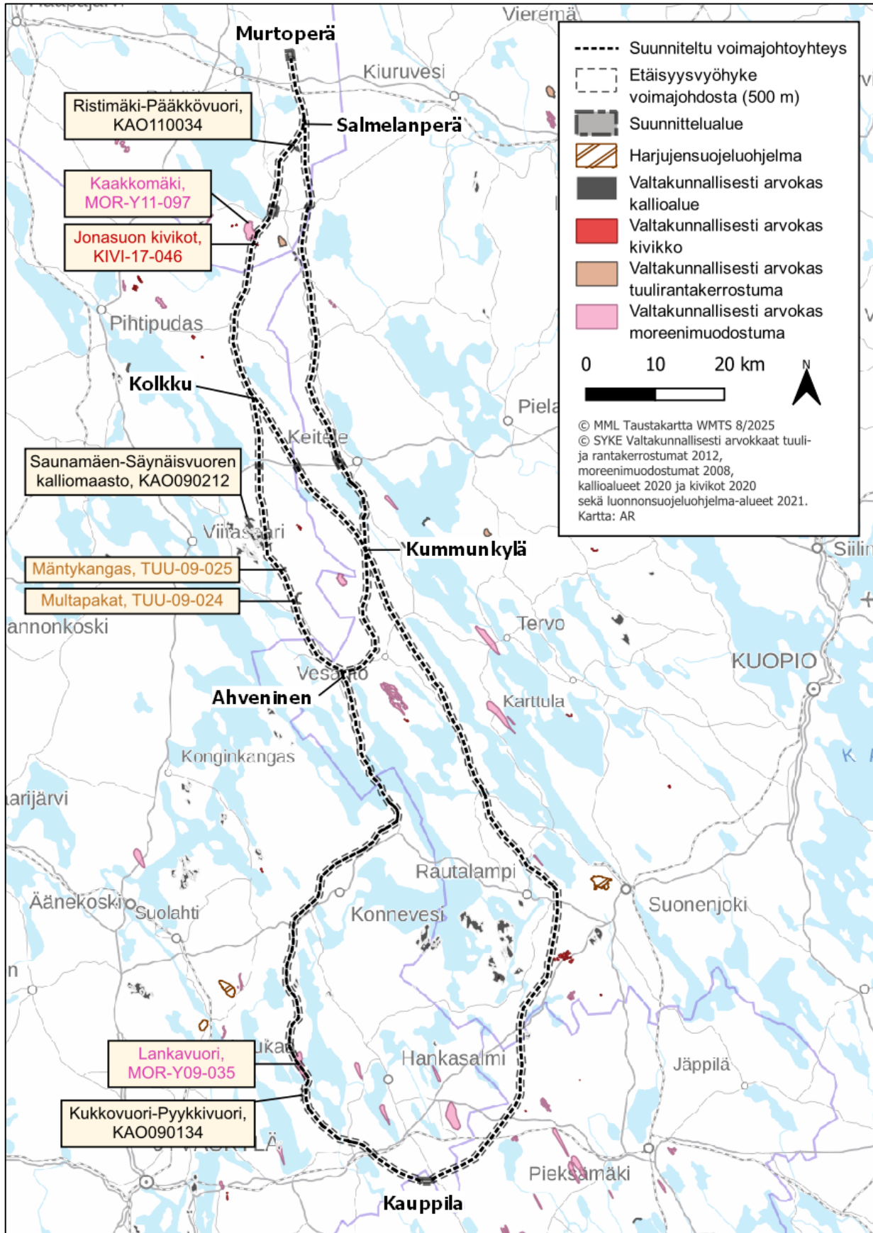
Kuva 5.56. Geologisesti arvokkaat kohteet suunnitellulla voimajohtoyhteydellä ja sen läheisyydessä.
