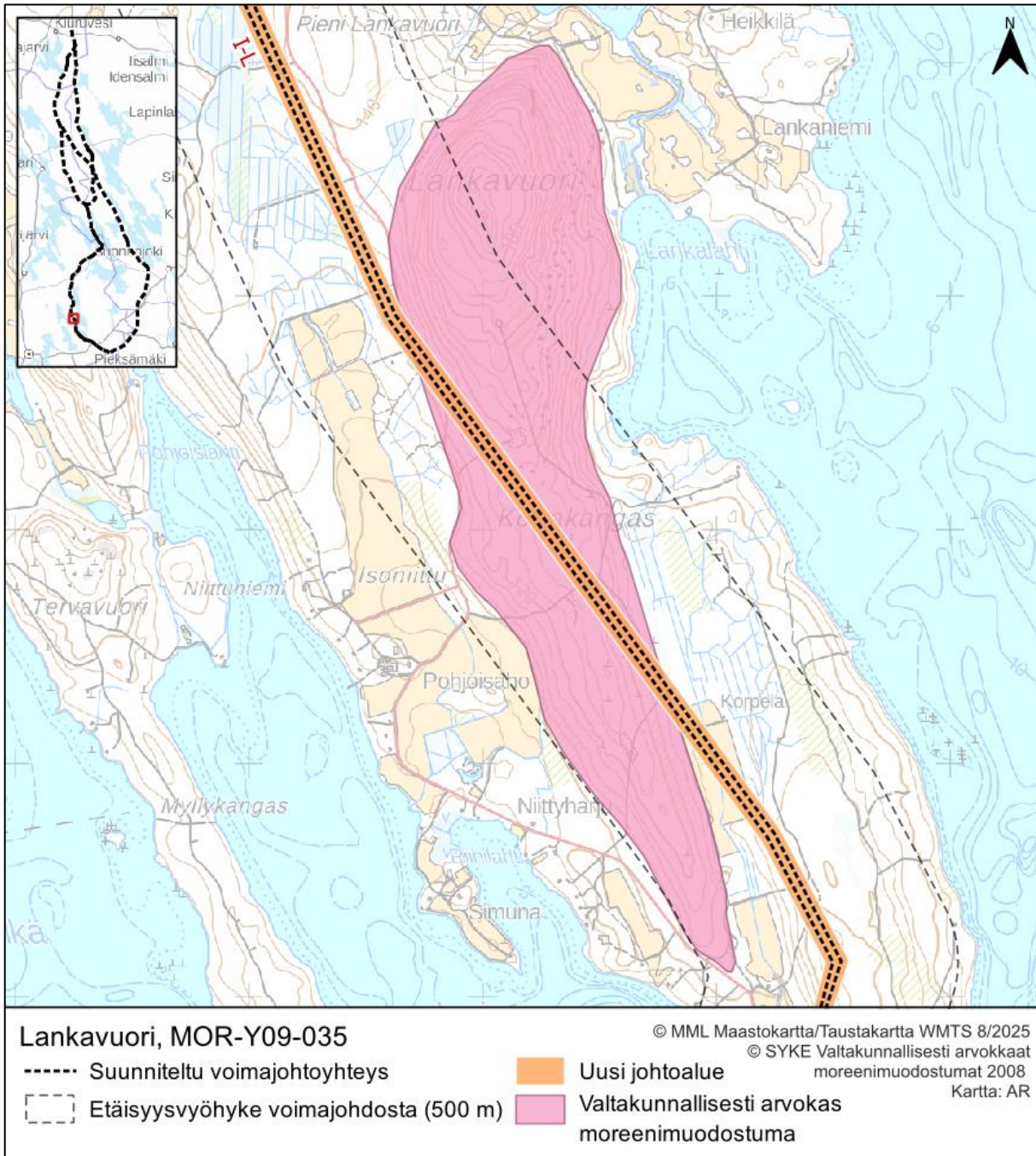
Kuva 5.62 Lankavuoren arvokas moreenimuodostuma (MOR-Y09-035) voimajohtoyhteyden johto-osuudella Ahveninen-Kauppi.
