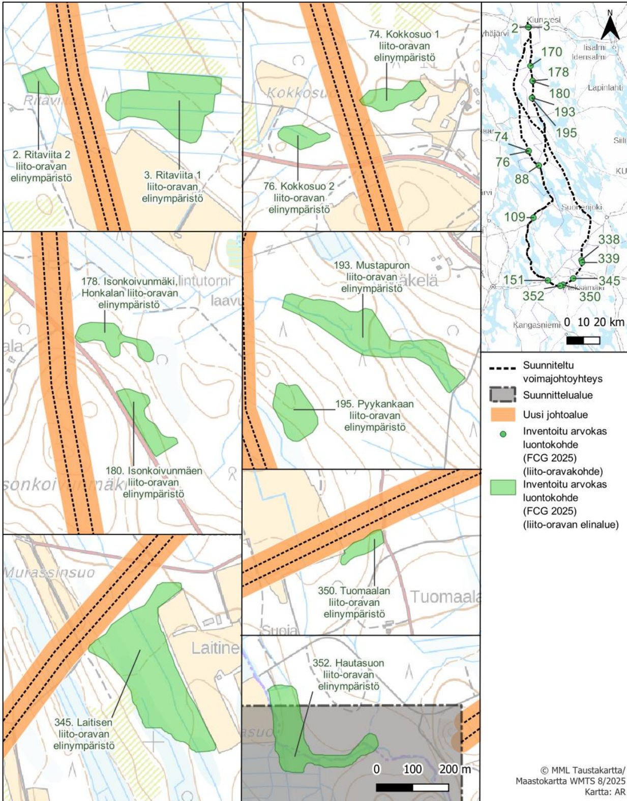
Kuva 5.86 Voimajohtoreittien uudelle voimajohtoalueelle ja sen välittömään läheisyyteen sijoittuvat liito-oravan elinympäristöt.
