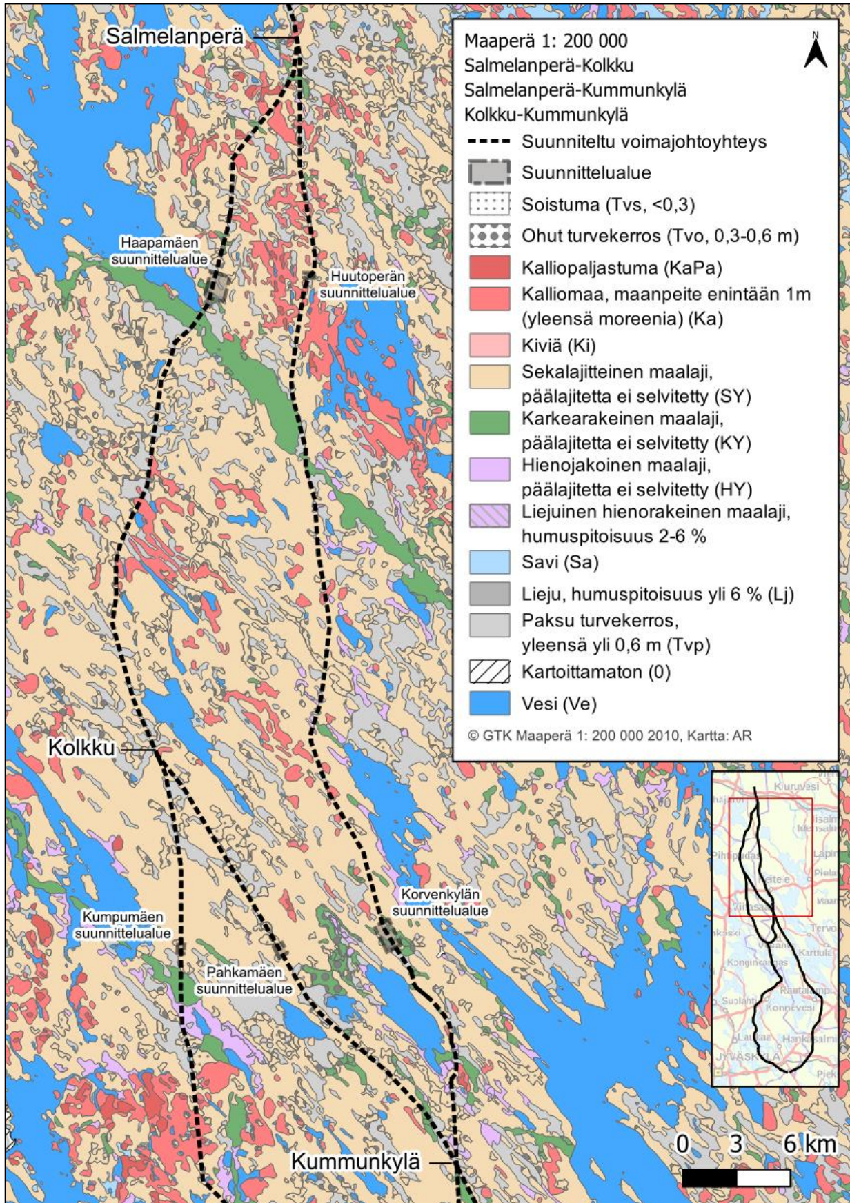
Kuva 5.51. Maaperä suunnitellun voimajohtoyhteyden johto-osuuksilla Salmelanperä-Kolkku, Salmelanperä-Kummunkylä ja Kolkku-Kummunkylä.
