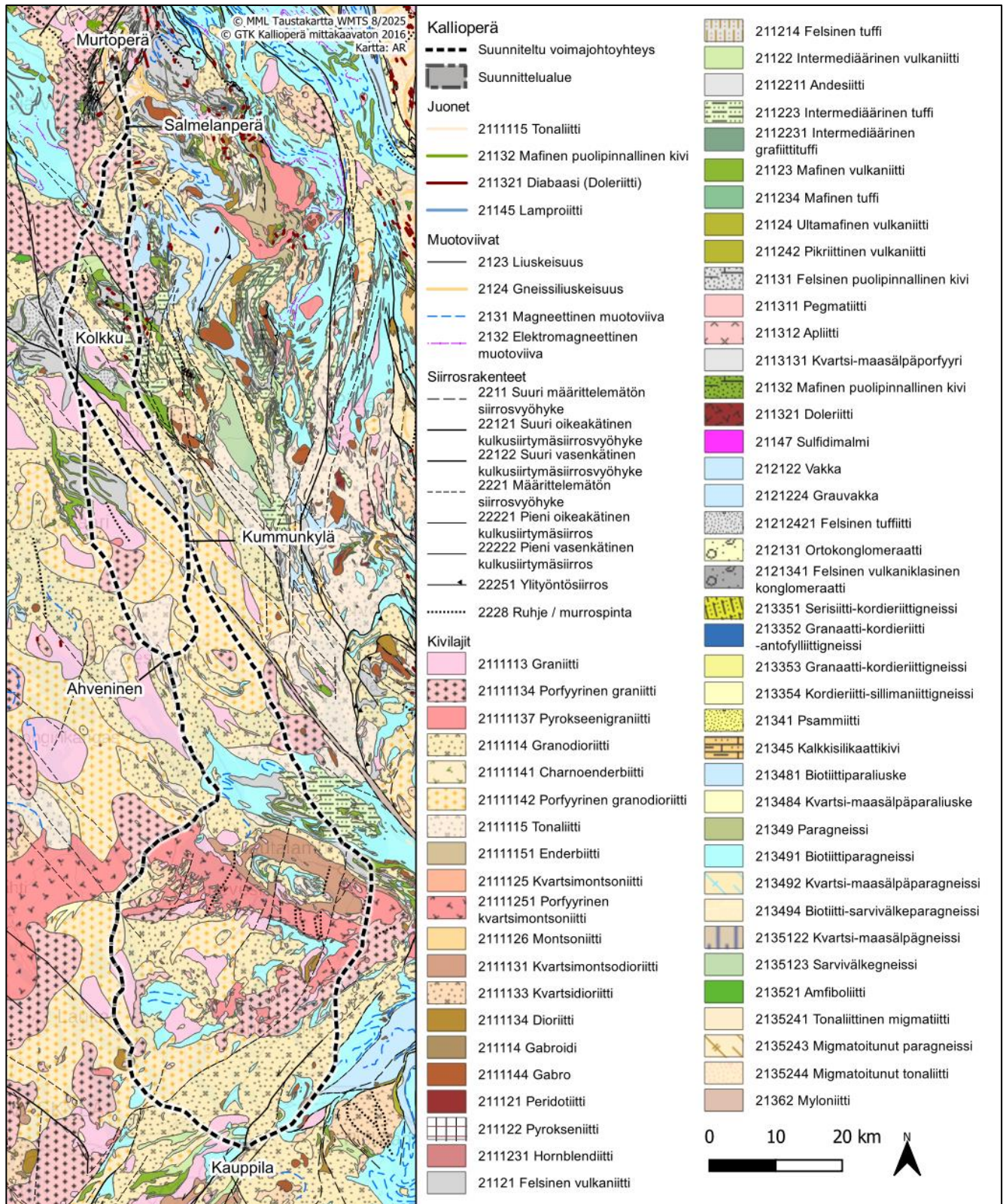
Kuva 5.49 Kallioperä suunnitelluilla voimajohtoreiteillä.
