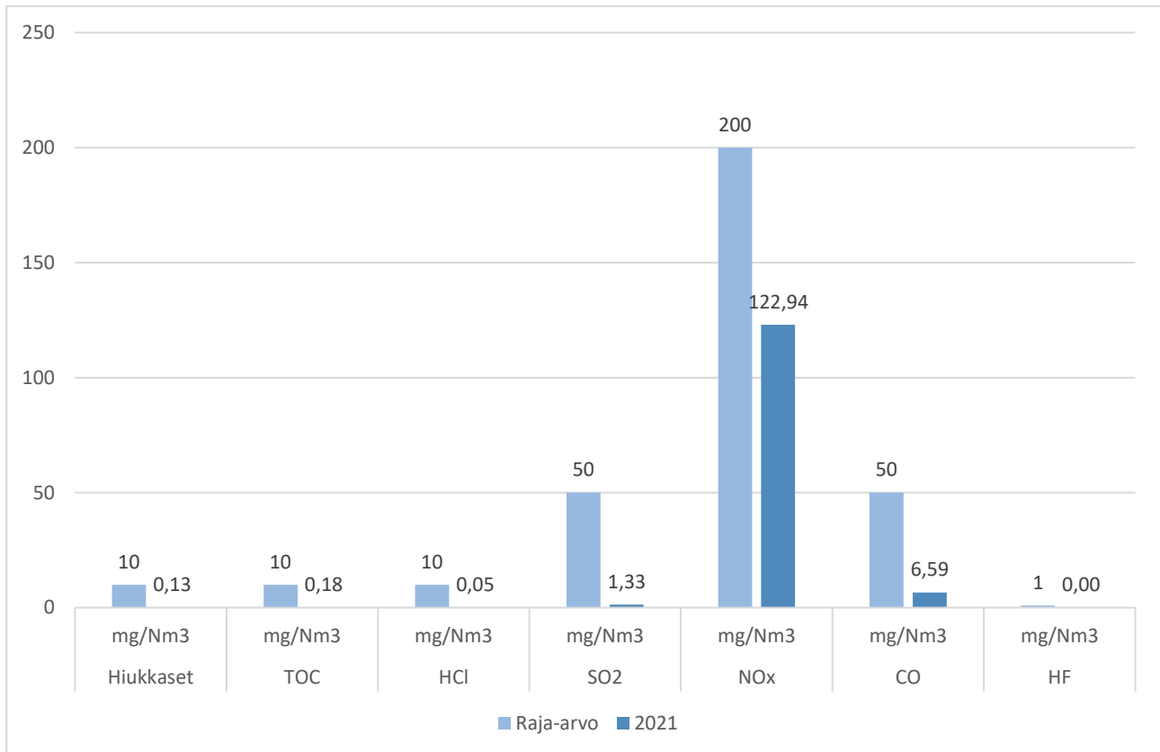
Kuva 3. Epäpuhtauksien keskimääräiset pitoisuudet savukaasussa vuonna 2021 verrattuna ympäristöluvan raja-arvoihin (mg/Nm 3 ).
