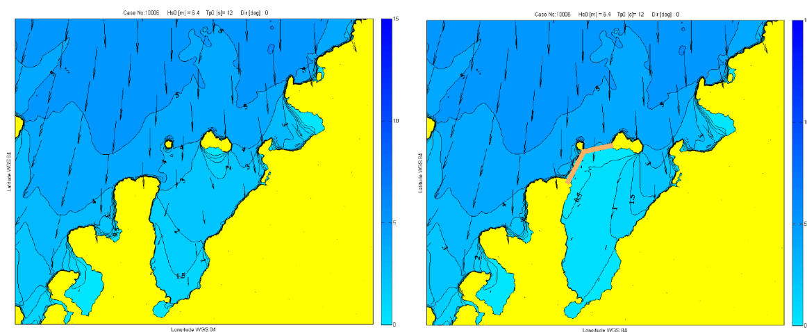
Figur 10. Analyse av 1-års signifikant bølgehøyde for innkommende havsjø ved Mehamn for bølger fra 0 ° (nord). Kart til t.v. viser dagens situasjon, mens t.h. vises situasjon med molo fra Vevikneset til Lille Kamøya. Kilde: Polytec 2014 (Report no.11792-R001)
