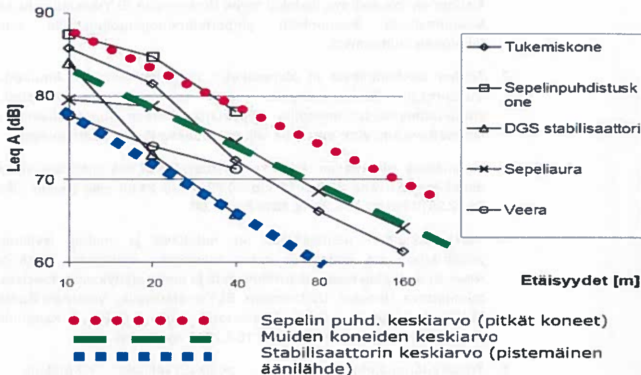
Kuva 1. Ratatyökoneiden aiheuttamat melupäästöt etäisyyden funktiona.
