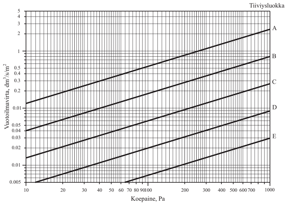
Kuva 3. Ilmanvaihtojärjestelmän ja sen osien suurimmat sallitut vuotoilmavirrat vaipan pinta-alaa kohti eri tiiviysluokissa.
