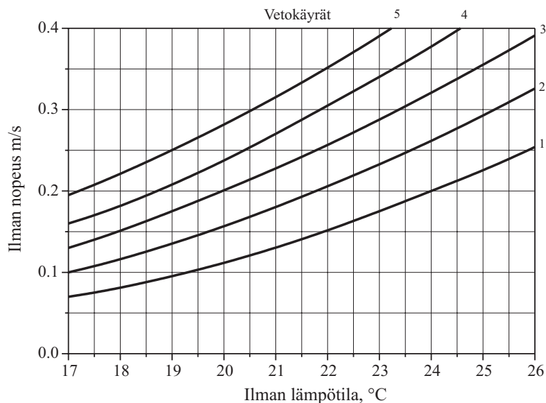
Kuva 1. Vetokäyrät kuvaavat epäviihtyisyyttä aiheuttavan ilman liikkeen riippuvuutta ilman lämpötilästä.
