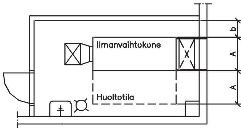
Kuva 4. Koteloidun ilmanvaihtokoneen huoltotilan sijoitus ja mitoitus esimerkki. A on ilmanvaihtokoneen leveys ja b on 0,4 kertaa ilmanvaihtokoneen korkeus tai vähintään 400 mm.
