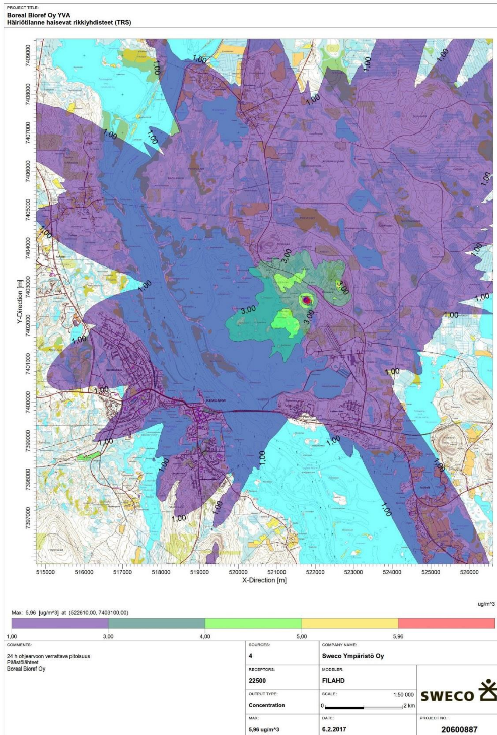
Kuva 4.4-17. Rikkiyhdisteiden (TRS) korkein vrk-ohjearvoon verrannollinen pitoisuus häiriötilanteessa H1.
