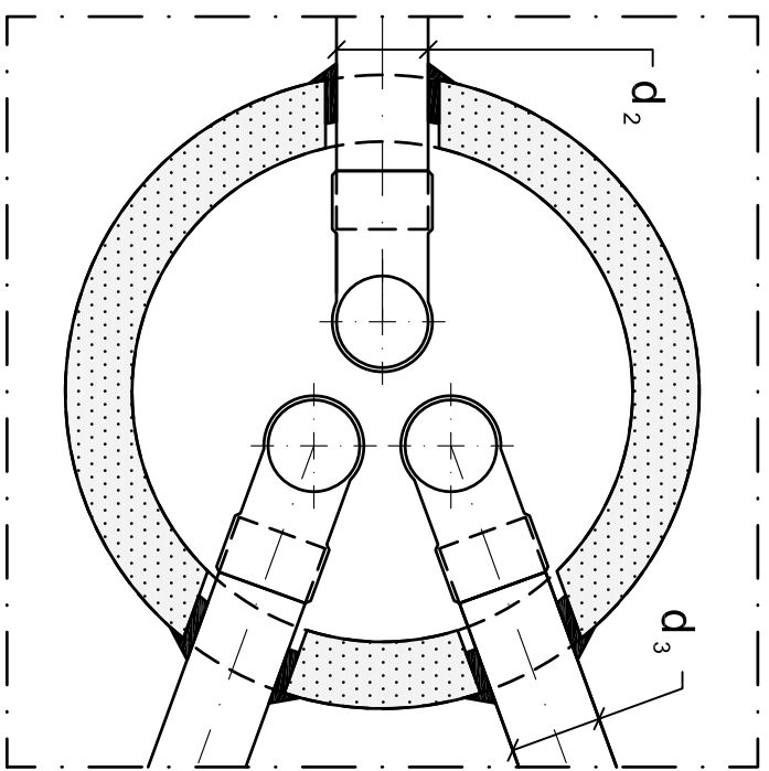
LEIKKAUS A - A
