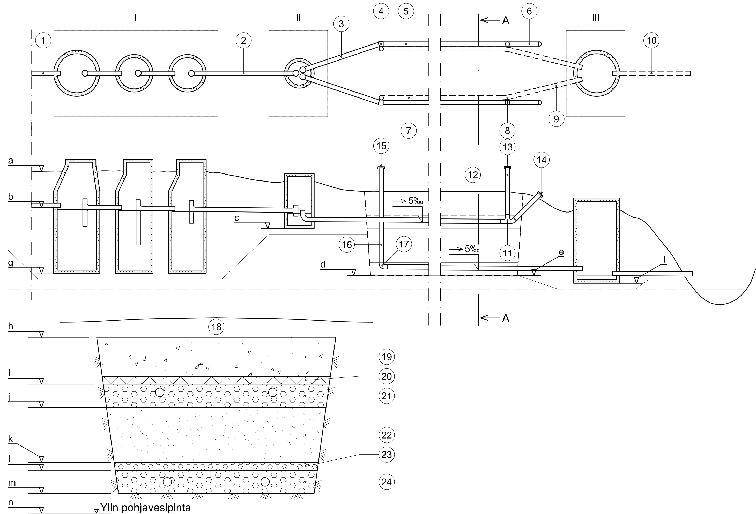
Leikkaus A - A (1:25)
