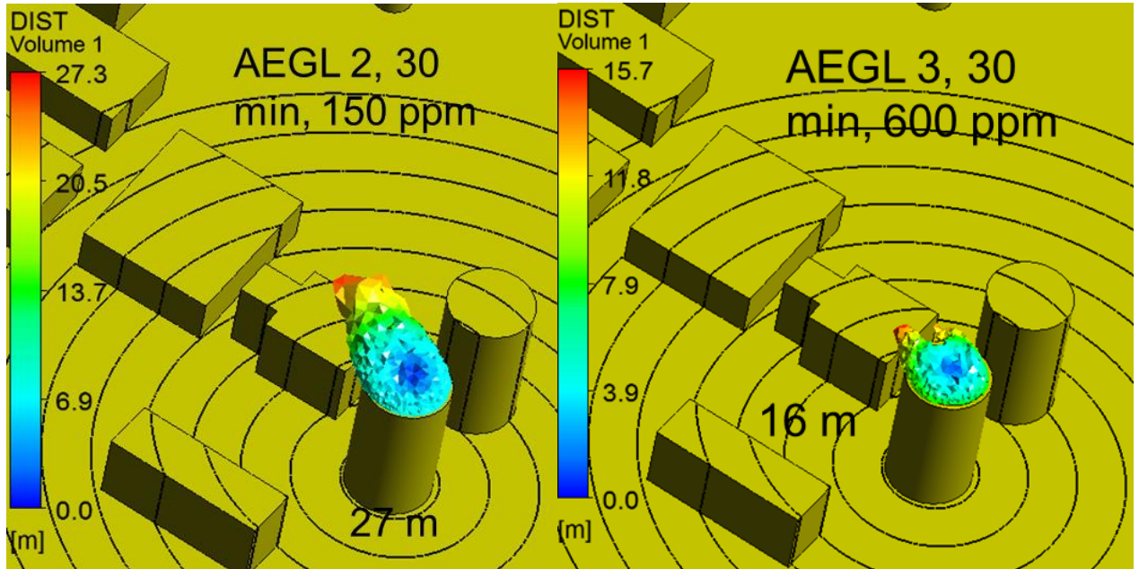
Kuva 20. Hiilimonoksidin leviämialueet hakepalossa tuulen nopeudella 10 m/s, joilla AEGL-2 (30 min) ja AEGL-3 (30 min) pitoisuudet ylittyvät.
