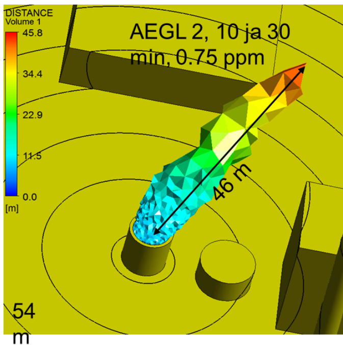
Kuva 17. Rikkidioksidin leviämialue POK-säiliön palossa tuulen nopeudella 5 m/s, joilla AEGL-2 (10 ja 30 min) ja AEGL-3 (10 ja 30 min) pitoisuudet ylittyvät.
