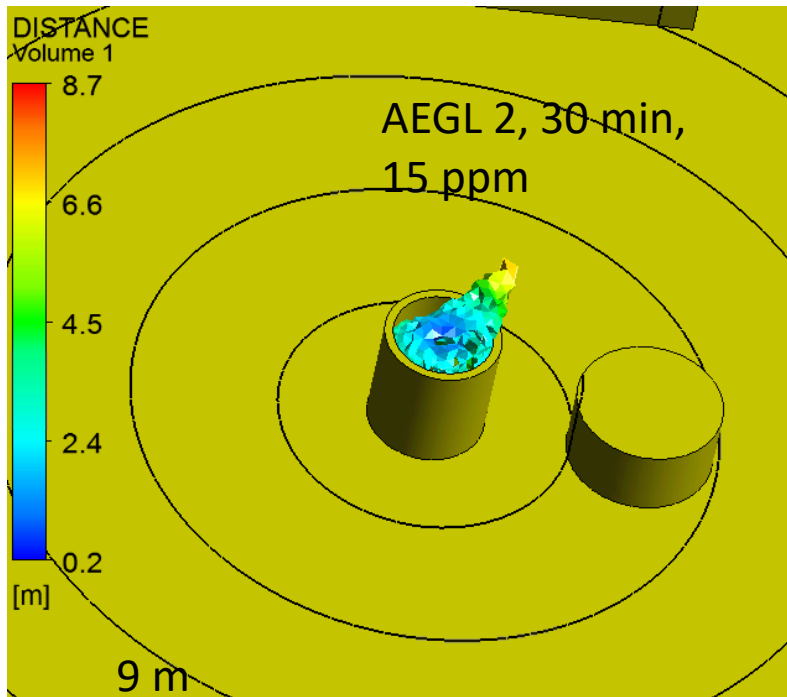
Kuva 16. Typpidioksidin leviämialueet POK-säiliön palossa tuulen nopeudella 10 m/s, jolla AEGL-2 (30 min) pitoisuudet ylittyvät. AEGL-2 (10 min) ja AEGL-3 -rajat eivät ylity.
