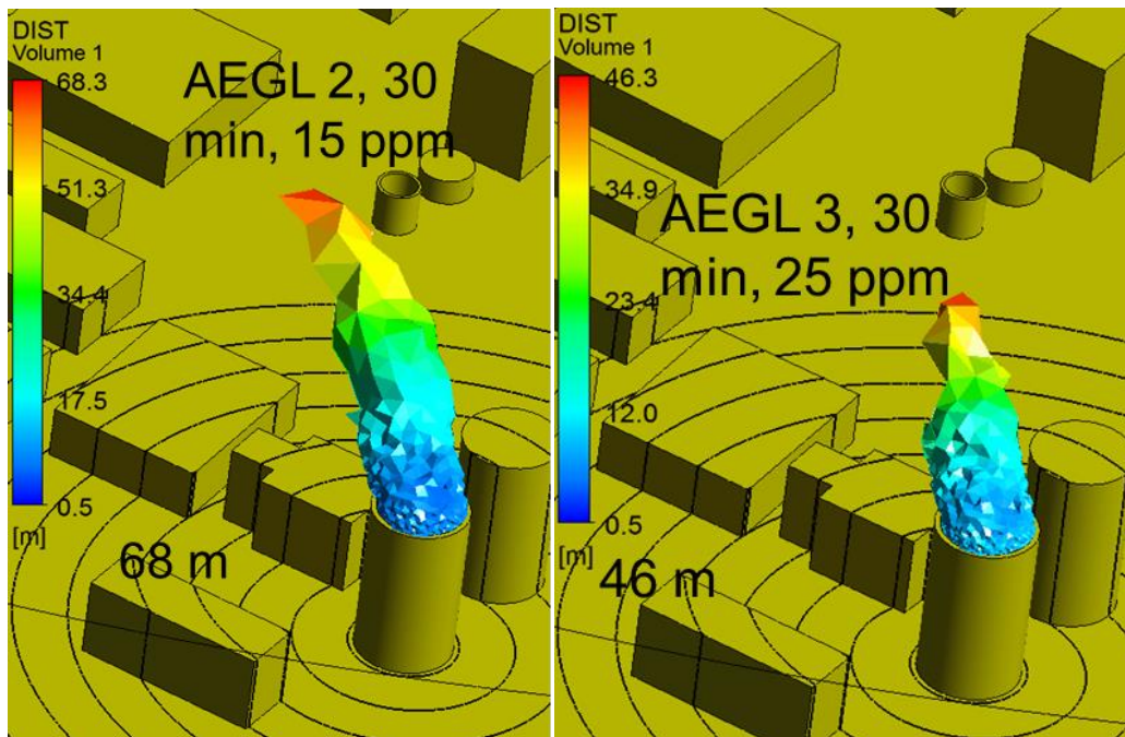
Kuva 23. Typpidioksidin leviämialueet hakepalossa tuulen nopeudella 5 m/s, joilla AEGL-2 ja AEGL-3 (30 min) pitoisuudet ylittyvät.
