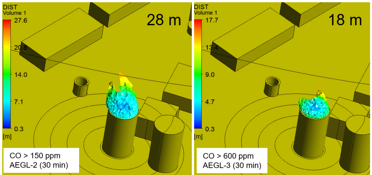
Kuva 26. Hiilimonoksidin leviämisalueet hakepalossa tuulen nopeudella 10 m/s, joilla AEGL-2 (30 min) ja AEGL-3 (30 min) pitoisuudet ylittyvät.
