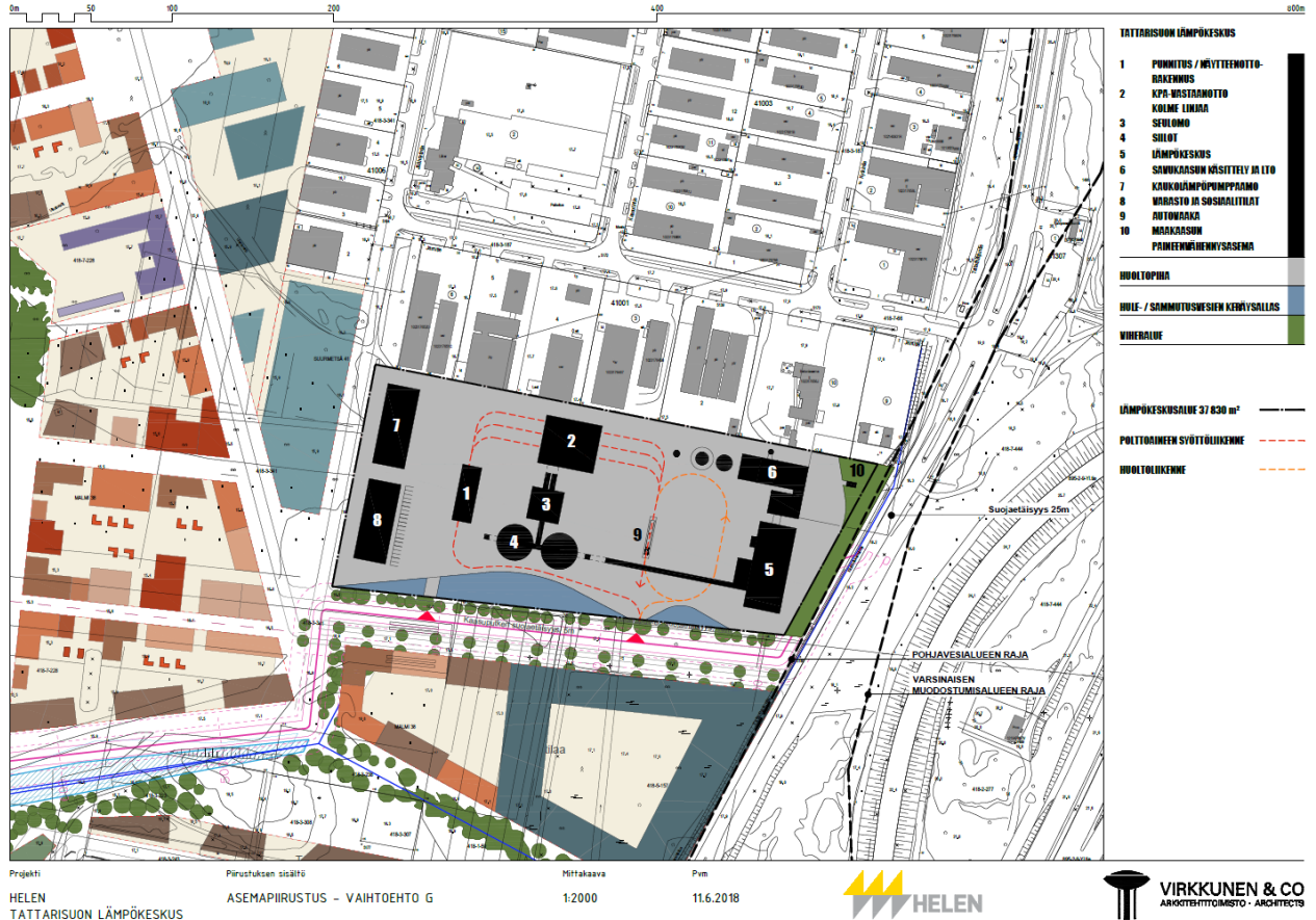
Kuva 3. Tattarisuon biolämpökeskuksen VE2:n suunniteltu layout.
