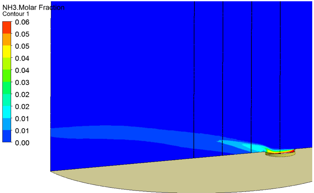
Kuva 39. Ammoniakkiliuossäiliön palo, alle 6 % pitoisuudet, kaikki ammoniakki ei pala.
