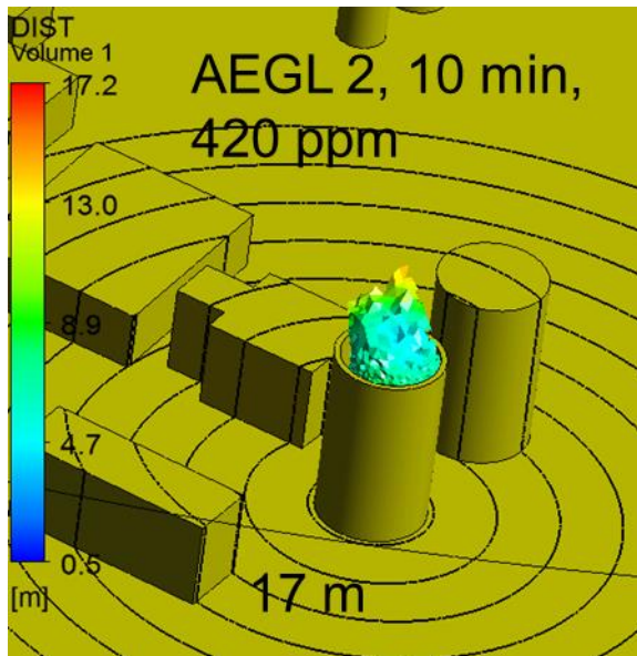
Kuva 21. Hiilimonoksidin leviämialueet hakepalossa tuulen nopeudella 5 m/s, jolla AEGL-2 (10 min) pitoisuudet ylittyvät. AEGL-3 (10 min) 1700 ppm pitoisuudet eivät ylitä.
