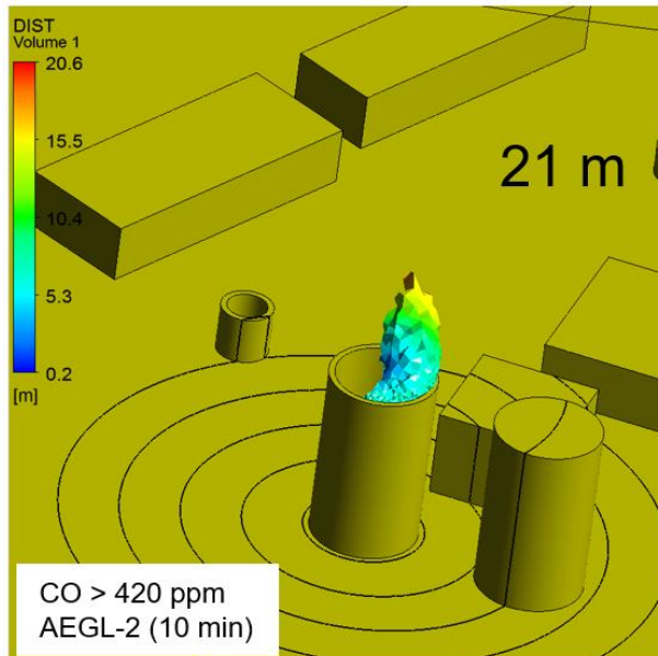
Kuva 27. Hiilimonoksidin leviämisalueet hakepalossa tuulen nopeudella 5 m/s, jolla AEGL-2 (10 min) pitoisuudet ylittyvät. AEGL-3 (10 min) 1700 ppm pitoisuudet eivät ylitä.
