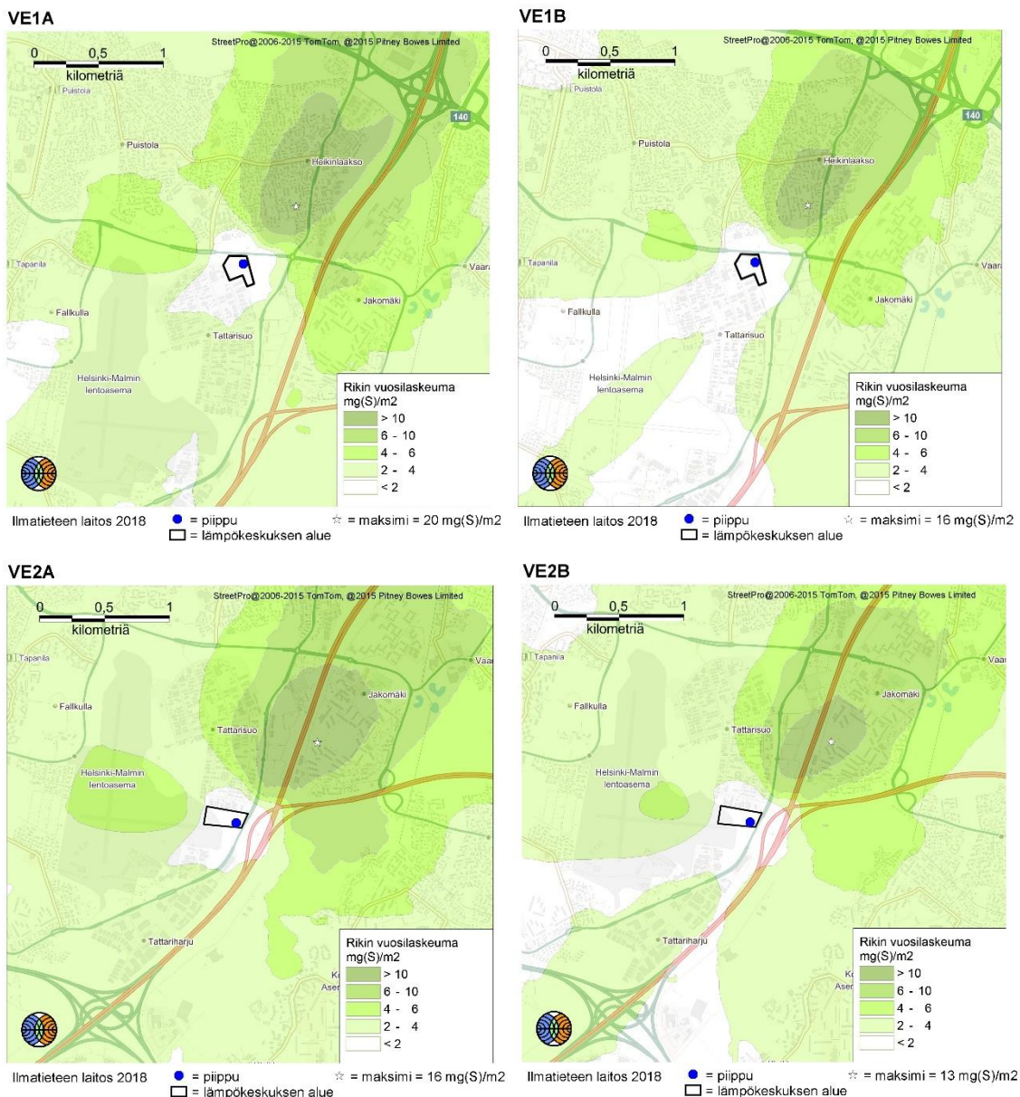
Kuva 13. Leviämismallilaskelmilla saadut Helen Oy:n Tattarisuon rikkidioksidipäästöjen aiheuttamat korkeimmat sulfaattilaskeuman vuosiarvot tutkimusalueella eri tarkasteluvaihtoehdoissa.
