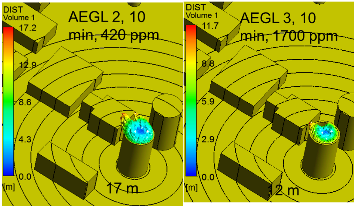
Kuva 22. Hiilimonoksidin leviämialueet hakepalossa tuulen nopeudella 10 m/s, jolla AEGL-2 ja AEGL-3 (10 min) pitoisuudet ylittyvät.
