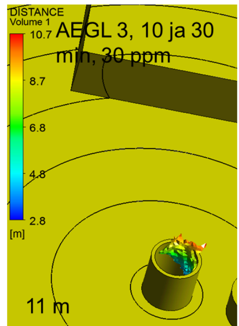
Kuva 17. Rikkidioksidin leviämialue POK-säiliön palossa tuulen nopeudella 5 m/s, joilla AEGL-2 (10 ja 30 min) ja AEGL-3 (10 ja 30 min) pitoisuudet ylittyvät.
