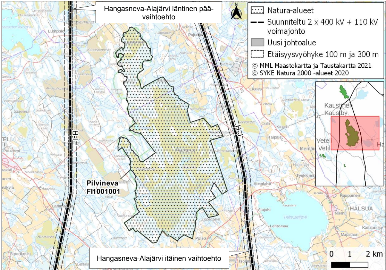
Kuva 6.1. Suunniteltujen voimajohtoreittivaihtoehdojen sijoittuminen suhteessa Pilvinevan Natura-alueeseen.
