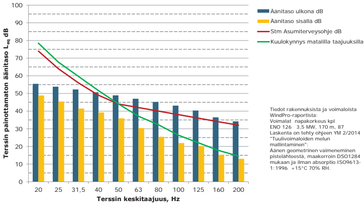
Matalien taajuuksien äänitasot ulkona ja sisällä, Z Lomarakennus (Haukilampi), ääneneristävyyttä DSO1284 mukaan
