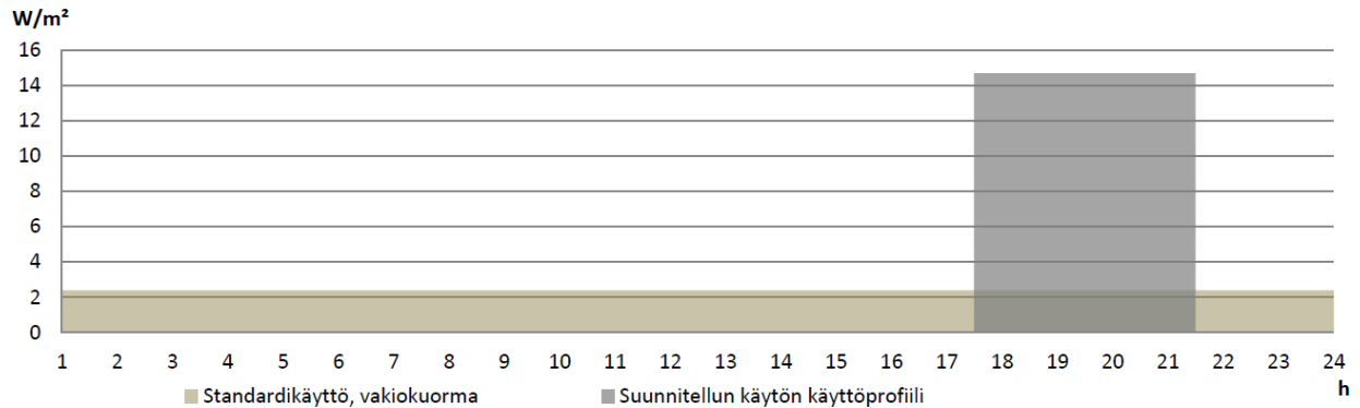
Kuva 3. Esimerkki asuinkeittiön olohuoneen kuluttajalaitteiden standardikäytön ( 4,0 \text{ W/m}^2 \times 0,6 = 2,4 \text{ W/m}^2 , ma-su 24 h) ja suunnitellun käytön ( 250 \text{ W} kulutuselektronikka / 17,0 \text{ m}^2 = 14,7 \text{ W/m}^2 , ma-su 18-22) lämpökuorman käyttöprofiilista.
